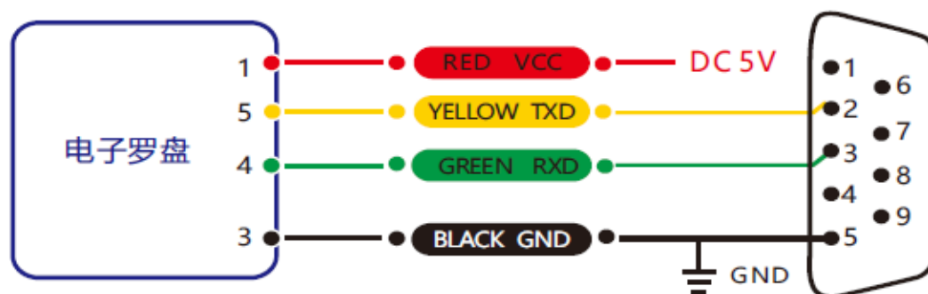
RS 232接线图
