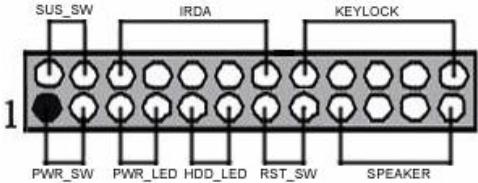
面板插针接口
