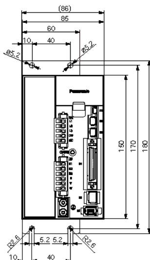
托架固定型 (可选零部件: 正面安装)
