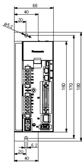
托架固定型 (可选零部件: 正面安装)
