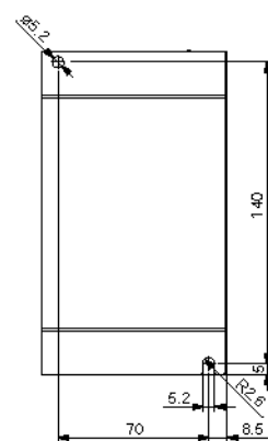
基础固定型 (标准: 在背面安装)
