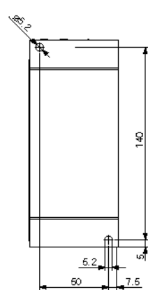
基础固定型 (标准: 在背面安装)
