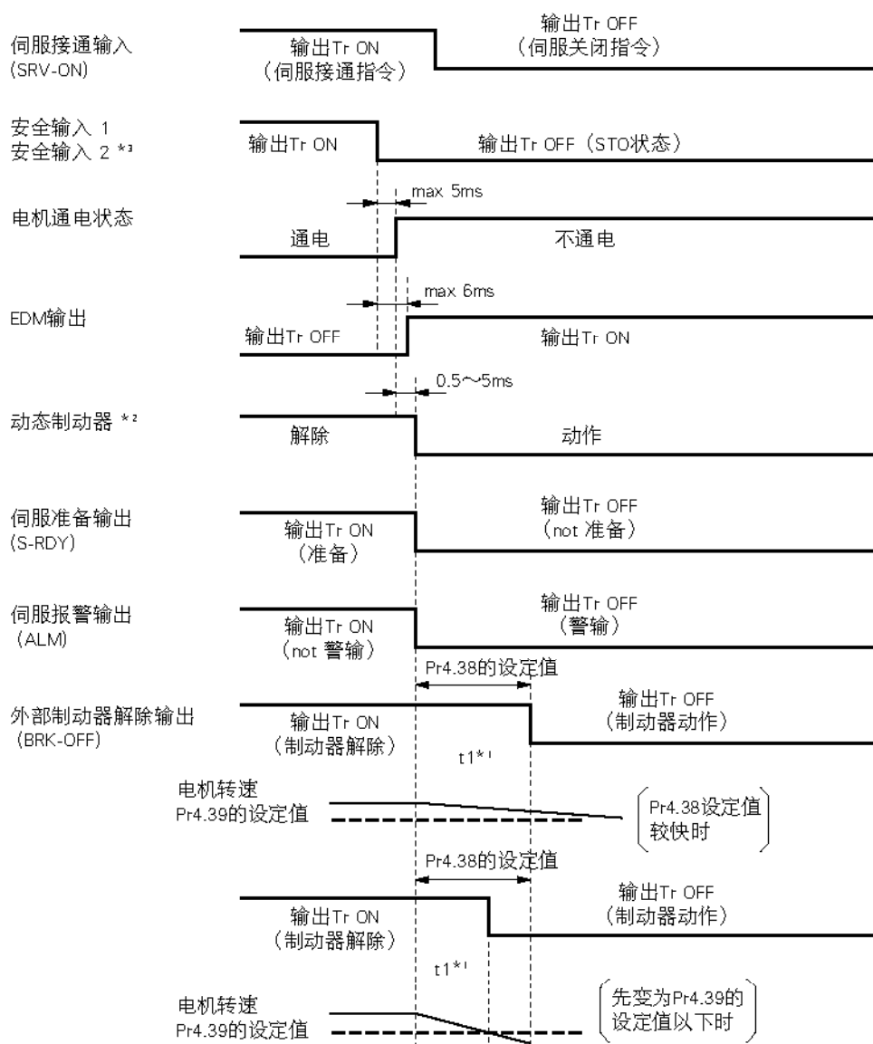
进入安全状态的工作时间图
