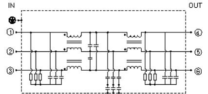
电路图
