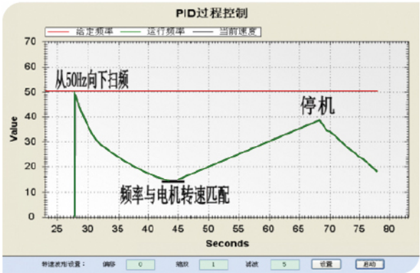
飞车启动扫频曲线
