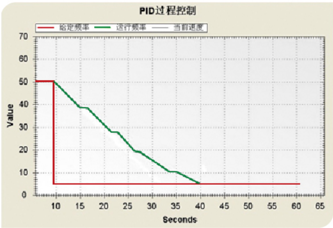
正常减速曲线
