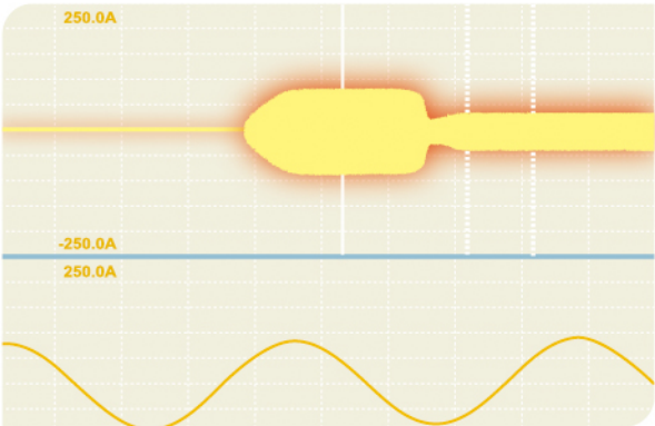
飞车启动电流曲线
