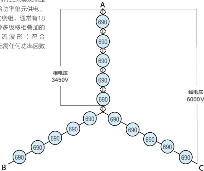
6kV产品 5个功率单元叠加图
