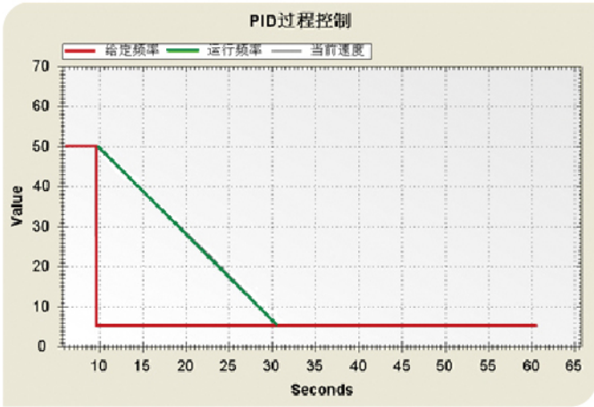
自均衡技术减速曲线
