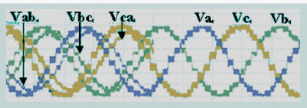
单元A3被旁路后输出电压波形
