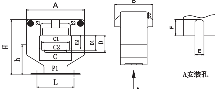
图3 LMZ3(D)-0.66 (400~600) A
