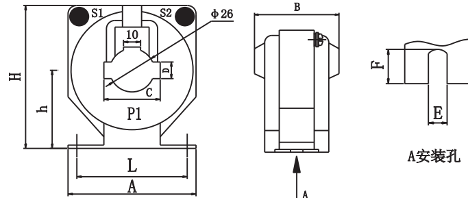
图2 LMZ3(D)-0.66 (150~300) A
