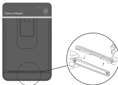
图30 清洁集水盘
