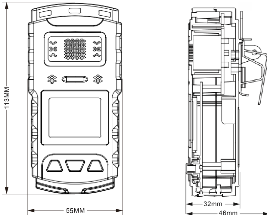
CTH1000 一氧化碳测定器外形尺寸
