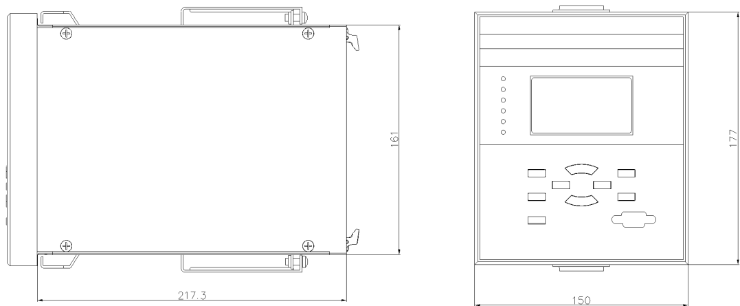
图 3-1 外形尺寸
