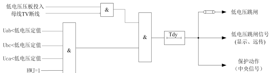
图中 Tdy 为低电压延时
