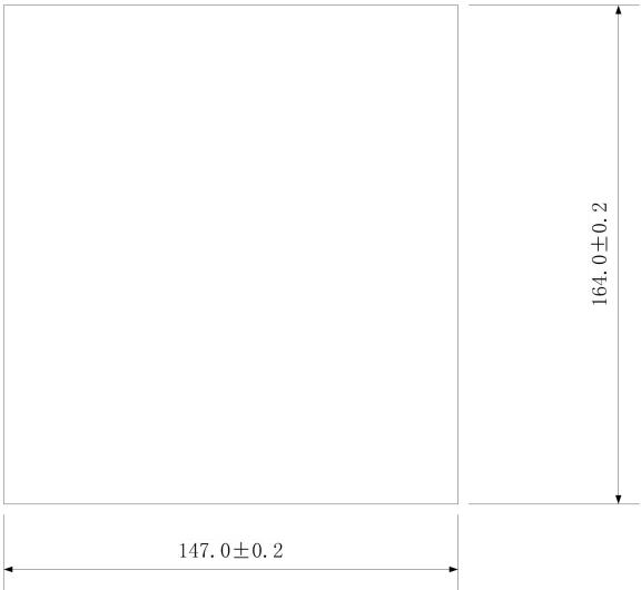
图 3-2 安装开孔尺寸
