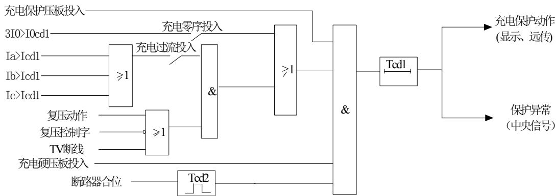
Tcd1: 充电动作时间 Tcd2: 充电投入时间
