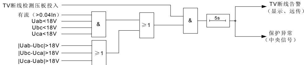
图 4-11 TV 断线检测原理框图
