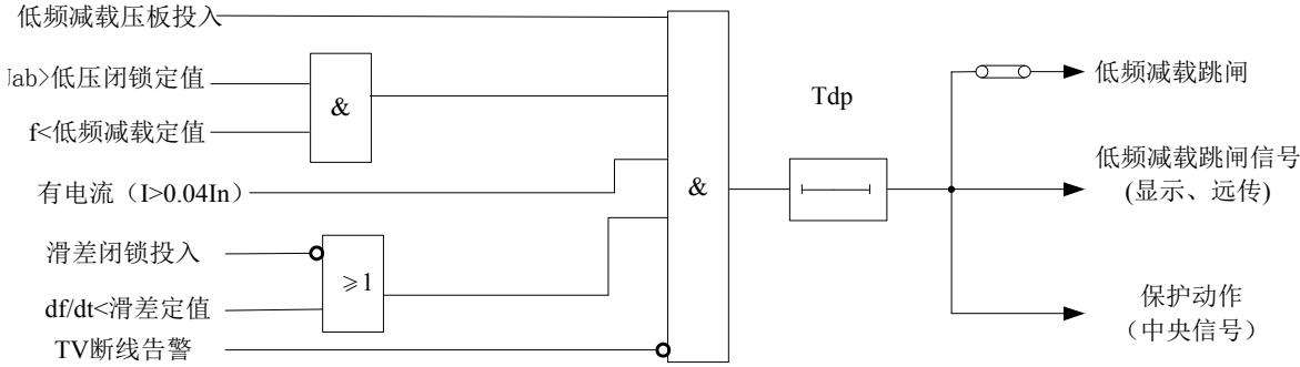
图中Tdp为低频减载延时
