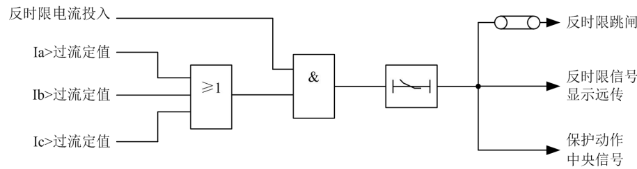
图 4-3 过流反时限逻辑框图
