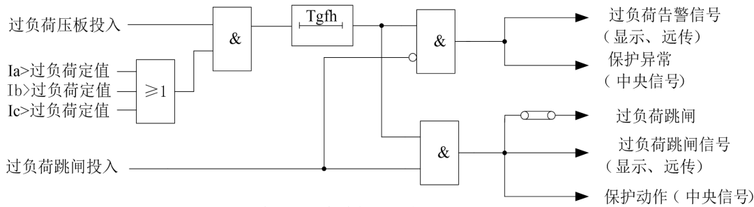
图中 Tgfh 为过负荷延时
