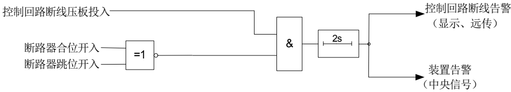
图 4-12 控制回路异常告警原理框图
