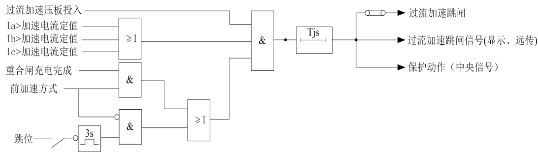
图中Tjs为过流加速延时
