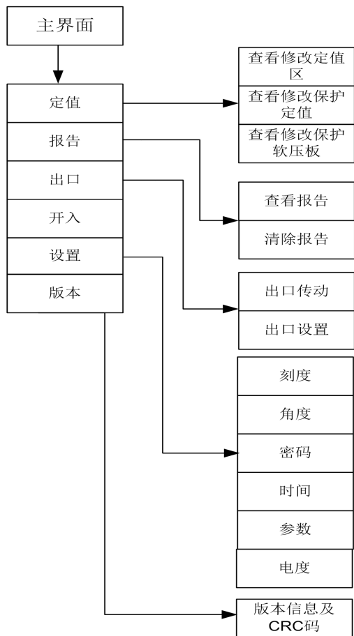
图 6-1 主菜单目录结构图
