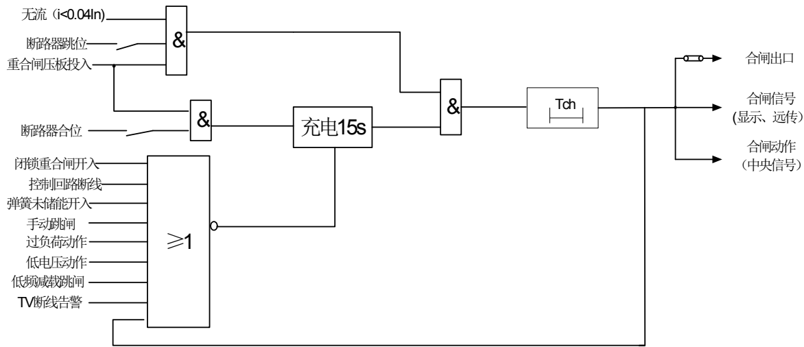
图 4-7 三相一次重合闸原理框图
