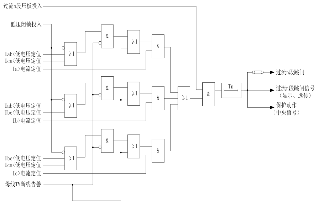
图中Tn为电流n段延时 (n=I、II、III)
