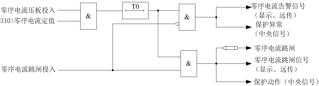
图中T0为零序电流延时
