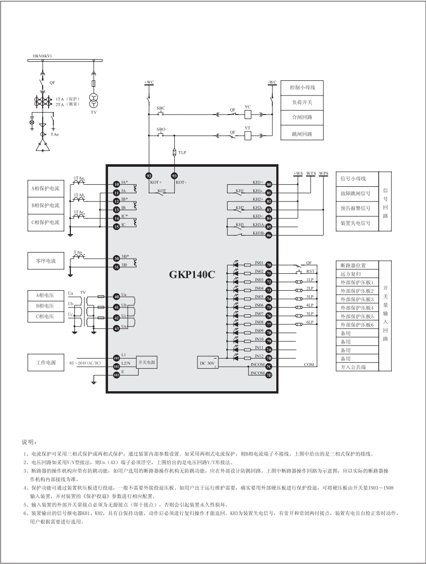
GKP140C高压电容器保护装置接线原理图
