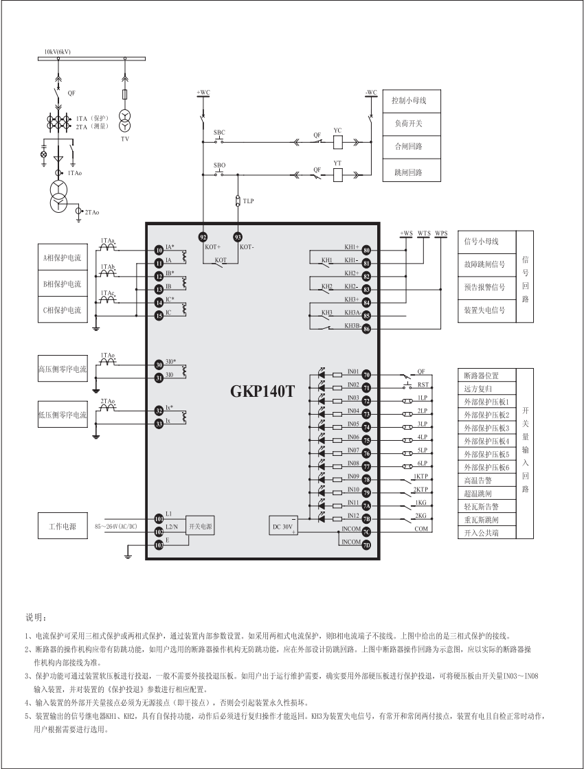
140T厂用变压器保护装置原理图
