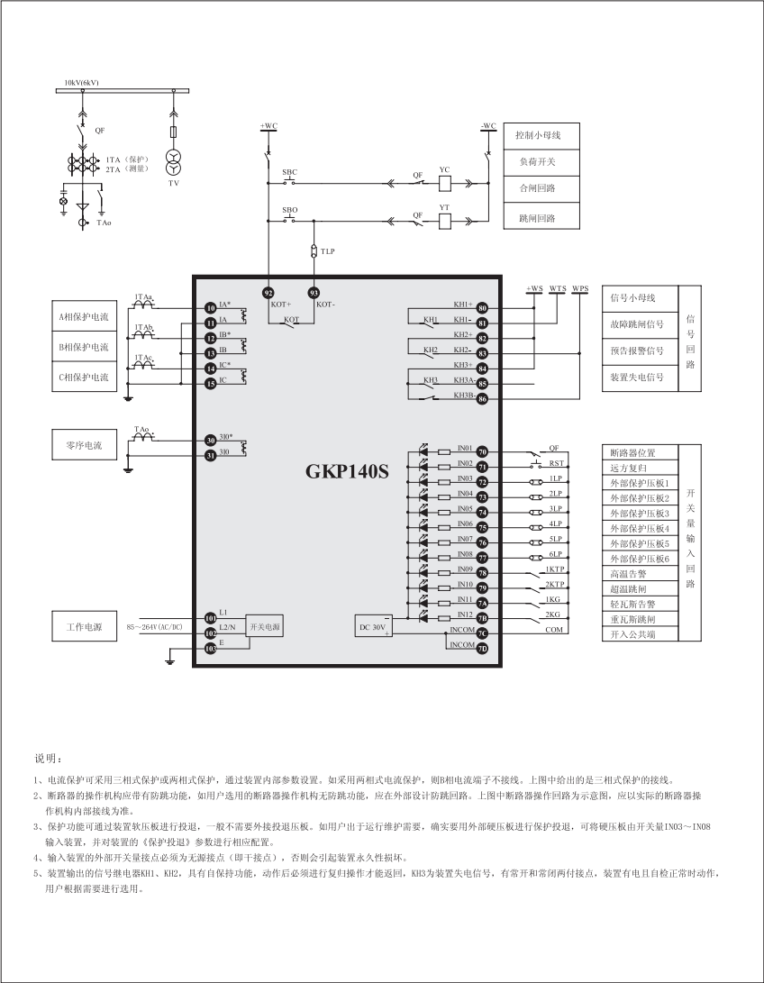
GKP140S组合式电流保护装置接线原理图
