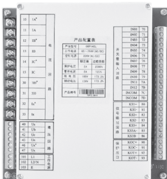
图 2.2 GKP140 后面板接线端子图
