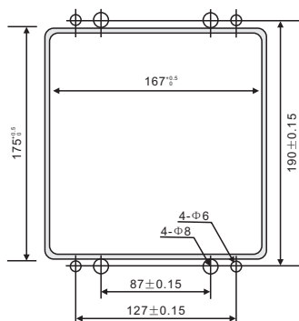
安装开孔图
