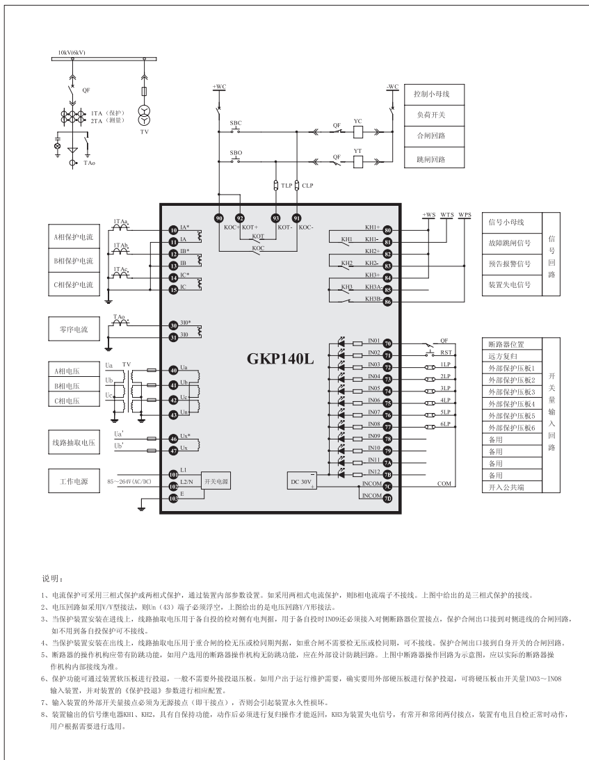
GKP140L线路保护装置原理图
