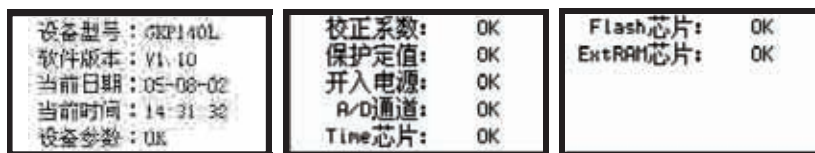
图 3.3.5 系统自检信息显示画面
