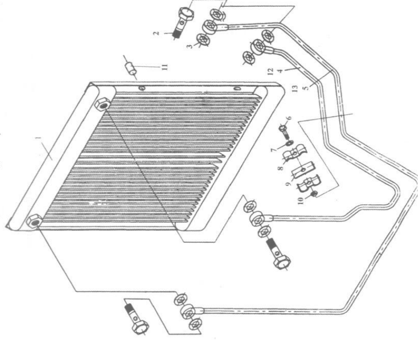
4. 机油散热器 (用于 8041、8002) Oil Radiator (for 8041, 8002)
