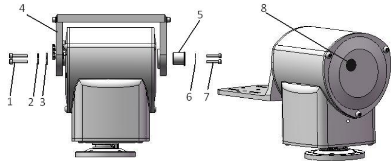
图 11 用侧装部件来替换顶装部件
