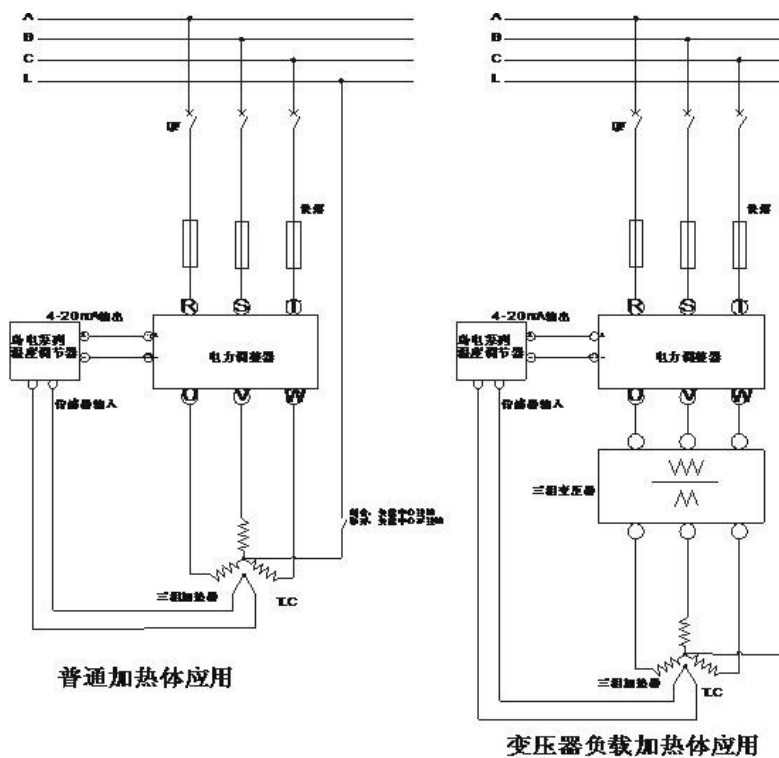
三相负载加热器星形接法(中心点接地和不接地接法)
