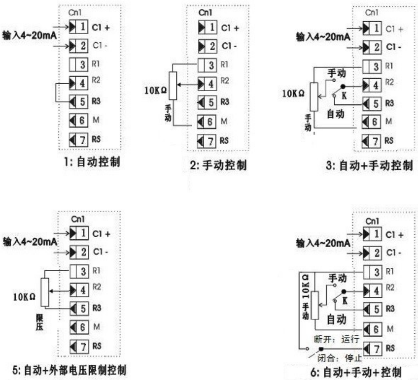
接线组合示意图
