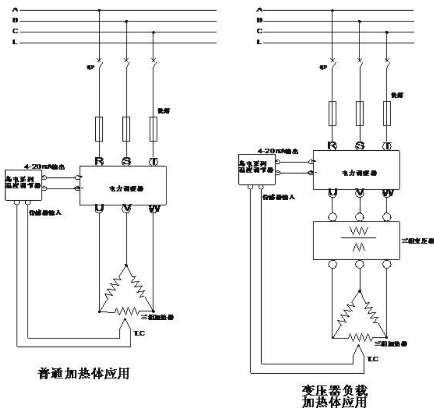
三相负载三角形接法
