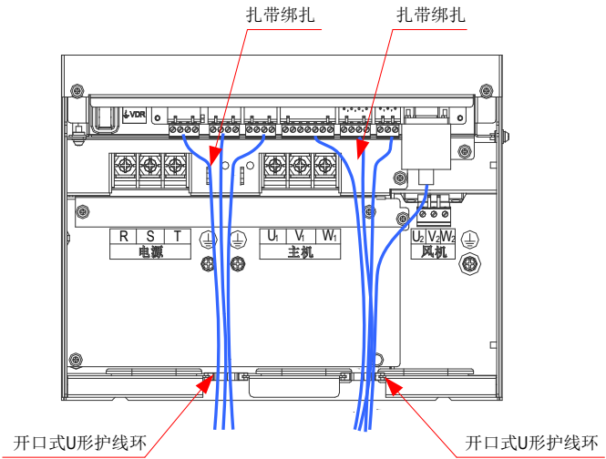
图 4-6 控制线线缆走线示意图
