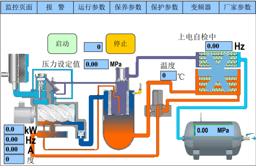
图 6-2 HMI 主页面（示意图）
