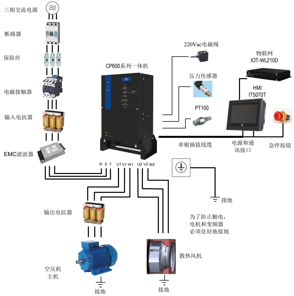
图 2-3 CP600 系统构成说明
