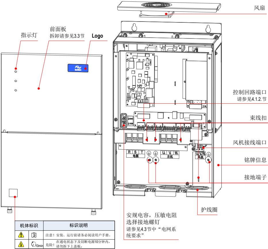
图 2-2 外观部件说明
