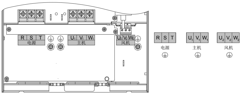
图 4-1 主回路端子分布示意图
