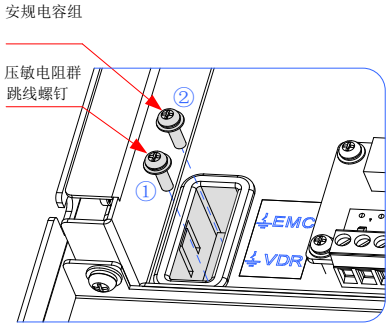
图 4-4 压敏电阻（VDR）、安规电容（EMC）对地跳线位置示意图
