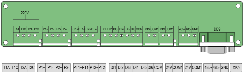
图 4-2 控制端子分布示意图
