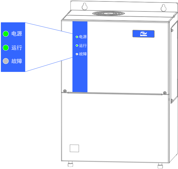
图 5-1 指示灯位置说明
