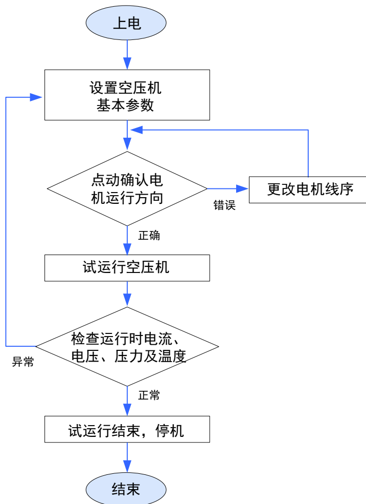
图 6-1 CP600 系列空压机一体机调试流程图
