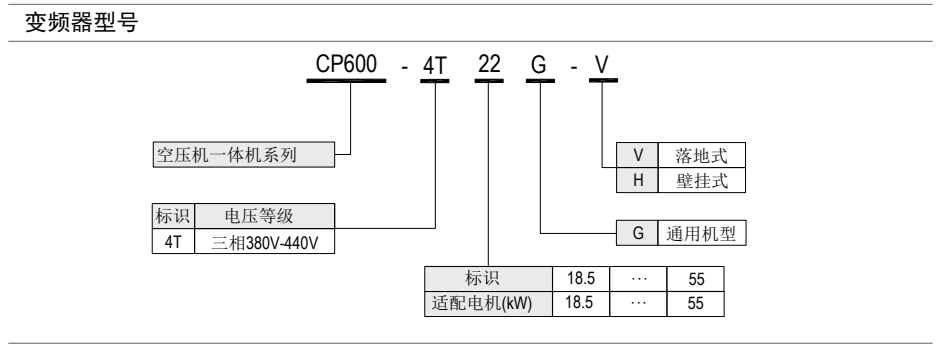
图 2-1 铭牌信息及型号说明
