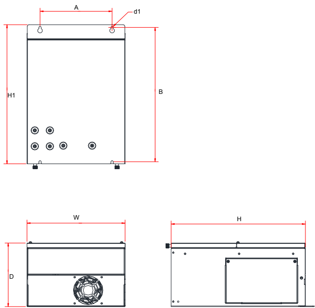
图 3-2 壁挂式机型安装尺寸示意图
