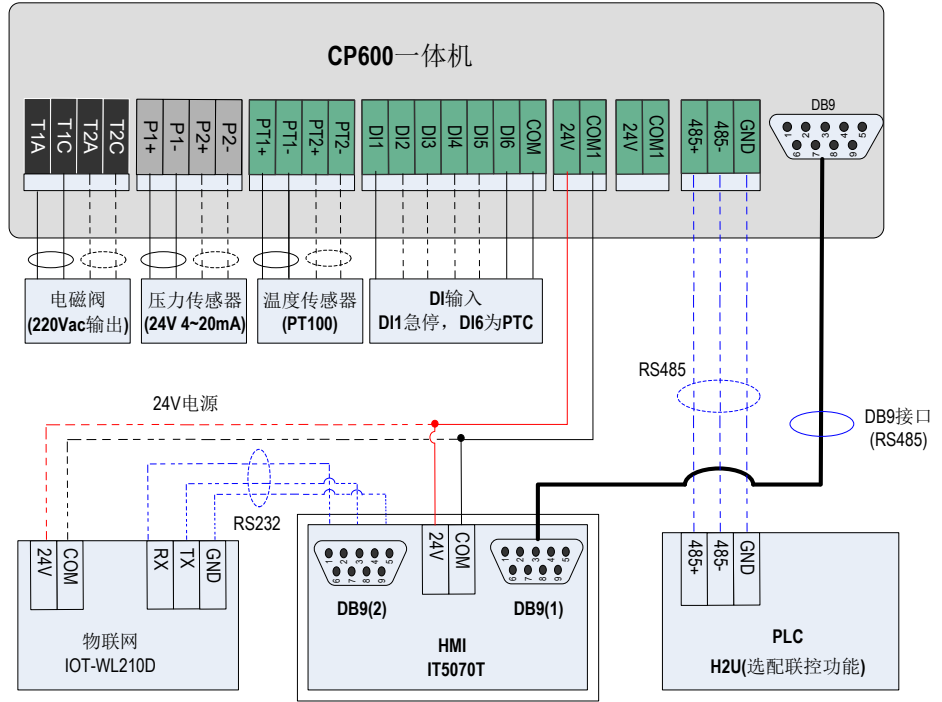
图 4-3 控制端子接线示意图
