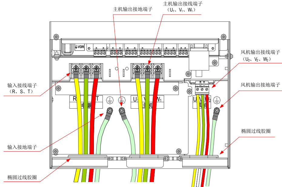
图 4-5 CP600-22G/37G 主功率线接线示意图
