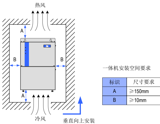
图 3-3 安装空间要求
