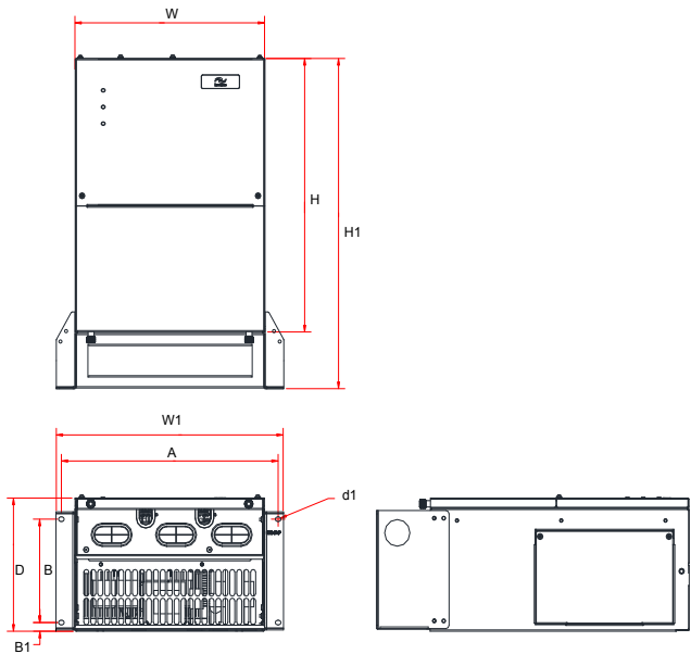
图 3-1 立柜式机型安装尺寸示意图
