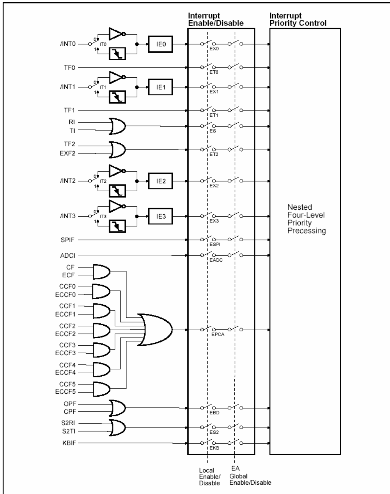
图 19-1. 中断系统
