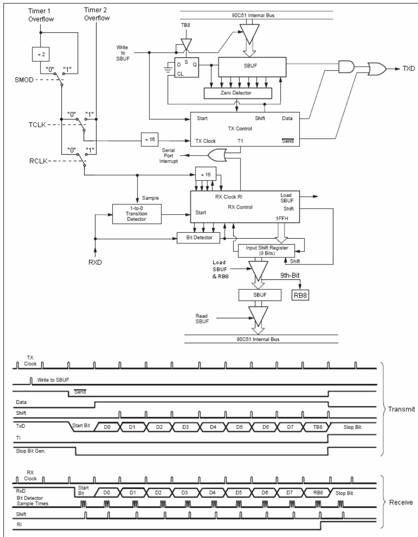
图 12-4 串行口模式 3
