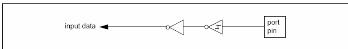
图 10-3 输入
