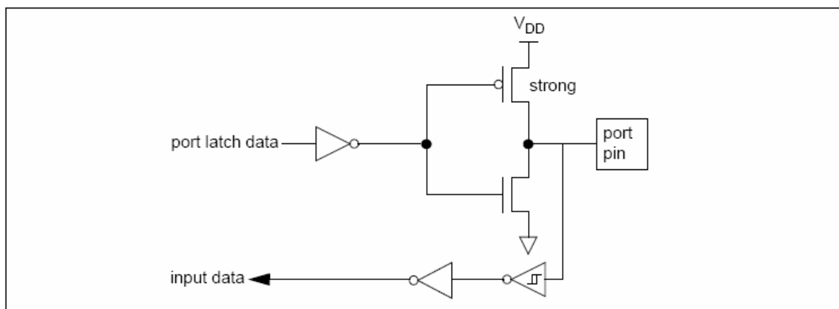
图 10-4 上拉输出
