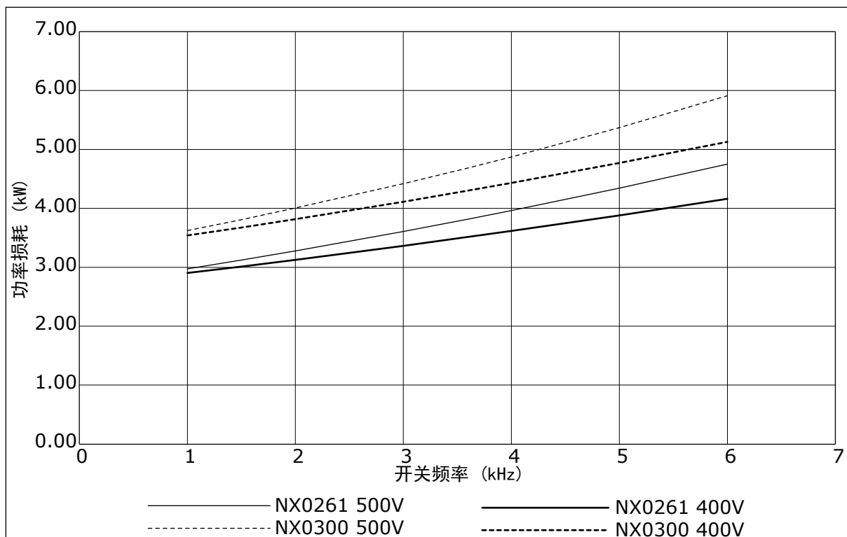
图 43: 功率损耗是开关频率的函数；NXS 或 NXP 0261-0300
