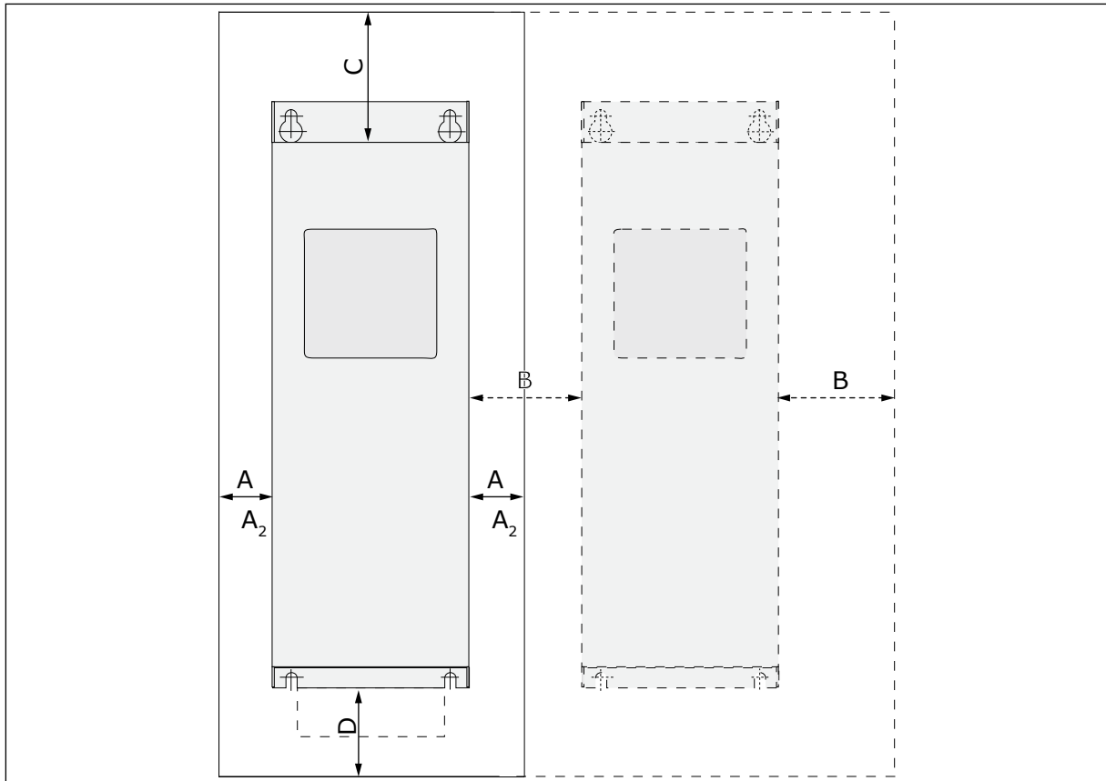
图 16: 安装空间
