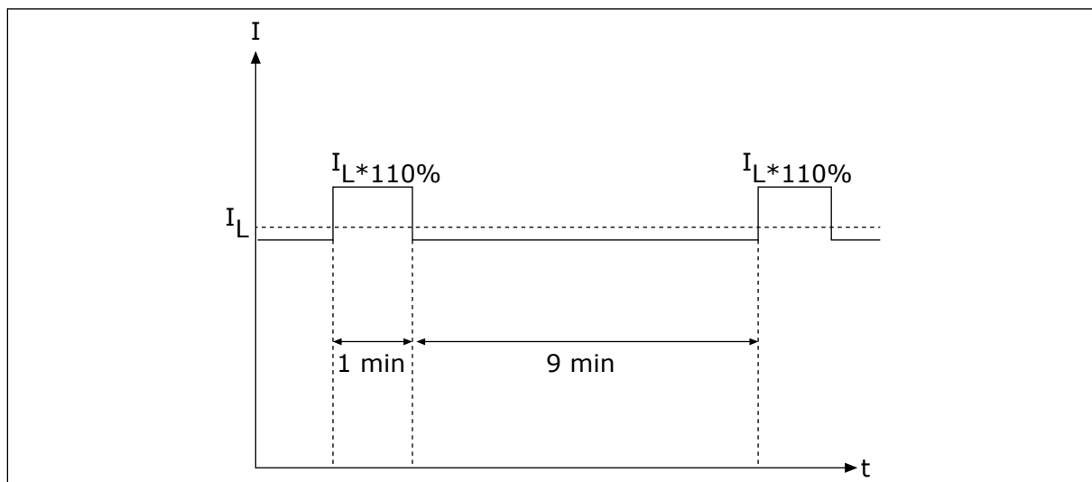
图 36: 低过载
