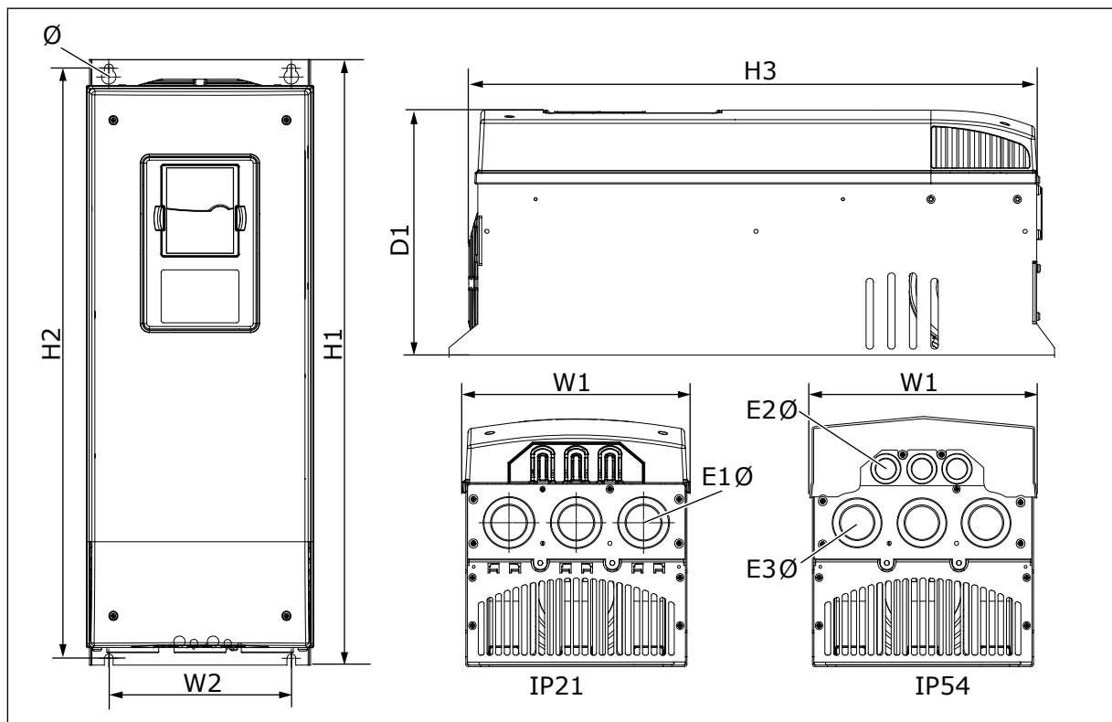
图 6: NXS 和 NXP 交流变频器的尺寸, FR7
