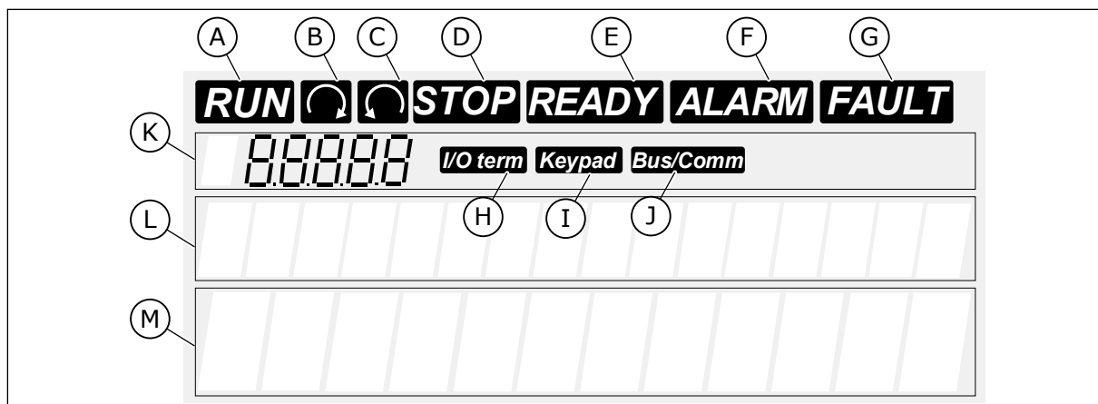
图 33: 显示屏指示
