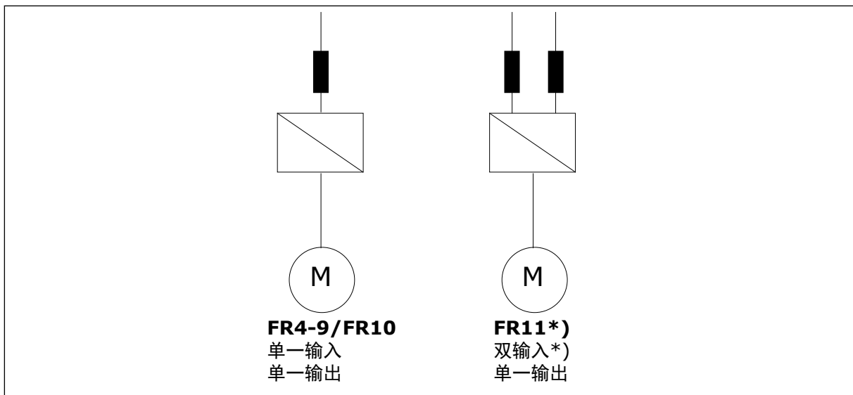
图 21: 机柜规格 FR4 – FR11 的拓扑
