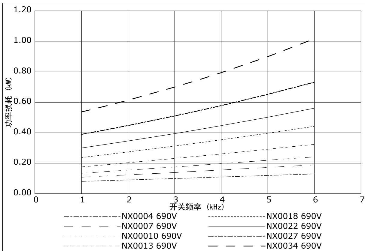
图 46: 功率损耗是开关频率的函数；NXS 或 NXP 0004-0034
