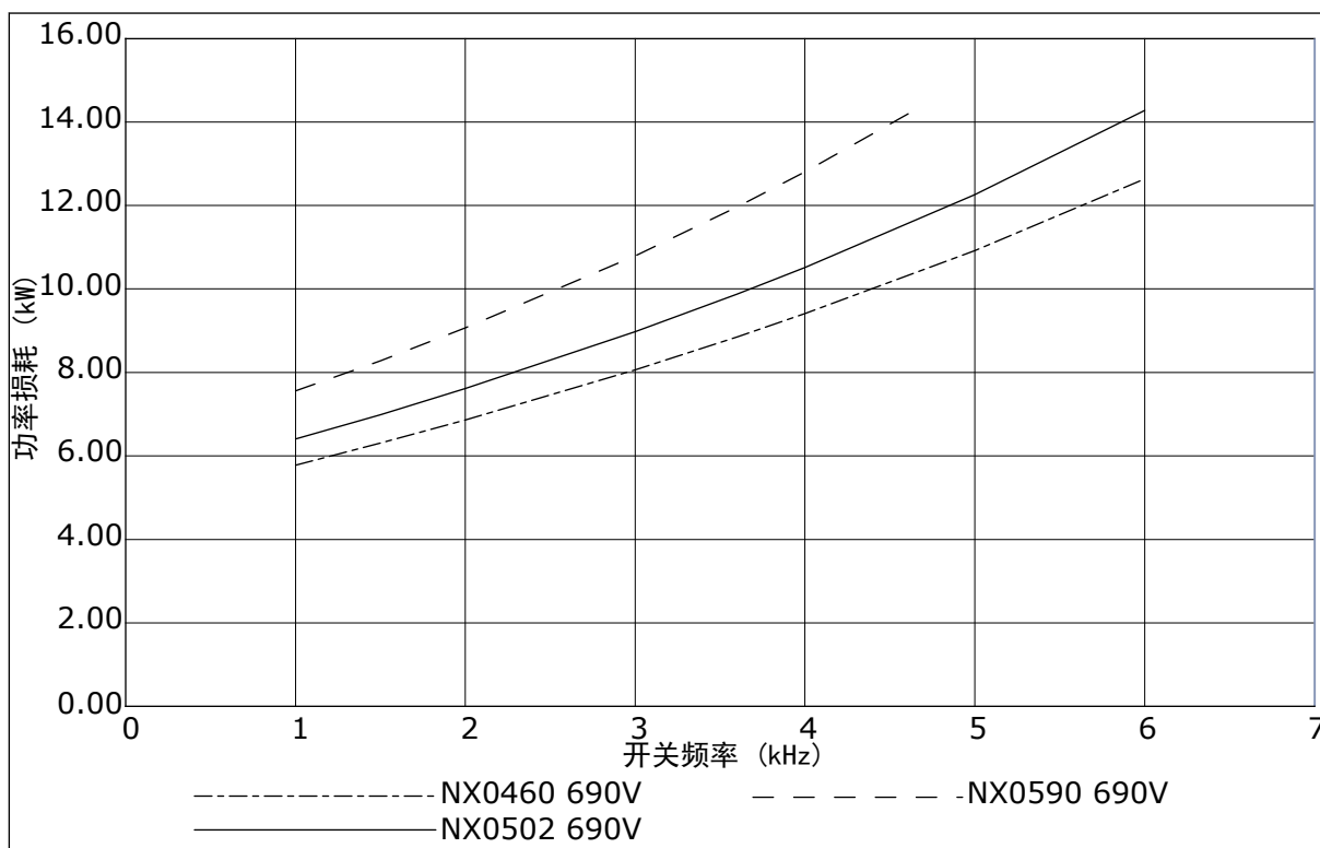
图 51: 功率损耗是开关频率的函数 ; NXS 或 NXP 0460-0590
