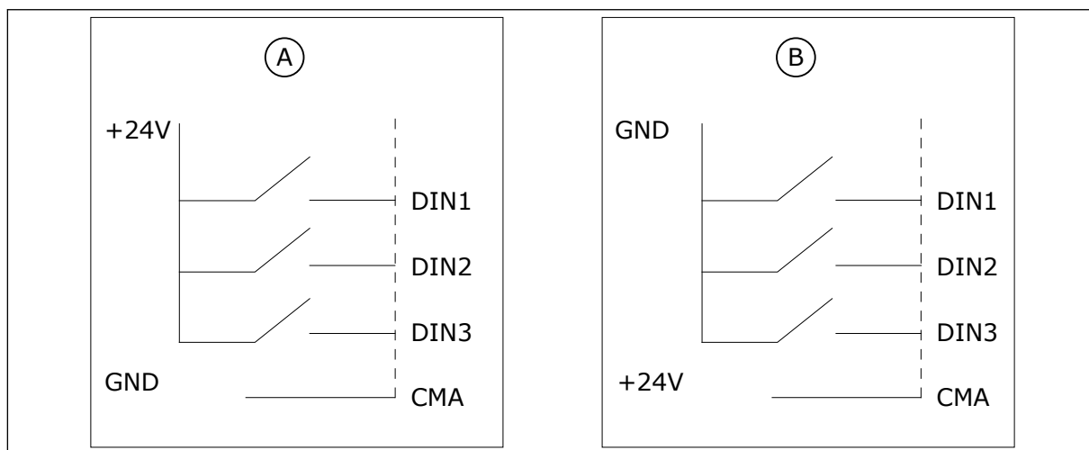
图 25: 正/负逻辑
