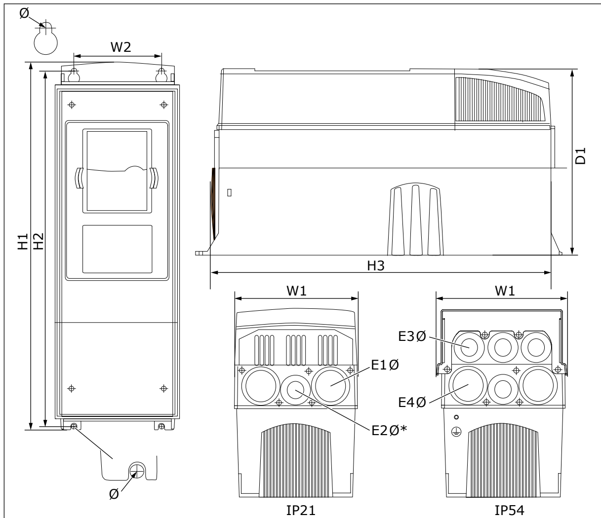
图 5: NXS 和 NXP 交流变频器的尺寸, FR4-FR6
