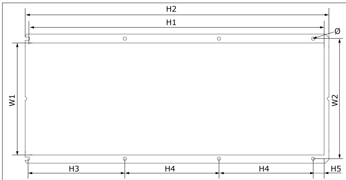
图 13: 使用法兰时的开口和变频器轮廓尺寸，FR8
