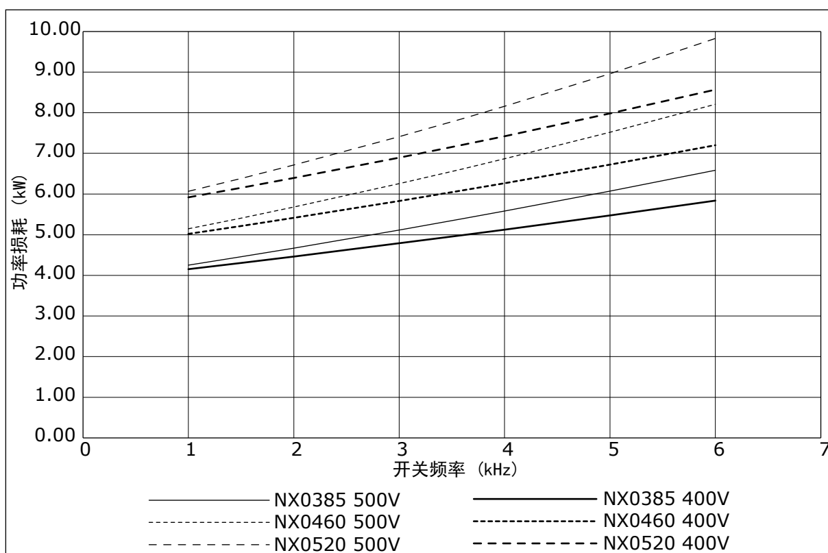
图 44: 功率损耗是开关频率的函数；NXS 或 NXP 0385-0520
