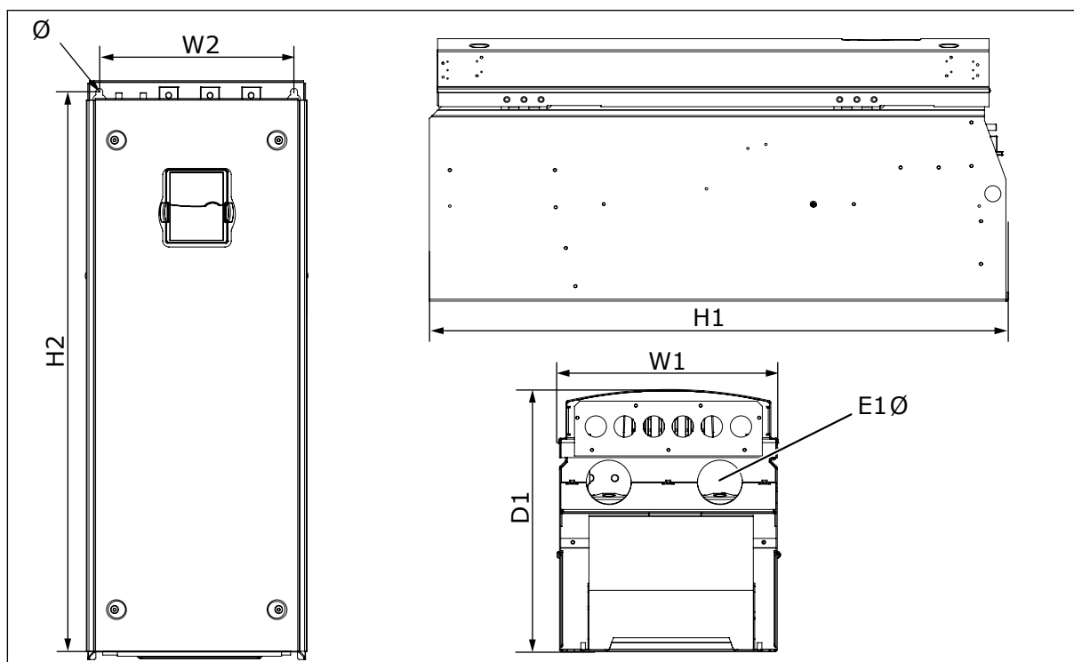
图 7: NXS 和 NXP 交流变频器的尺寸, FR8
