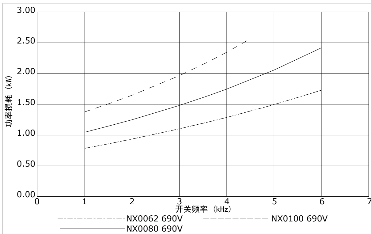
图 48: 功率损耗是开关频率的函数 ; NXS 或 NXP 0062-0100
