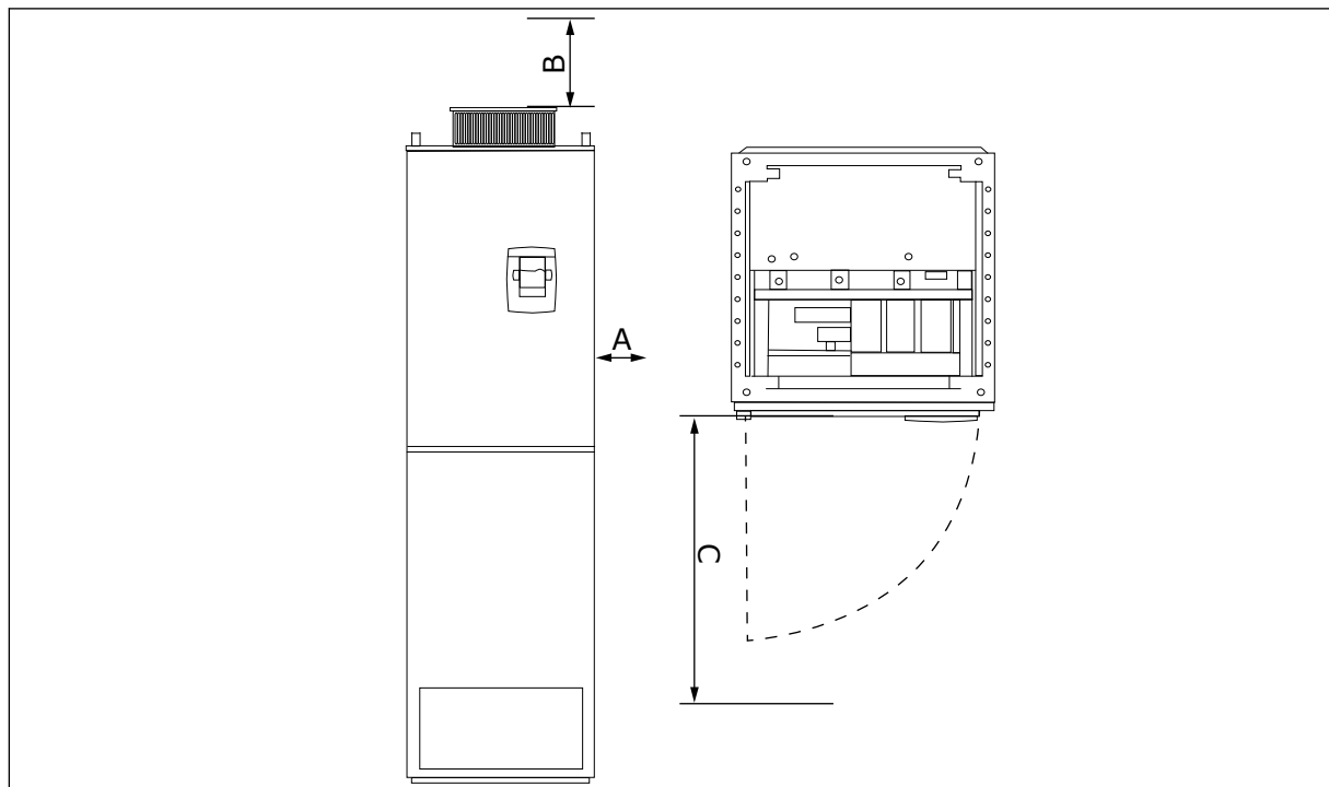
图 17: 交流变频器周围的最小间隙
