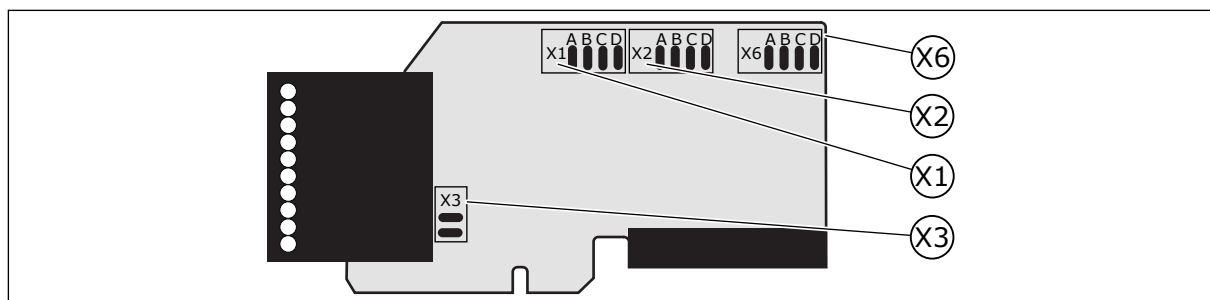
图 26: OPTA1 上的跳线块
