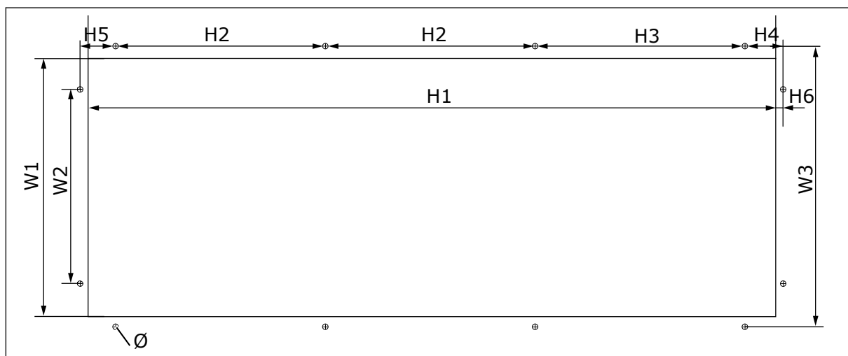
图 12: 使用法兰时的开口和变频器轮廓尺寸，FR7
