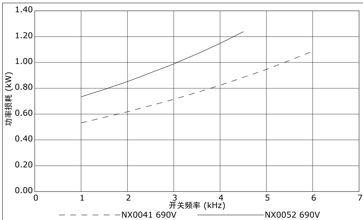
图 47: 功率损耗是开关频率的函数；NXS 或 NXP 0041-0052
