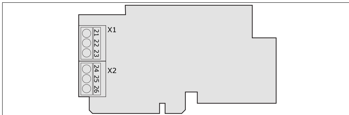
图 29: OPTA2
