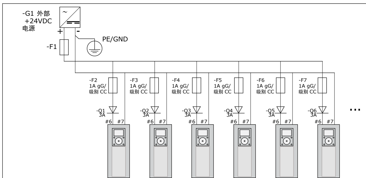
图 22: 多个交流变频器 24 V 输入的并联
