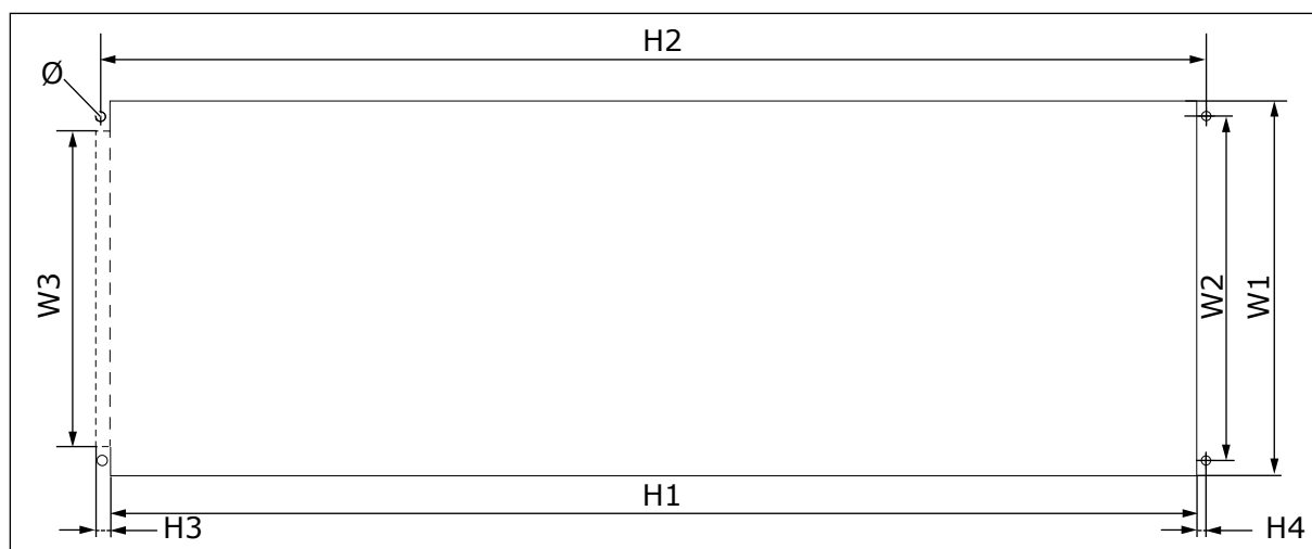
图 10: 使用法兰时的开口和变频器轮廓尺寸, FR4 至 FR6
