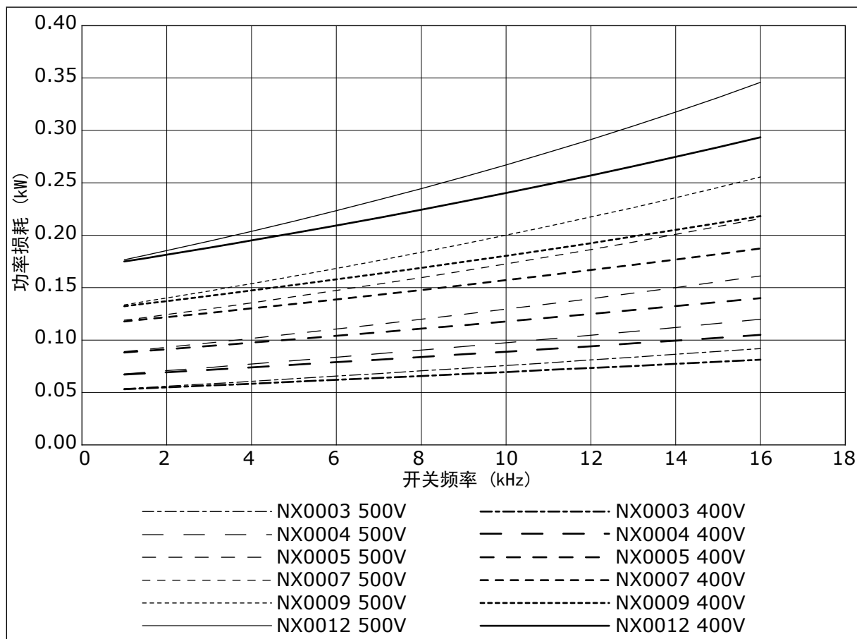
图 38: 功率损耗是开关频率的函数；NXS 或 NXP 0003-0012
