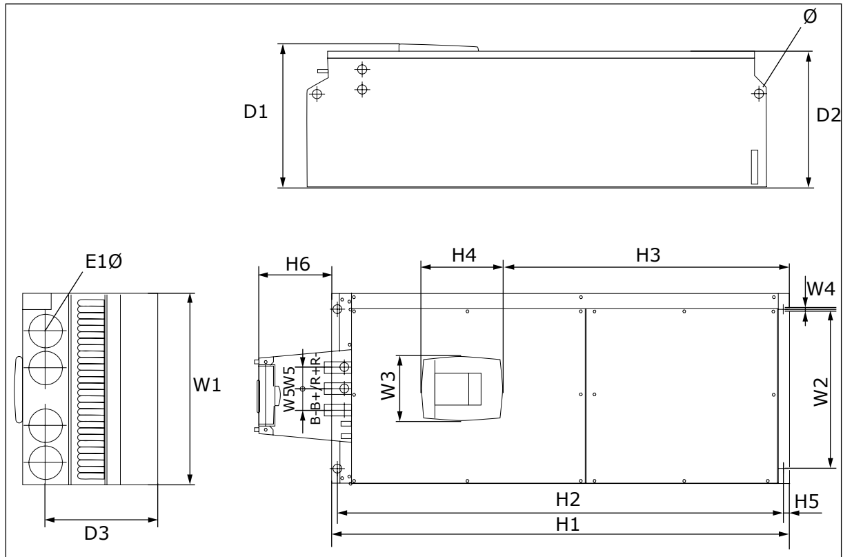
图 8: NXS 和 NXP 交流变频器的尺寸, FR9
