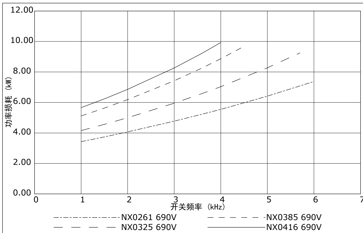
图 50: 功率损耗是开关频率的函数 ; NXS 或 NXP 0261-0416
