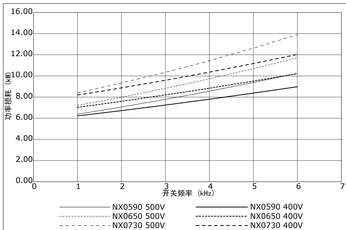
图 45: 功率损耗是开关频率的函数；NXS 或 NXP 0590-0730
