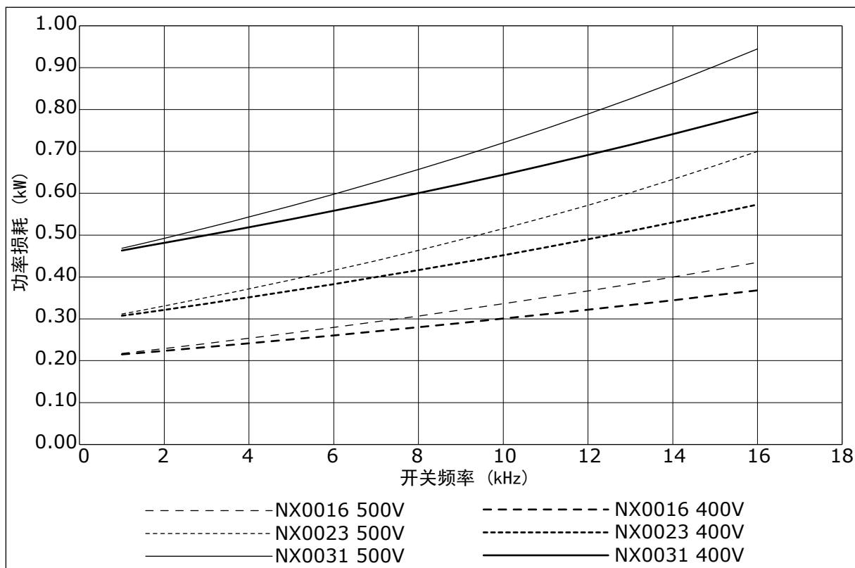
图 39: 功率损耗是开关频率的函数；NXS 或 NXP 0016-0031
