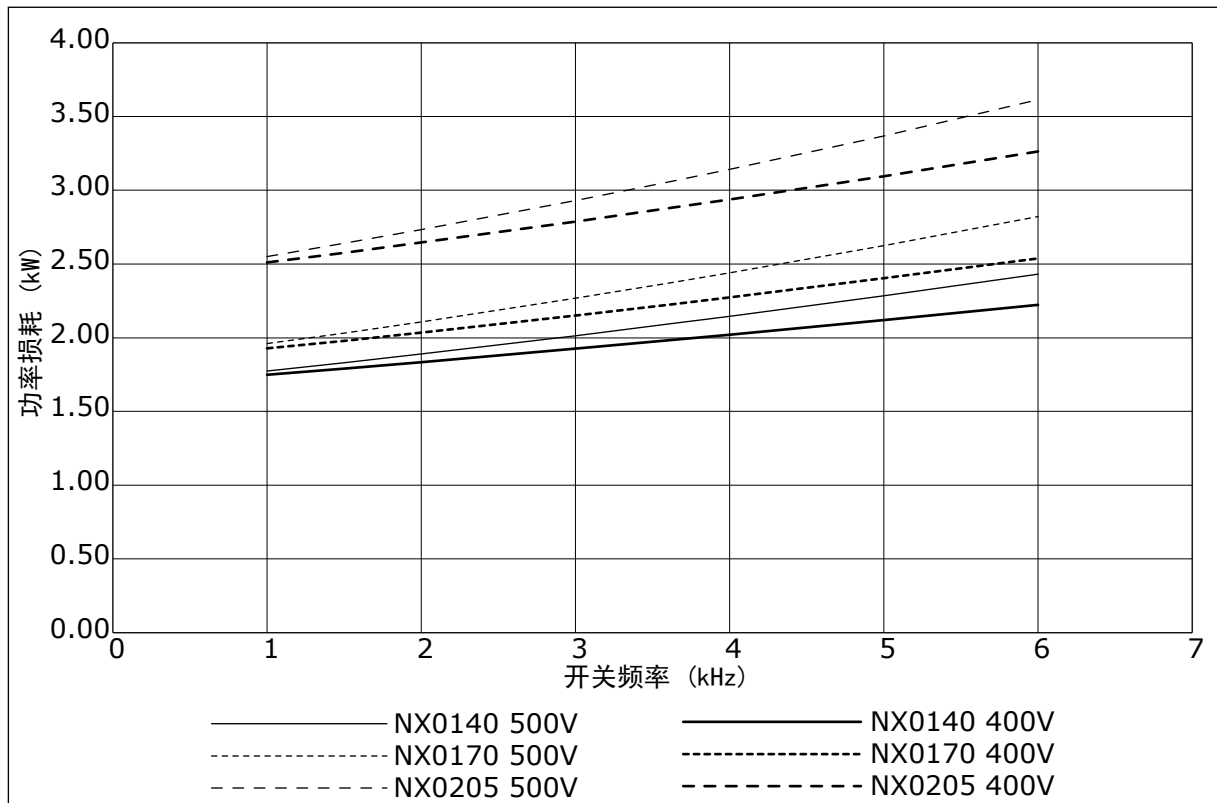
图 42: 功率损耗是开关频率的函数；NXS 或 NXP 0140-0205
