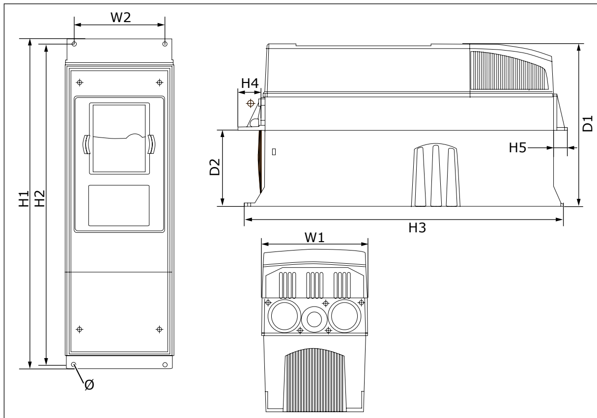
图 9: 带法兰的 NXS 和 NXP 交流变频器的尺寸, FR4-FR6
