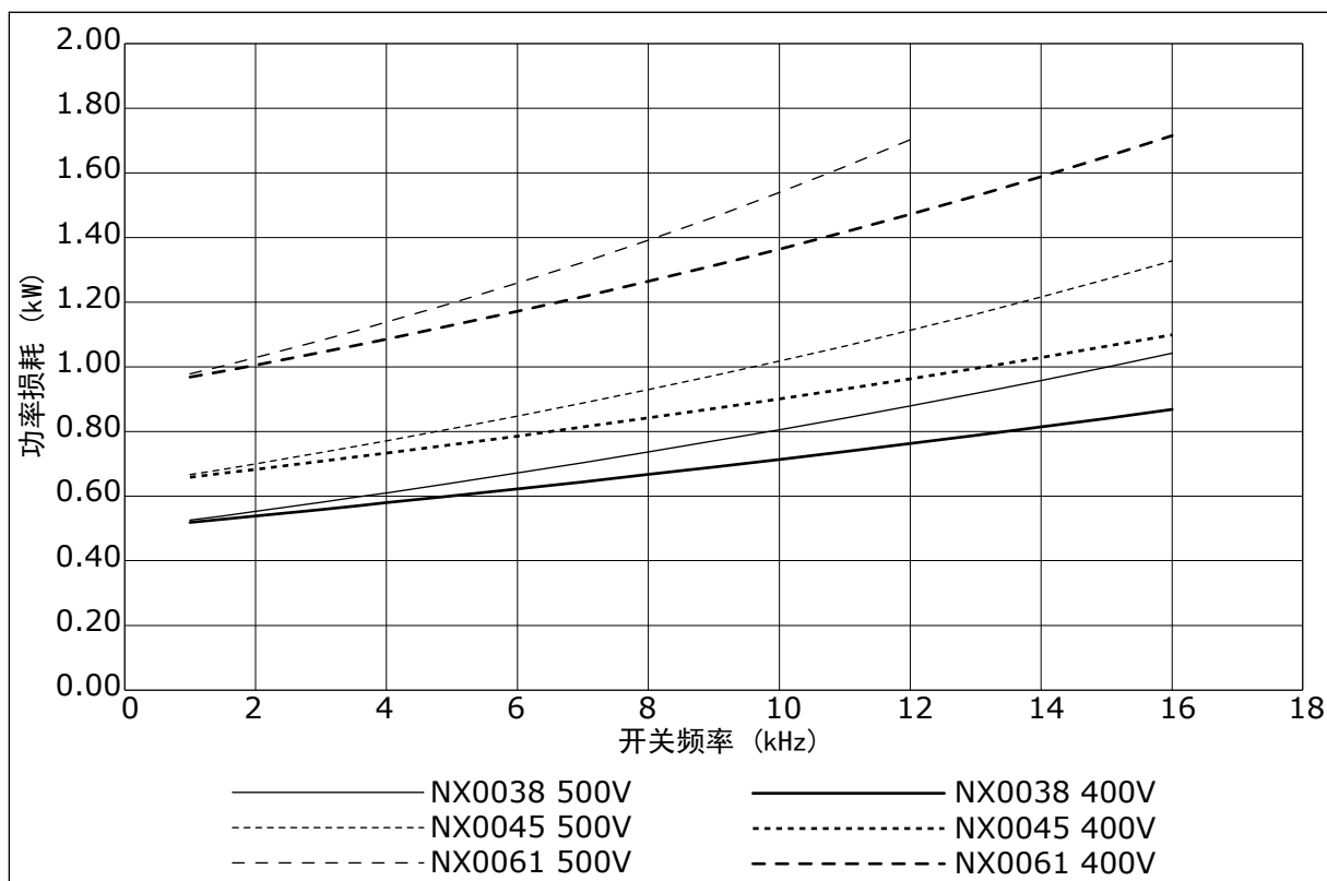
图 40: 功率损耗是开关频率的函数；NXS 或 NXP 0038-0061
