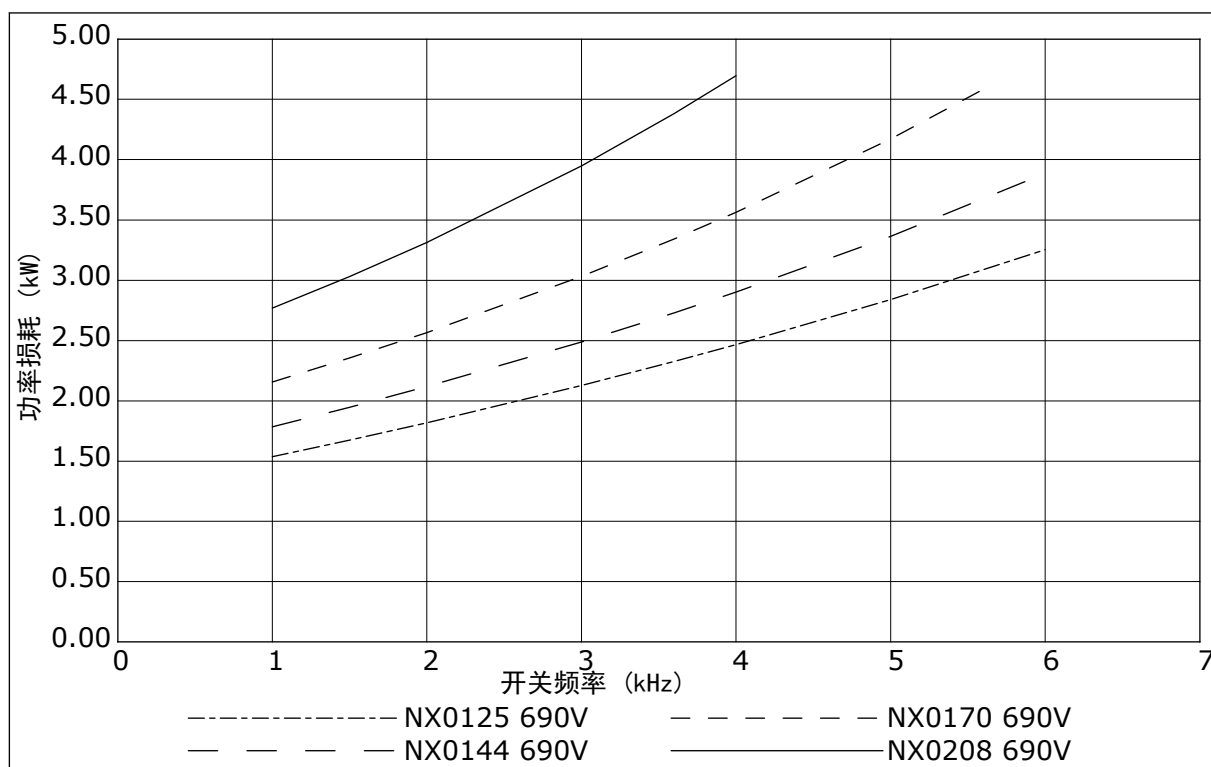
图 49: 功率损耗是开关频率的函数 ; NXS 或 NXP 0125-0208
