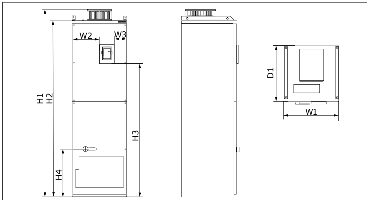
图 15: NXS 和 NXP 交流变频器的尺寸, FR10 和 FR11
