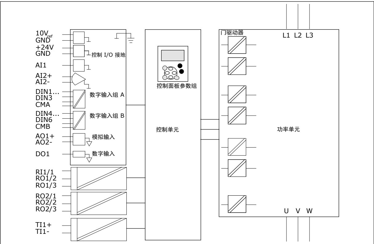
图 31: 电隔离屏障
