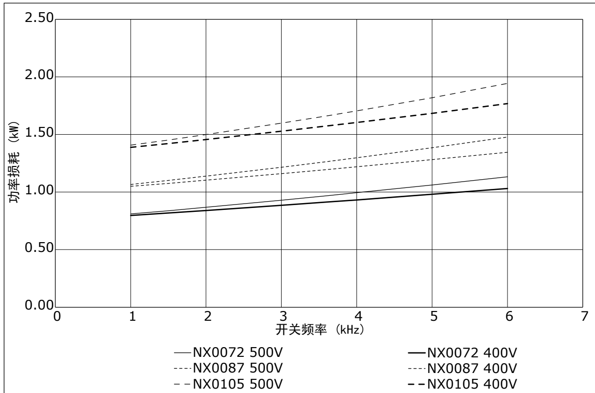
图 41: 功率损耗是开关频率的函数；NXS 或 NXP 0072-0105
