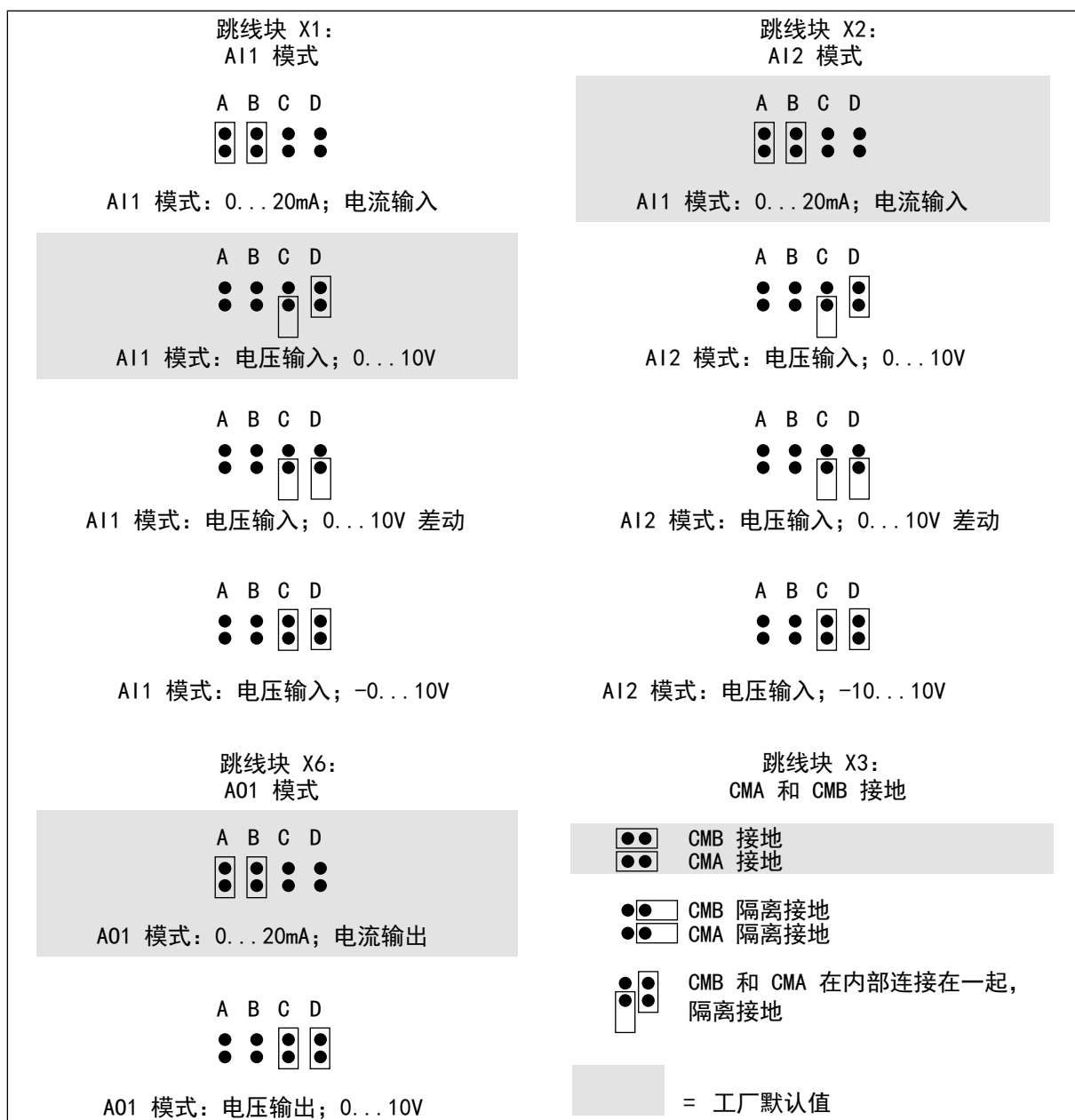
图 27: OPTA1 的跳线选择
