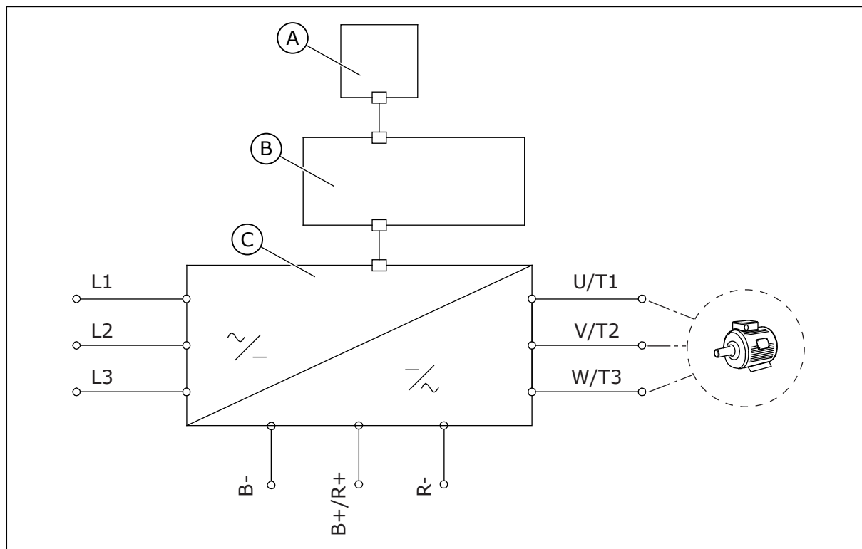
图 19: 主要连接图
