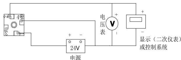
三线制电压输出接线图(JYB-K*-HV**)
