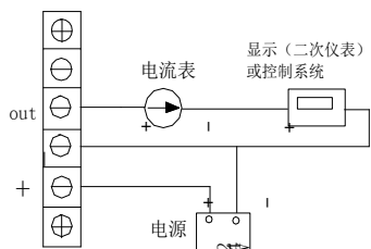
端子接线, 三线电流输出 三线制电流输出接线图(JYB-K*-WPA1*-**)
