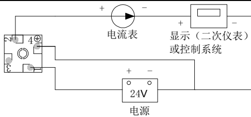
三线制电流输出接线图(JYB-K*-HA1**)
