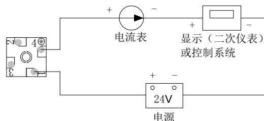
二线制电流输出接线图(JYB-K*-HA**)
