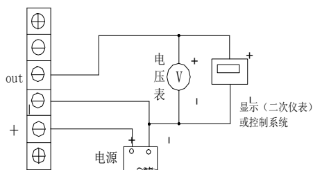
三线电压输出接线图(JYB-K*-WPV*-**)
