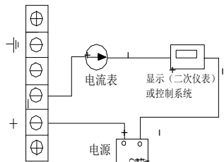
二线制电流输出接线图(JYB-K*-WPA*-**)
