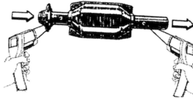
测量三元催化器进出口温度
