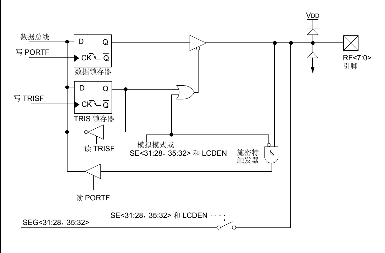
图 3-28: RF<7:0> 框图
