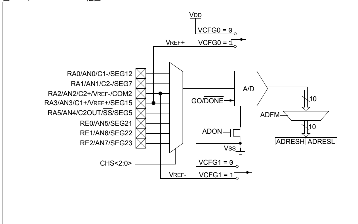
图 12-1: A/D 框图
