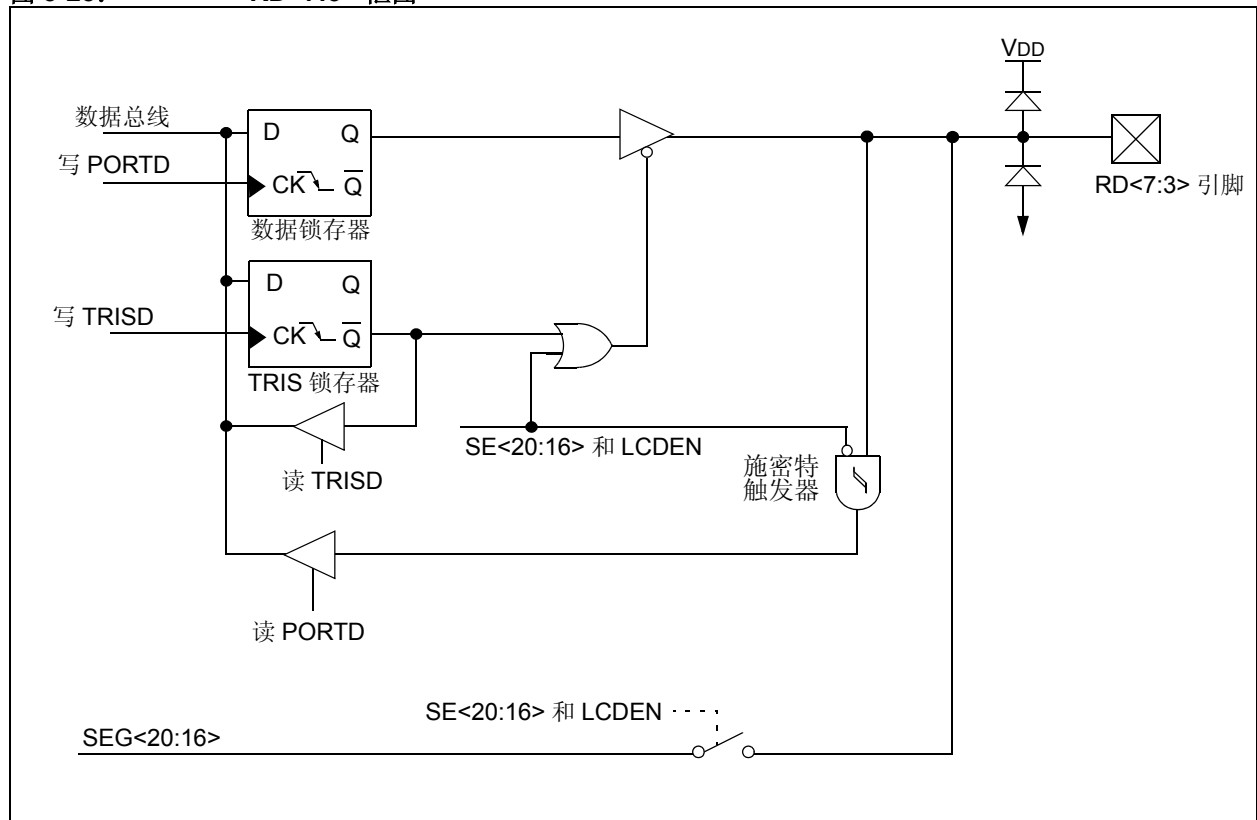
图 3-25: RD<7:3> 框图
