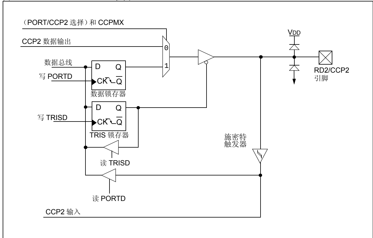
图 3-24: RD2/CCP2 框图
