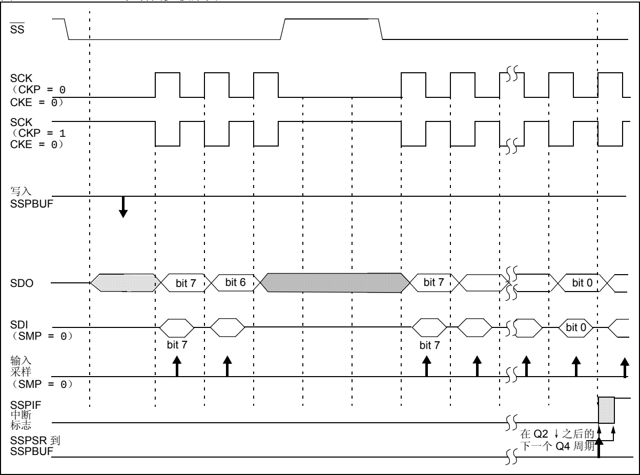
图 14-4: 从动同步波形图
