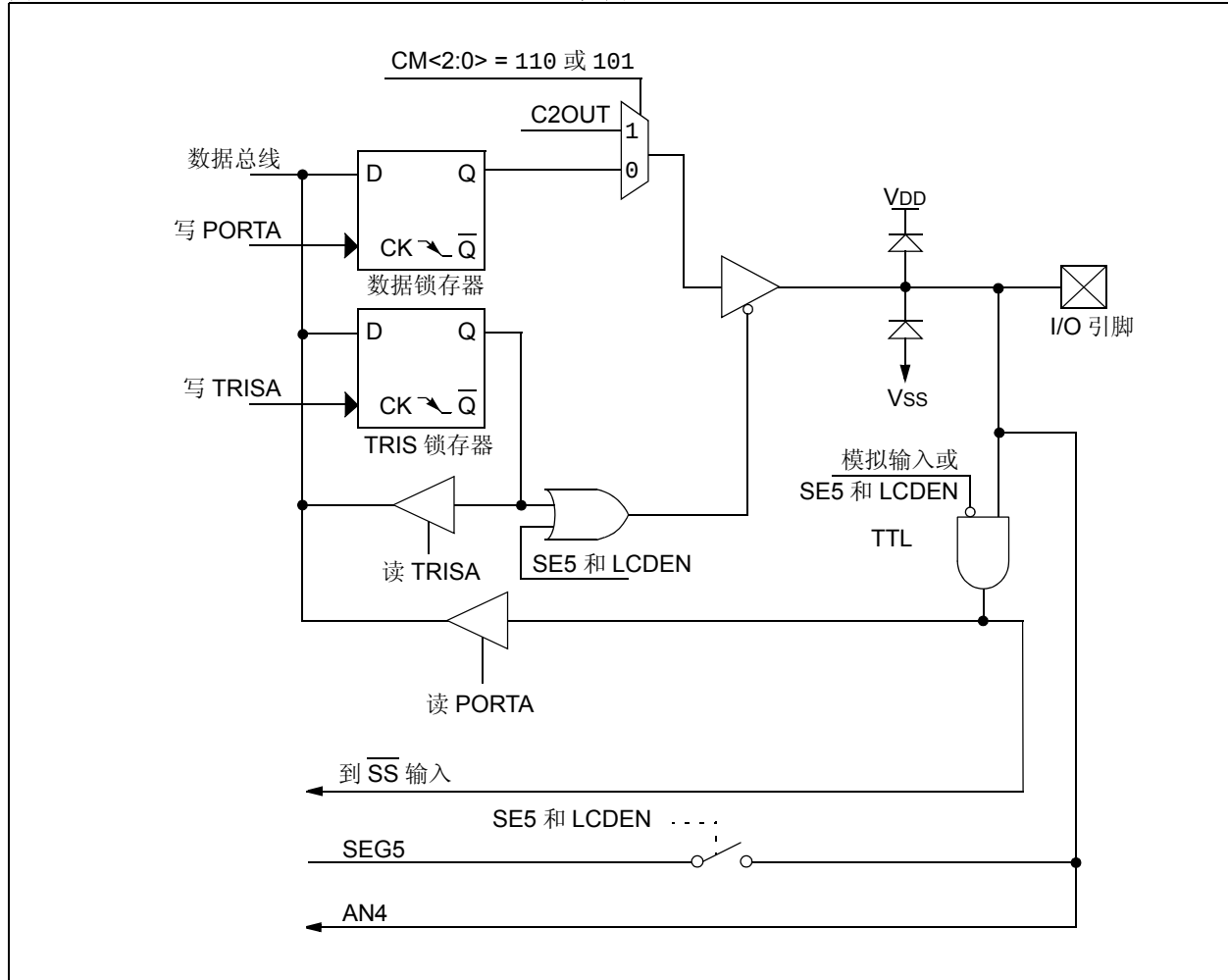
图 3-6: RA5/AN4/C2OUT/ \overline{\text{SS}} /SEG5 框图
