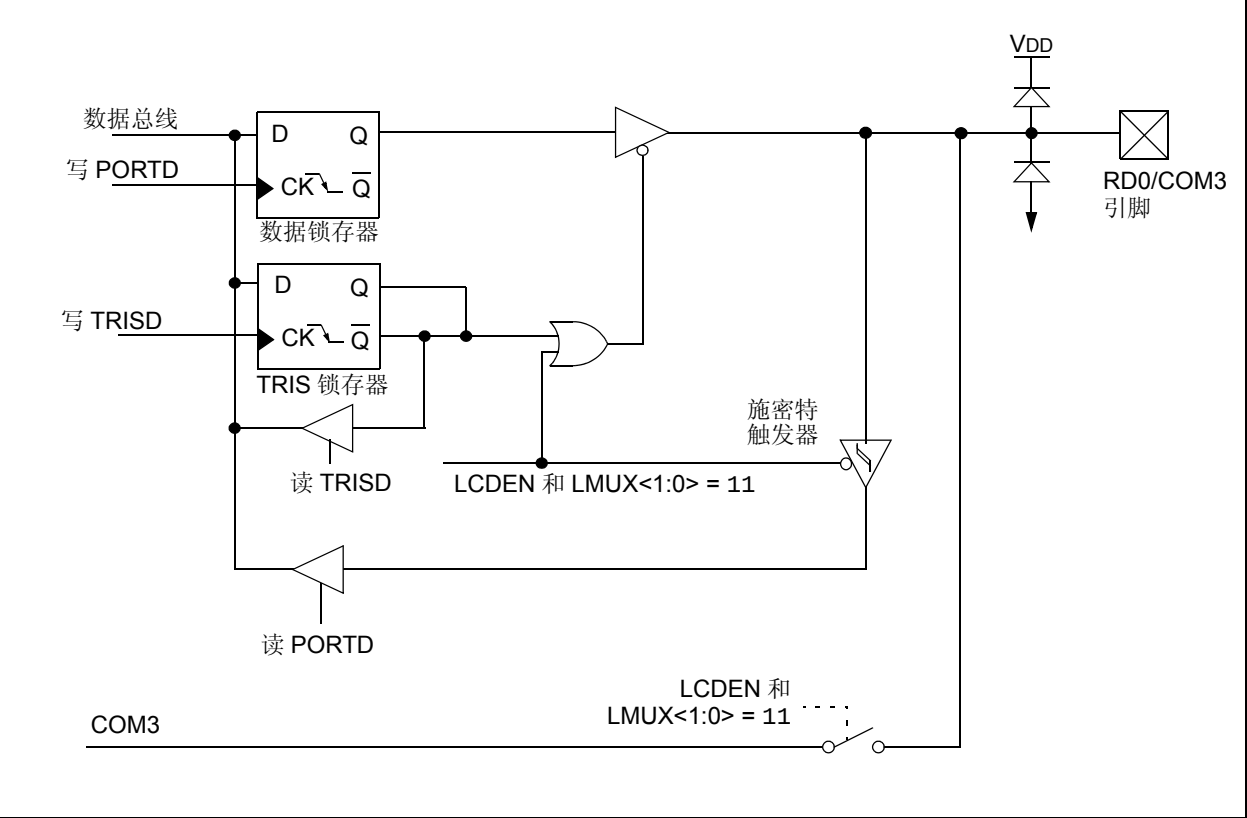
图 3-22: RD0/COM3 框图
