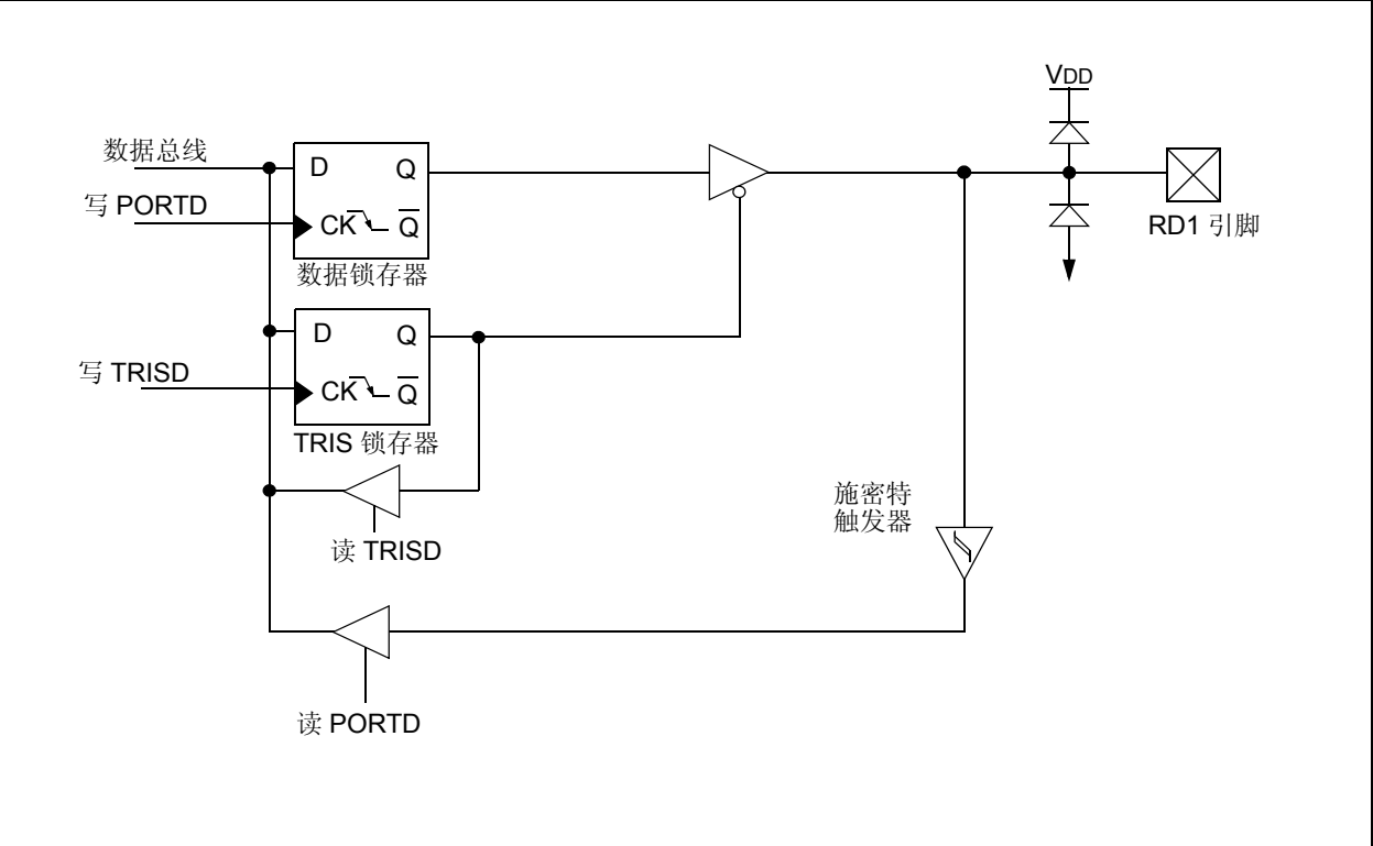
图 3-23: RD1 框图
