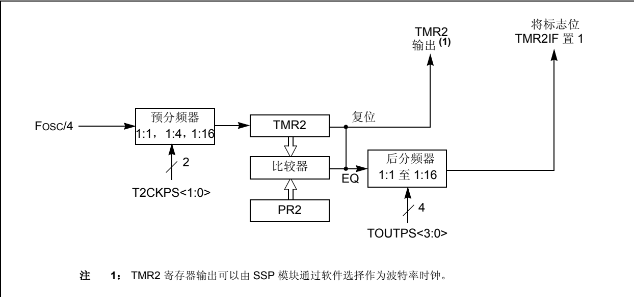
图 7-1: TIMER2 框图
