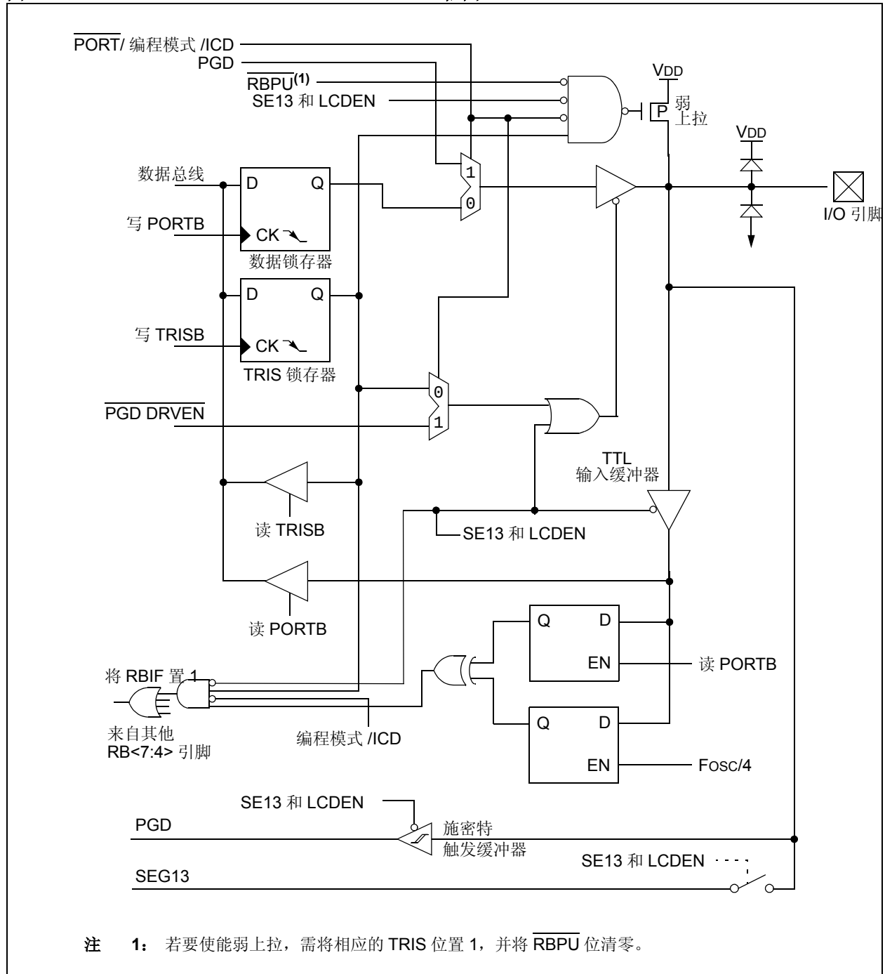
图 3-13: RB7/ICSPDAT/ICDDAT/SEG13 框图
