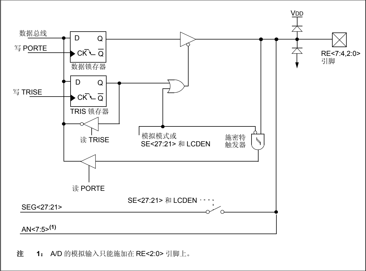
图 3-26: RE<7:4, 2:0> 框图
