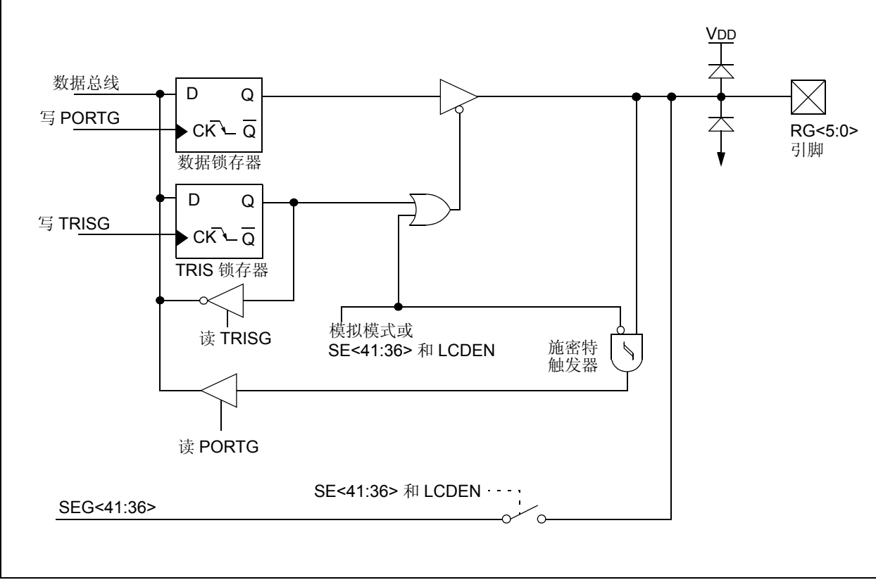
图 3-29: RG<5:0> 的框图
