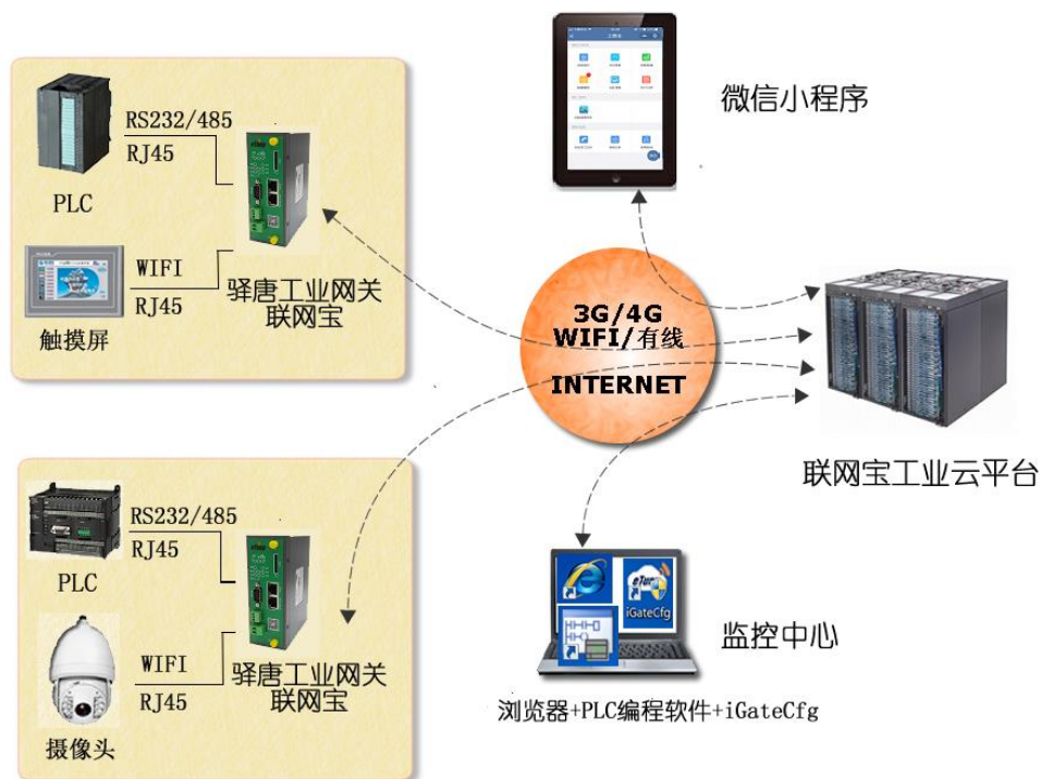
图 1-6: 工作原理图
