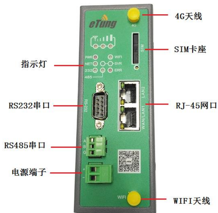
图 1-1: PLC-502 PRO 外观图
