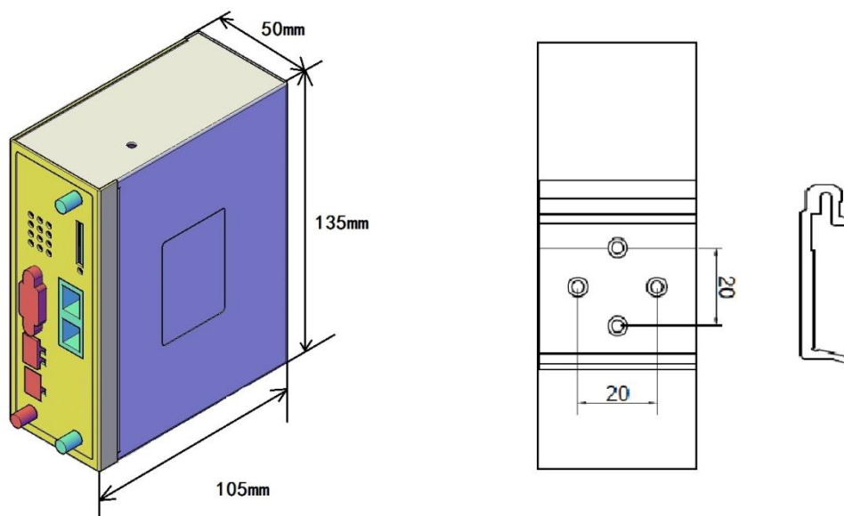
图 1-5: 安装尺寸
