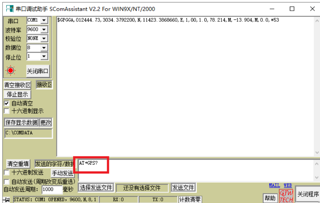
图附 3-3：通过串口 AT 命令查看位置信息
