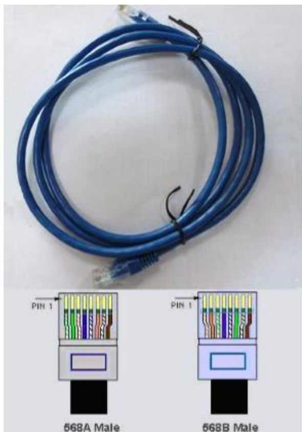
图 1-4: 交叉网线
