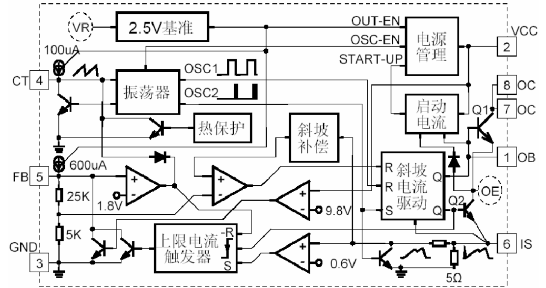
内部电路参考框图
