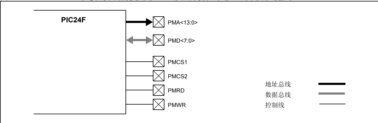
图 17-4: 主控模式下的解复用寻址（单独的读和写选通、两个片选信号）
