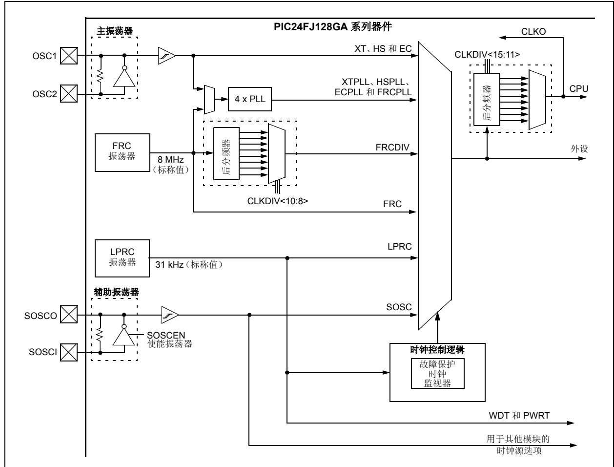
图 7-1: PIC24FJ128GA 系列器件时钟框图
