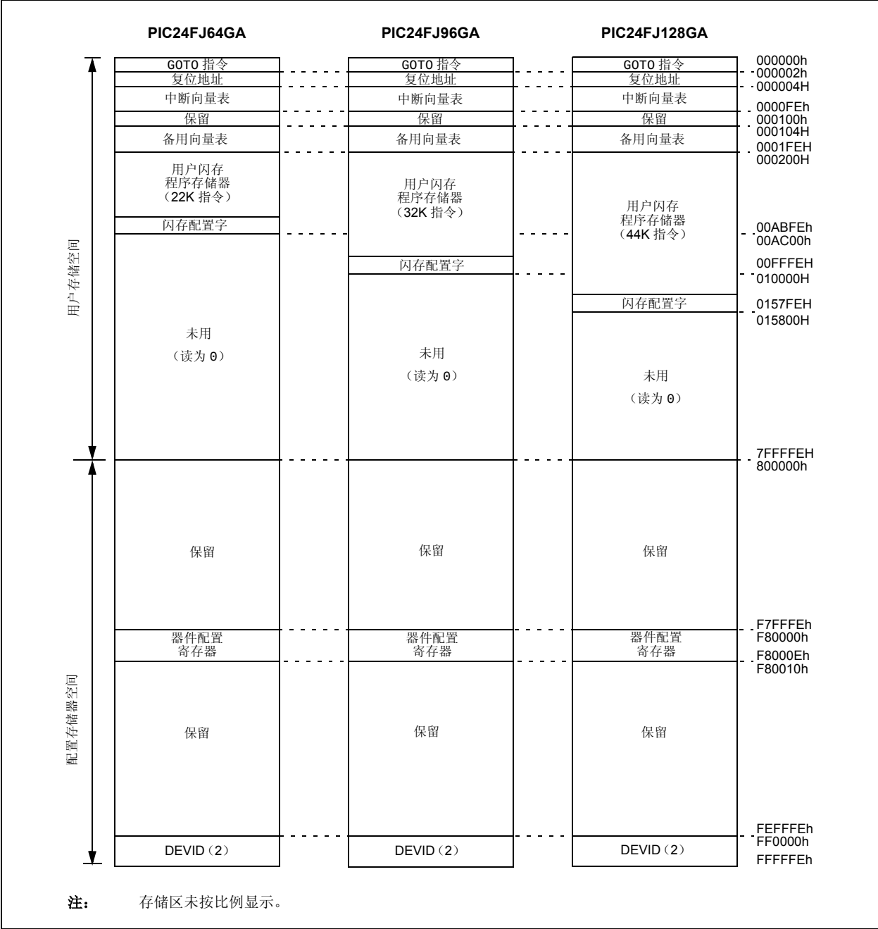
图 3-1: PIC24FJ128GA 系列器件的程序空间存储器映射
