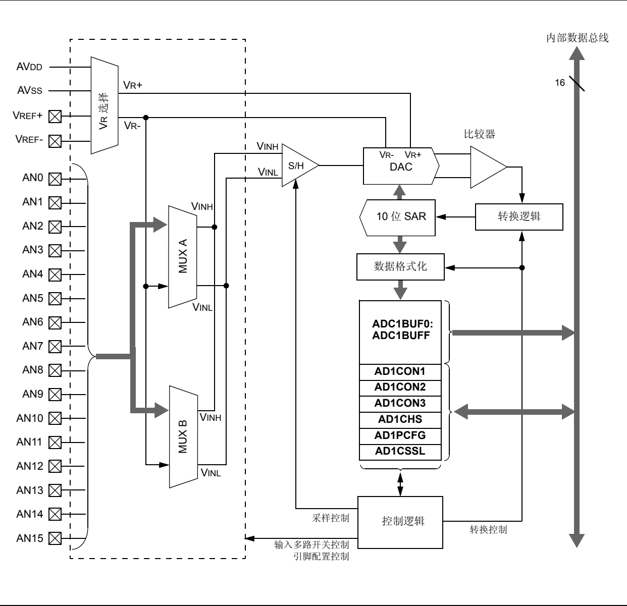
图 20-1: 10 位高速 A/D 转换器框图
