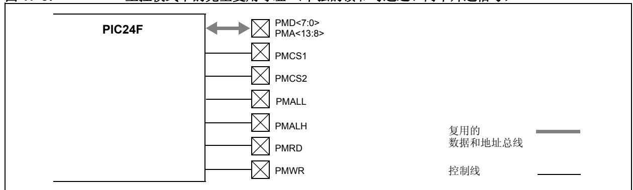
图 17-6: 主控模式下的完全复用寻址（单独的读和写选通、两个片选信号）
