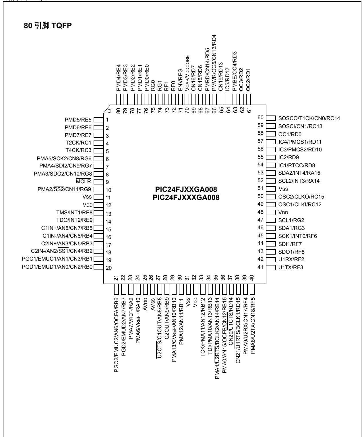
引脚图 (续)
