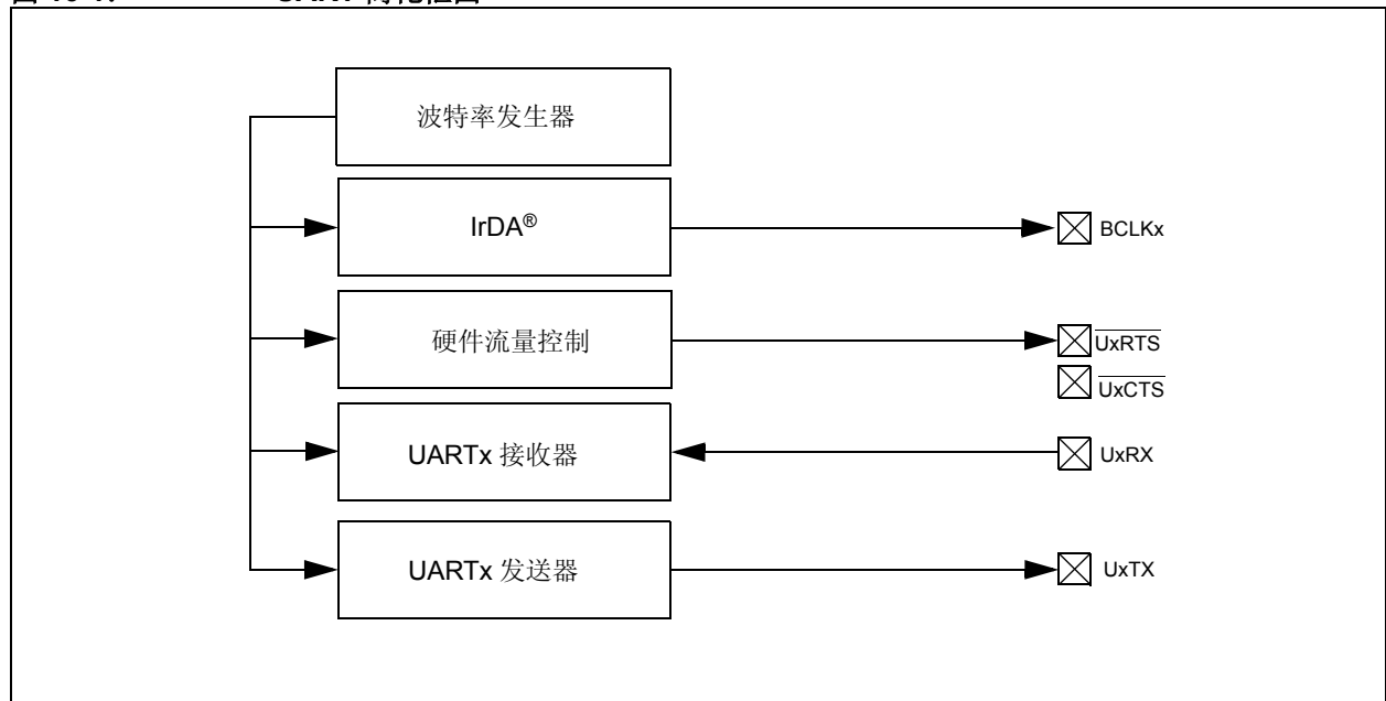
图 16-1: UART 简化框图
