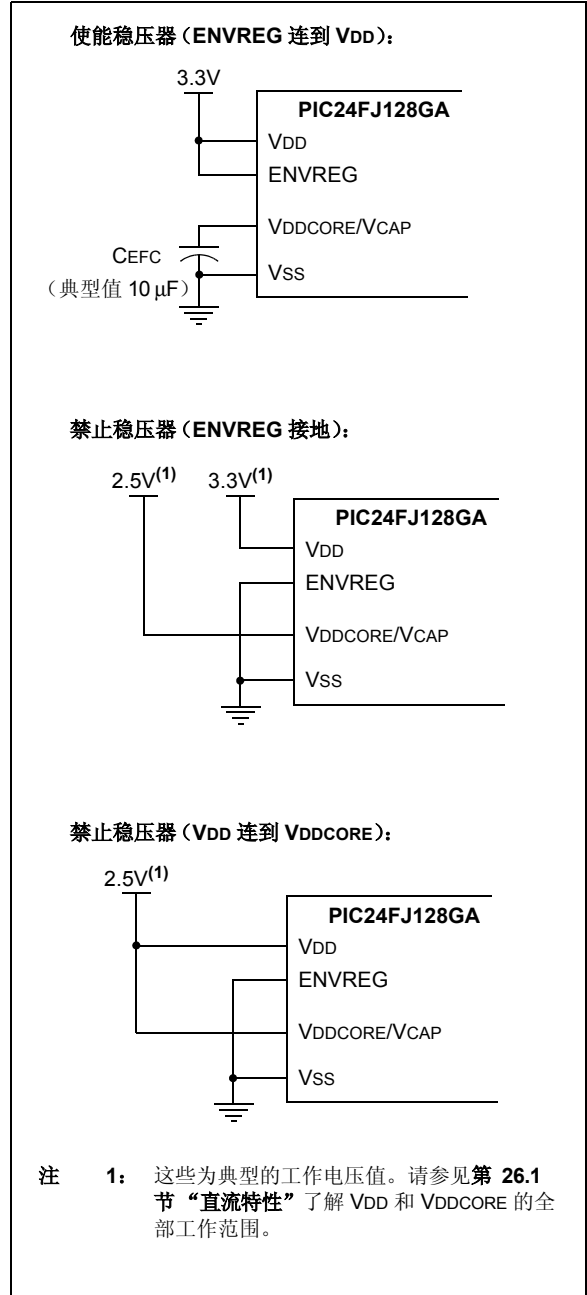
图 23-1: 片内稳压器连接
