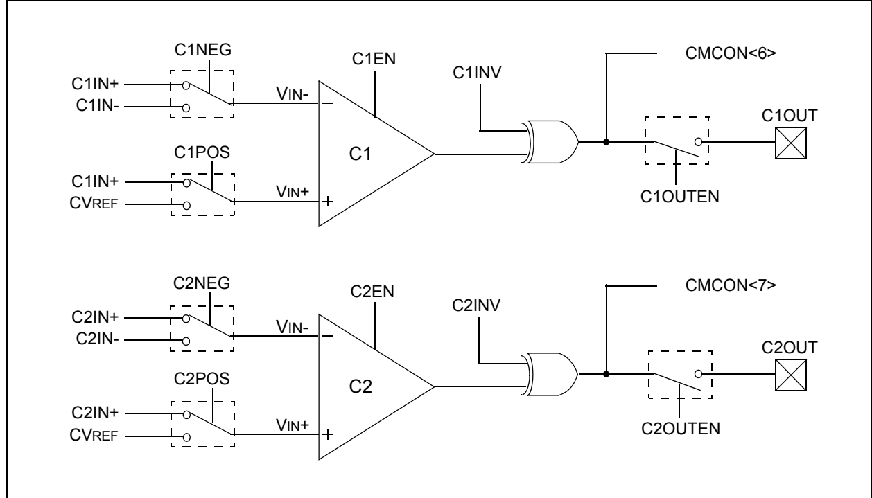
图 21-1: 比较器 I/O 工作模式
