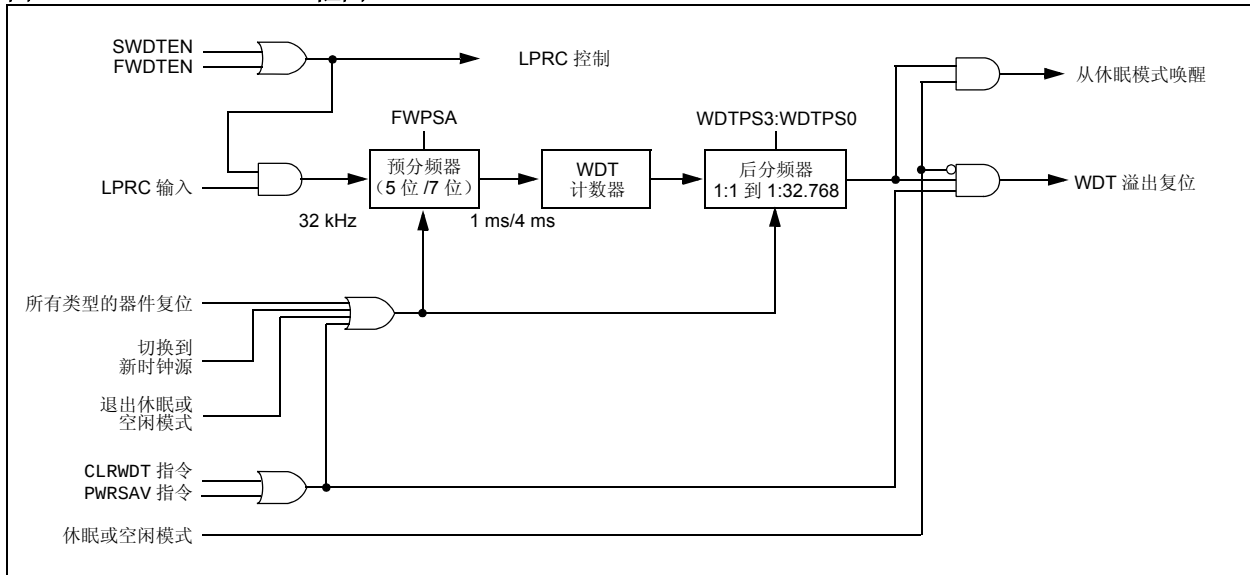
图 23-2: WDT 框图
