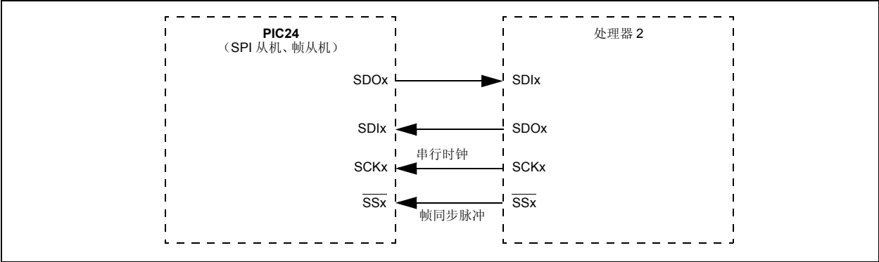
图 14-7: SPI 从机、帧从机连接图
