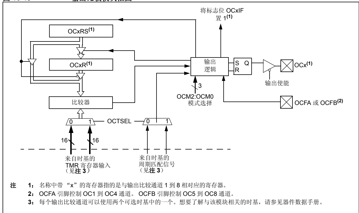
图 13-1: 输出比较模块框图
