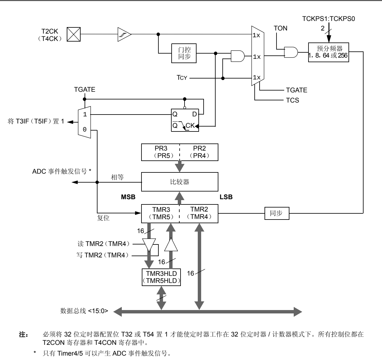
图 11-1: TIMER2/3 和 TIMER4/5 (32 位) 框图
