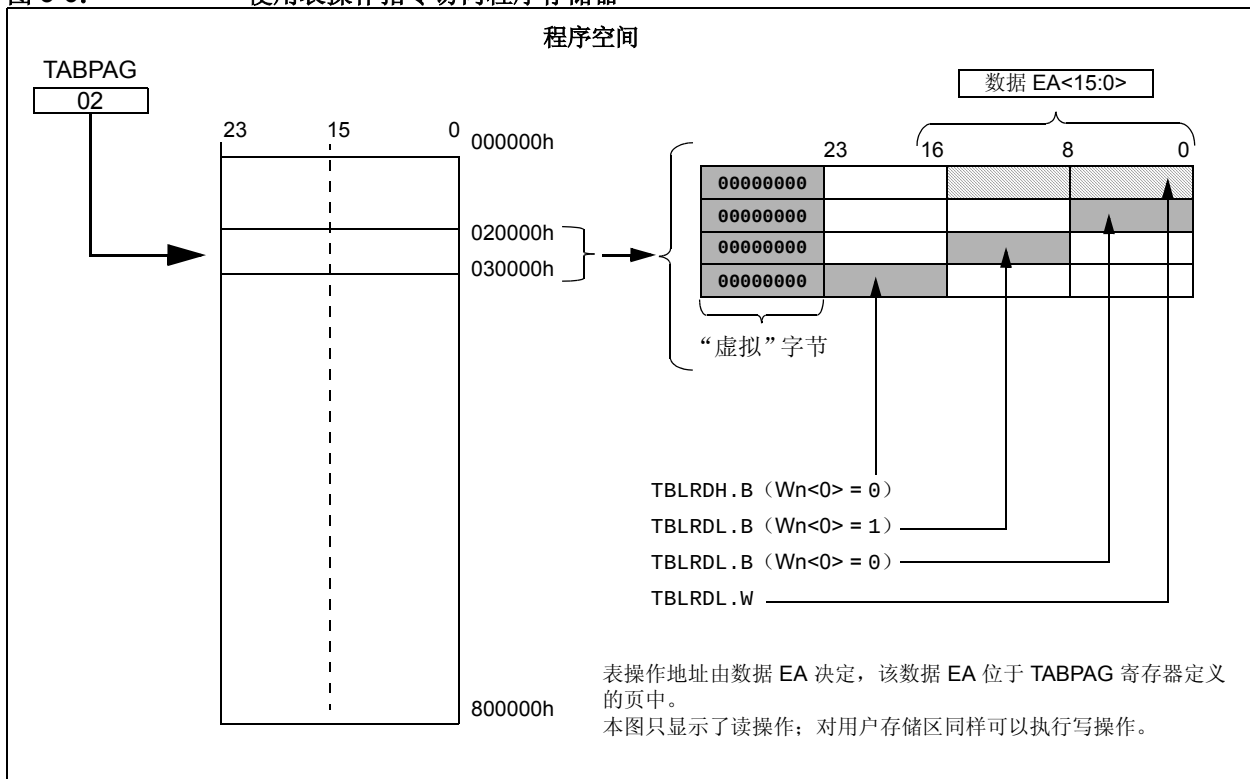
图 3-6: 使用表操作指令访问程序存储器
