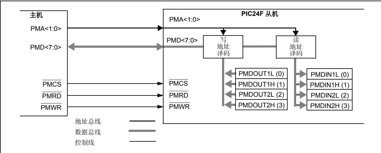
图 17-3: 可寻址并行从动端口示例
