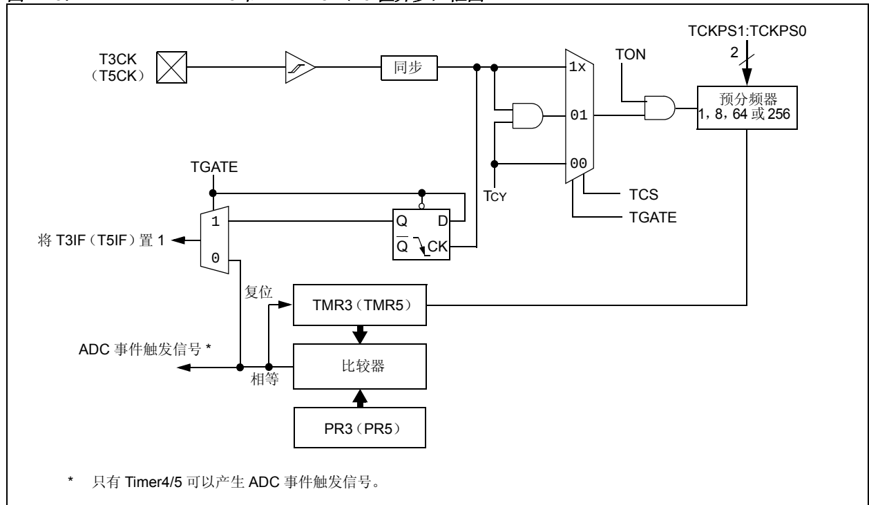
图 11-3: TIMER3 和 TIMER5 (16 位异步) 框图
