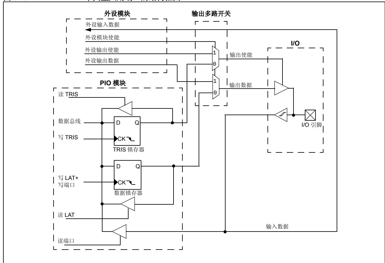
图 9-1: 一个典型共用端口的结构框图
