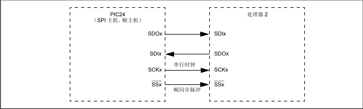
图 14-4: SPI 主机、帧主机连接图
