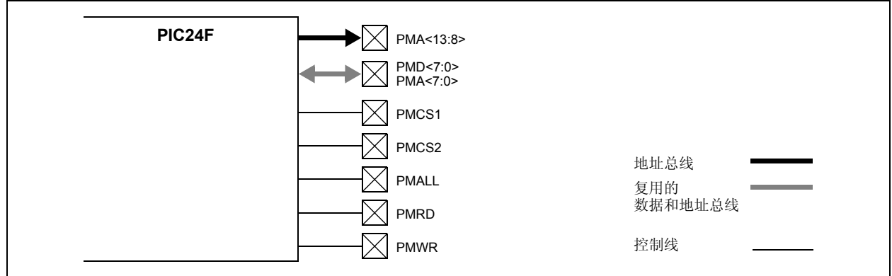
图 17-5: 主控模式下的部分复用寻址（单独的读和写选通、两个片选信号）
