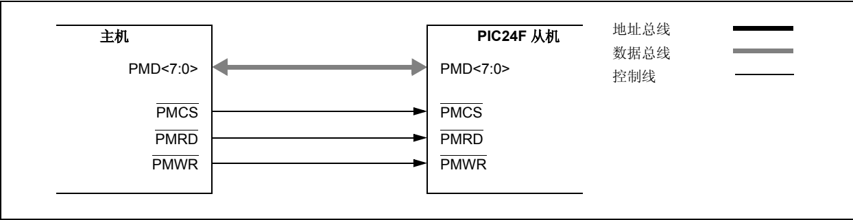
图 17-2: 传统并行从动端口示例
