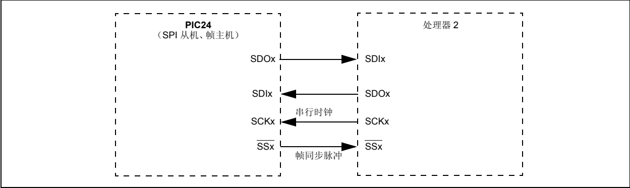
图 14-6: SPI 从机、帧主机连接图
