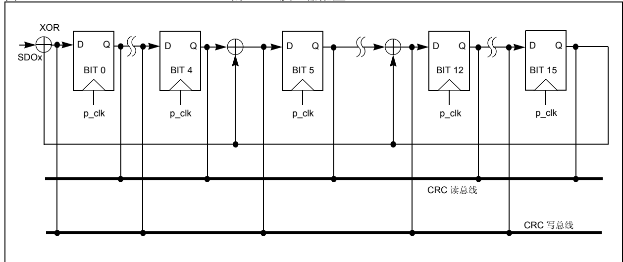
图 19-2: x^{16} + x^{12} + x^5 + 1 的 CRC 发生器配置
