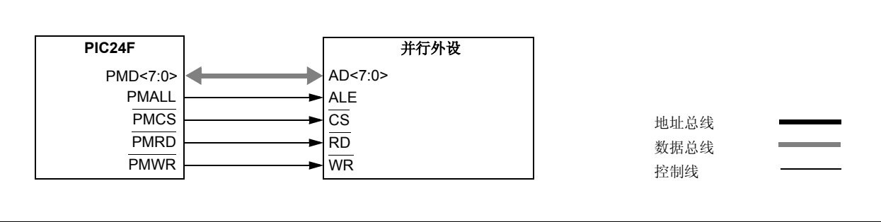
图 17-9: 8 位地址和数据复用的应用示例
