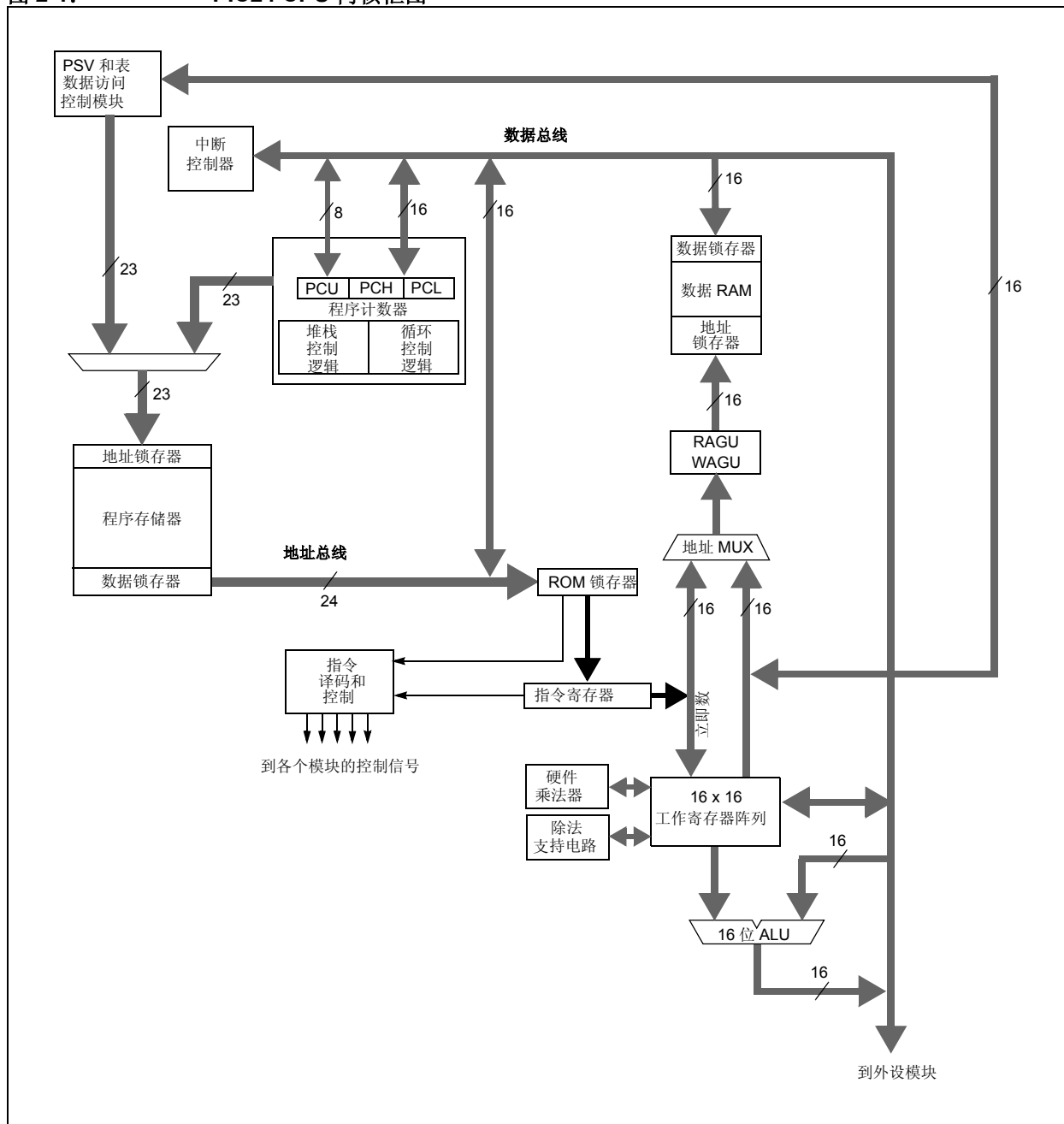
图 2-1: PIC24 CPU 内核框图
