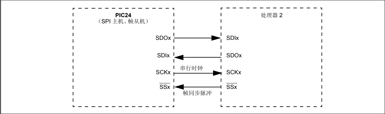
图 14-5: SPI 主机、帧从机连接图
