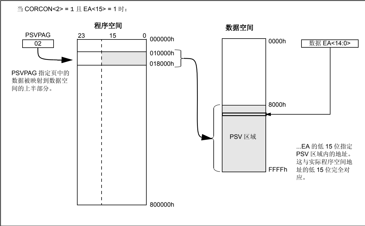
图 3-7: 程序空间可视化操作
