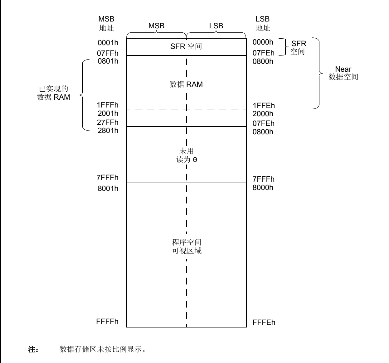
图 3-3: PIC24FJ128GA 系列器件的数据空间存储器映射
