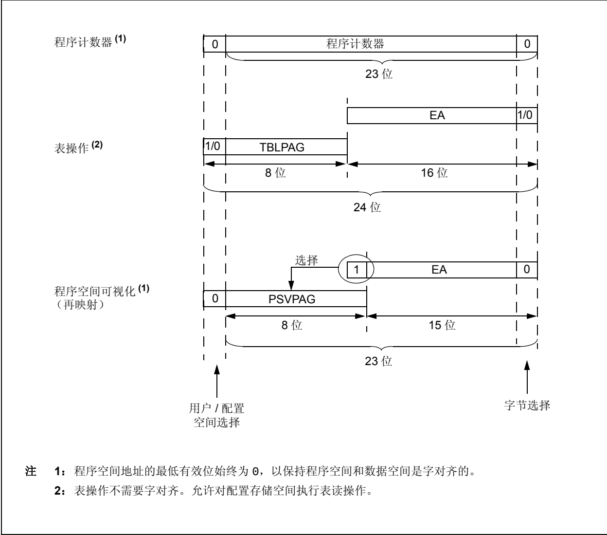
图 3-5: 用程序空间生成地址访问数据
