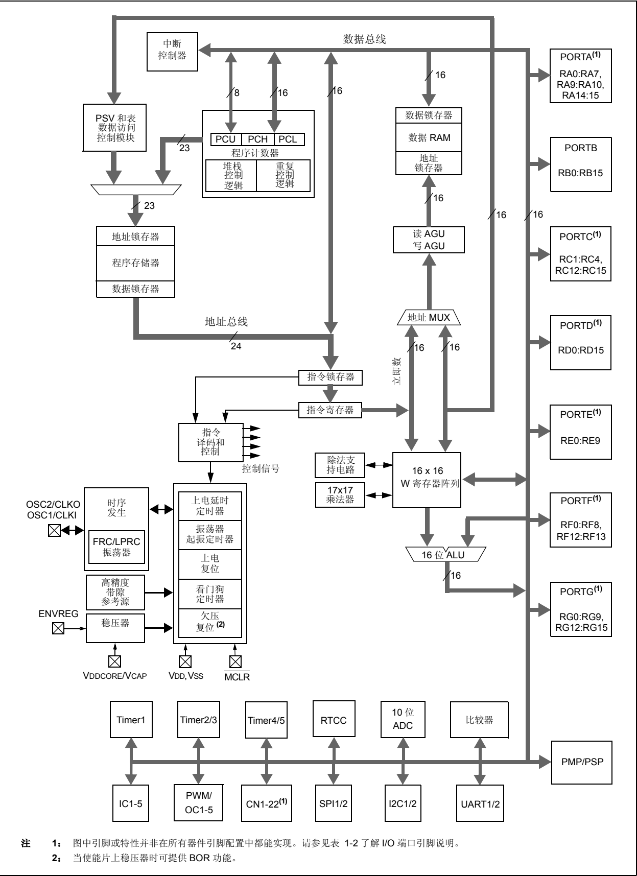
图 1-1: PIC24FJ128GA 系列的通用框图
