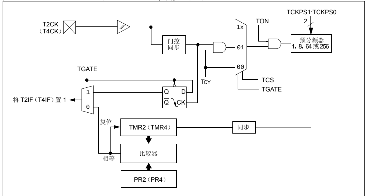
图 11-2: TIMER2 和 TIMER4 (16 位同步) 框图
