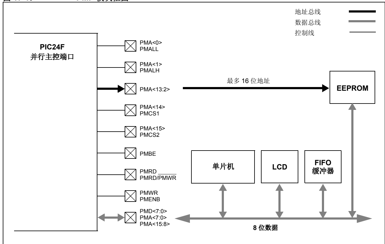
图 17-1: PMP 模块框图
