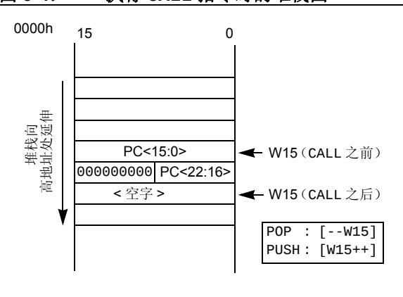
图 3-4： 执行 CALL 指令时的堆栈图
