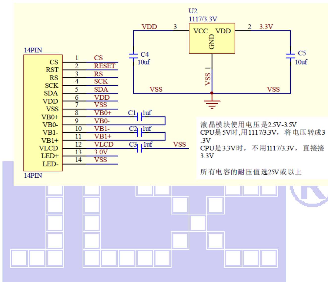
图 4. 串行接口
