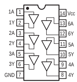
TC74HCT7007AF (AU:IC823)
