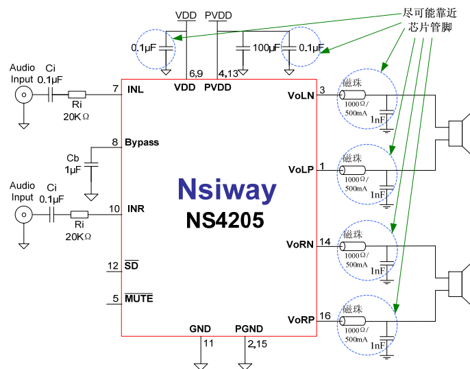
图5 NS4205 加磁珠应用电路
