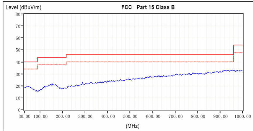
图4 EMI测试频谱图
