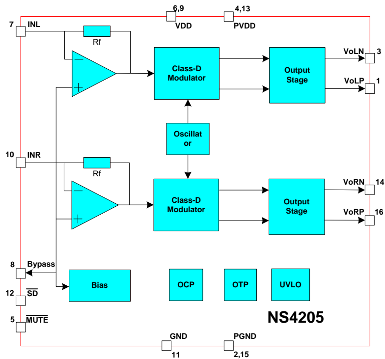
图3 NS4205 原理框图
