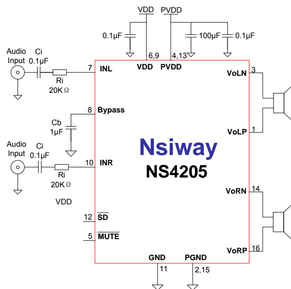
图1 NS4205 典型应用电路
