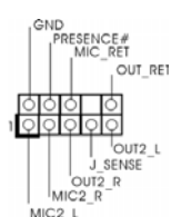
フロントオーディオパネルコネクタ (9ピン HD_AUDIO1) ページ2 , アイテム 36 を参照
