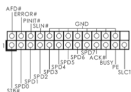
印表機接針 (25 針 LPT1) (見第 2 頁第 29 項)
