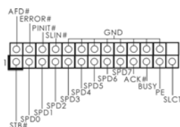
プリントポートヘッダ (25ピン LPT1) ページ2 , アイテム 29 を参照
