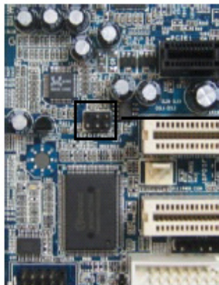
A. 5Pin JSPDIF header
