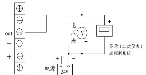
三线电压输出接线图 (JYB-KG-PV***)
