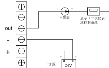
二线制电流输出接线图(JYB-KG-PA***)
