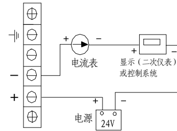
二线制电流输出接线图(JYB-KG-PA***)
