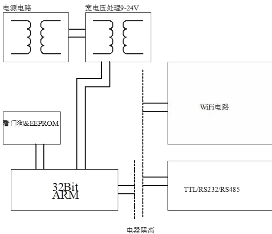
原理框图
