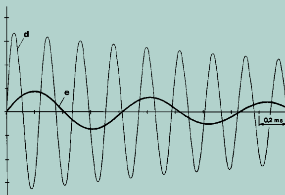
电流中的两个谐波（见上图）
