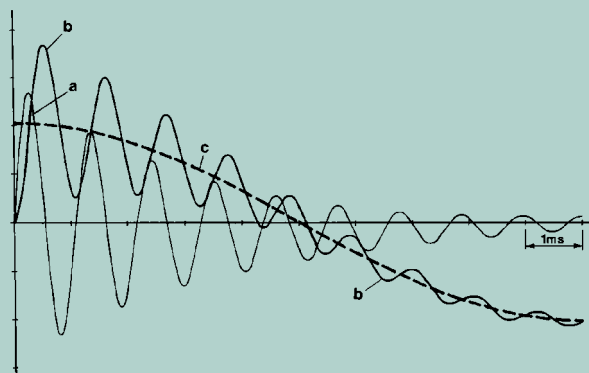
投切后初始 10ms 的电流、电压波形
