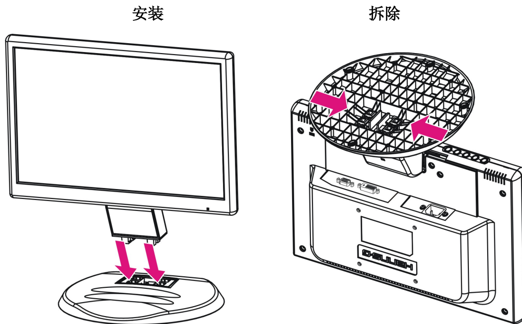
图一. 安装和拆除底座
