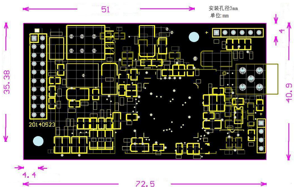
图 1-5: MD-139 裸板尺寸
