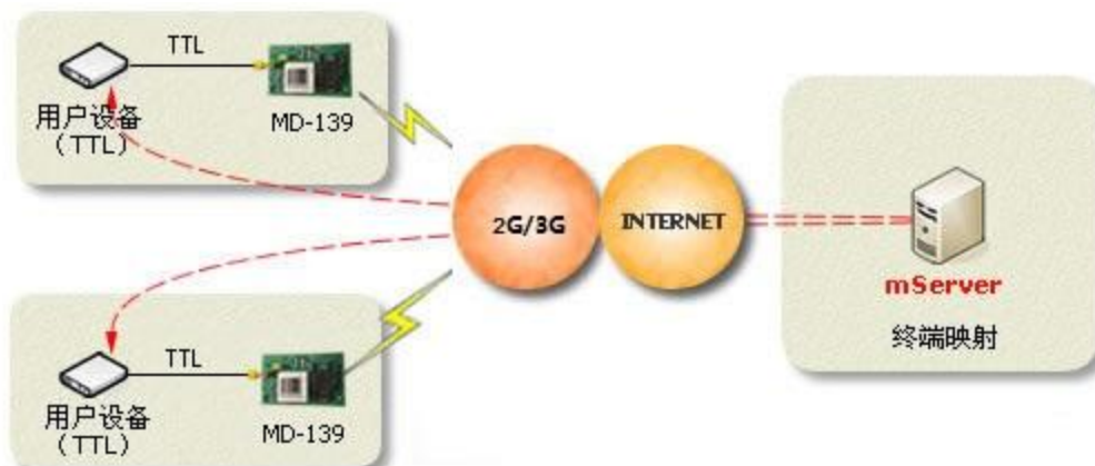
图 1-9: MD-139 通过 mServer 映射实现点到点（串口到串口）
