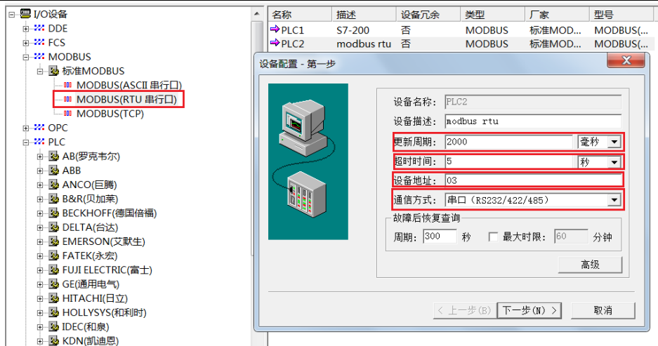
图附 6-9: 创建 MODBUS RTU 设备
