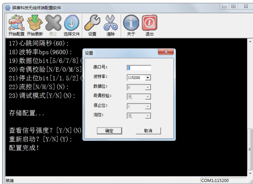
图 2-2: 设置串口号
