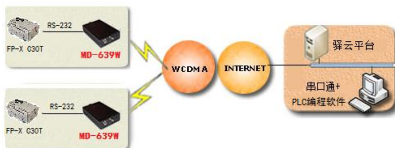
图附 7-1： FP-XC30T 与 MD-639W 连接远程下载程序
