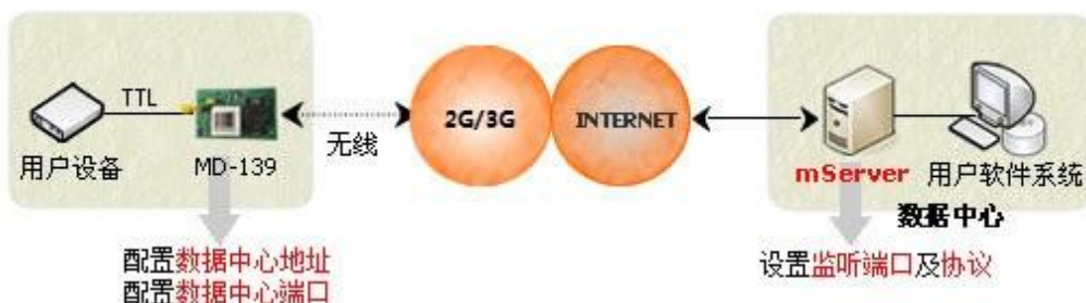
图 1-6: MD-139 工作原理
