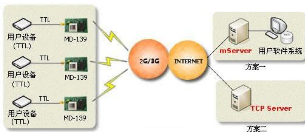
图 1-7: MD-139 多点到中心
