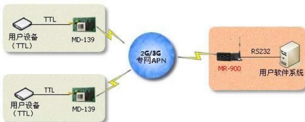
图 1-10: MD-139 嵌入式数据中心实现点到点（串口到串口）
