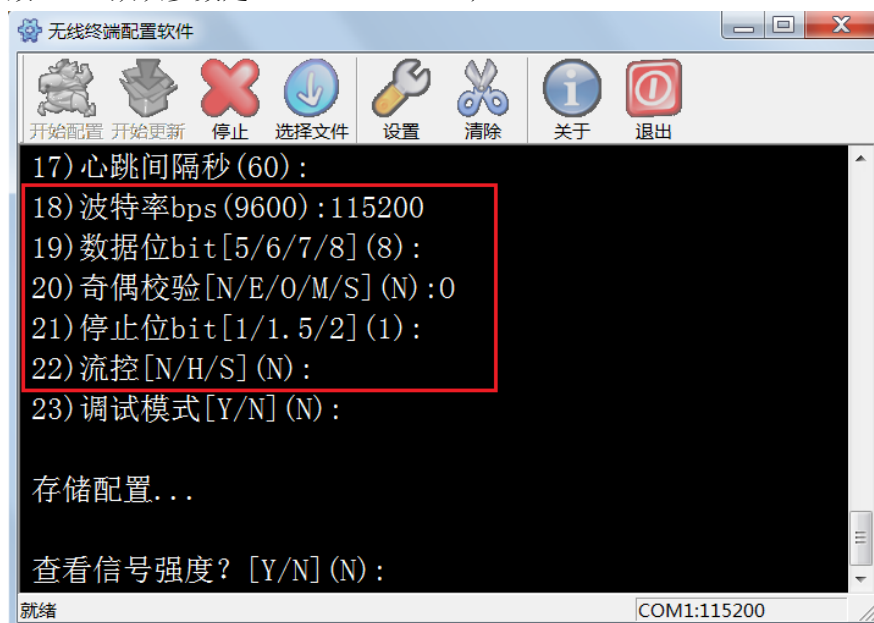
图附 7-2：设置 DTU 串口参数
