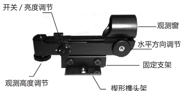
图 3-4 红点寻星镜
