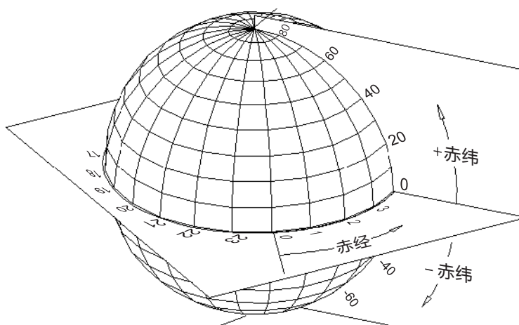
图 6-1 天球示意图
