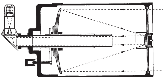
图 5-1 施密特-卡塞格林结构光路图
