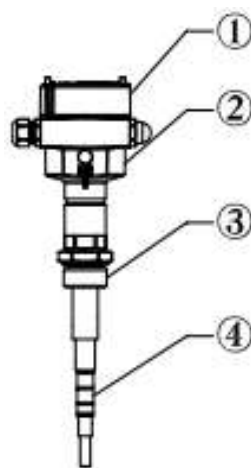
图 1 Cape-11 整体结构图
