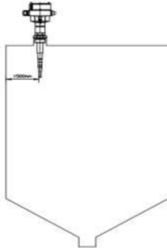
图3 垂直安装示意图
