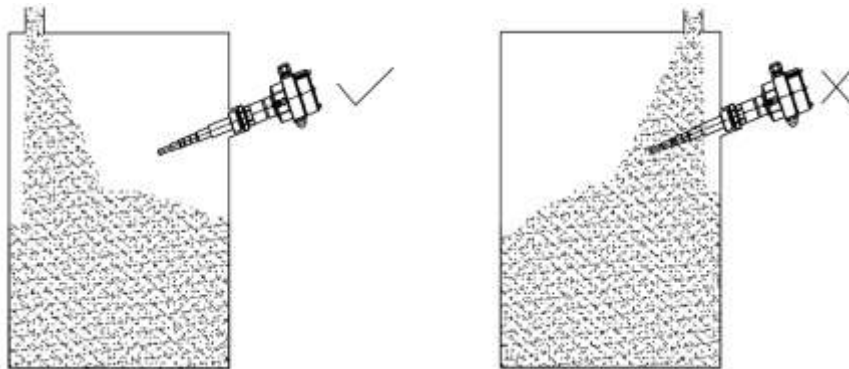
图4 避免入料口的安装示意图
