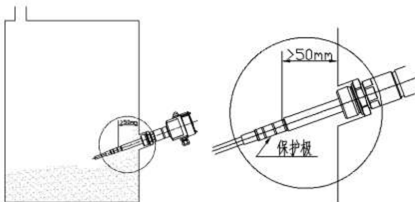
图 6 保护极插入深度
