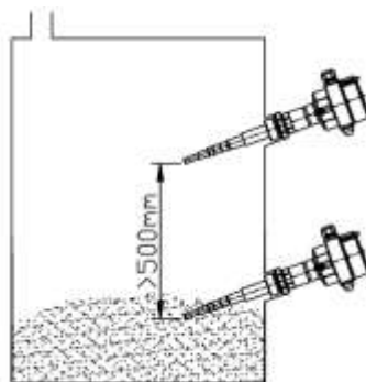
图5 安装间距
