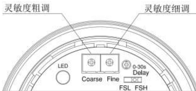
图9 灵敏度调节图
