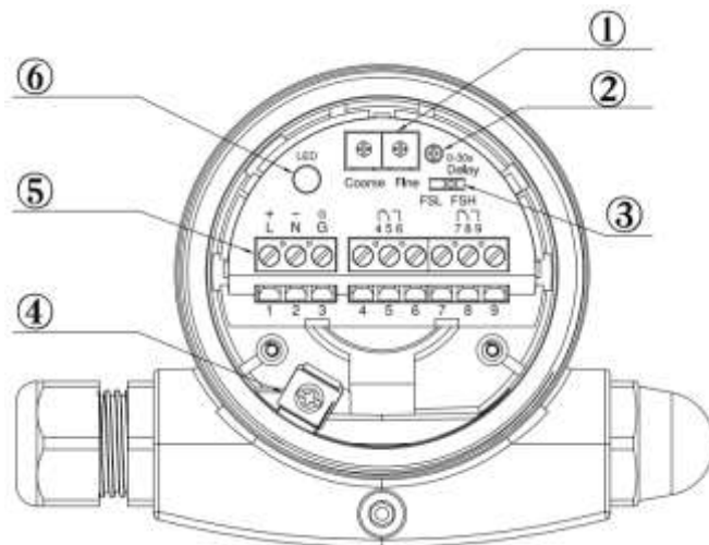
图 8 内部结构图
