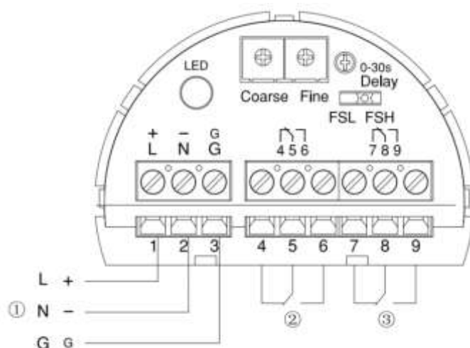
图 7 接线示意图
