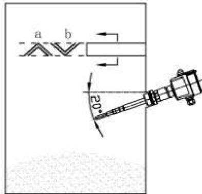
图 2 水平安装示意图
