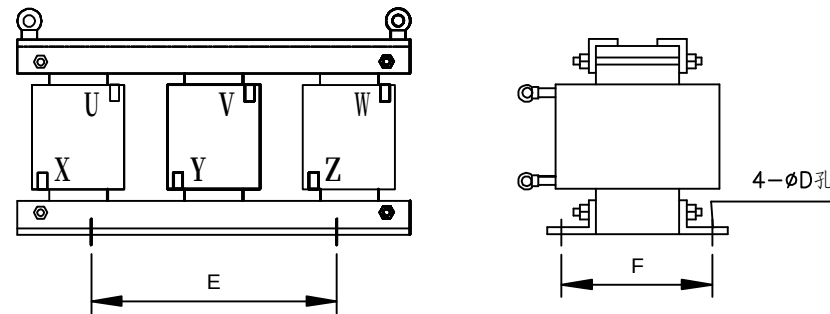
外形尺寸：
