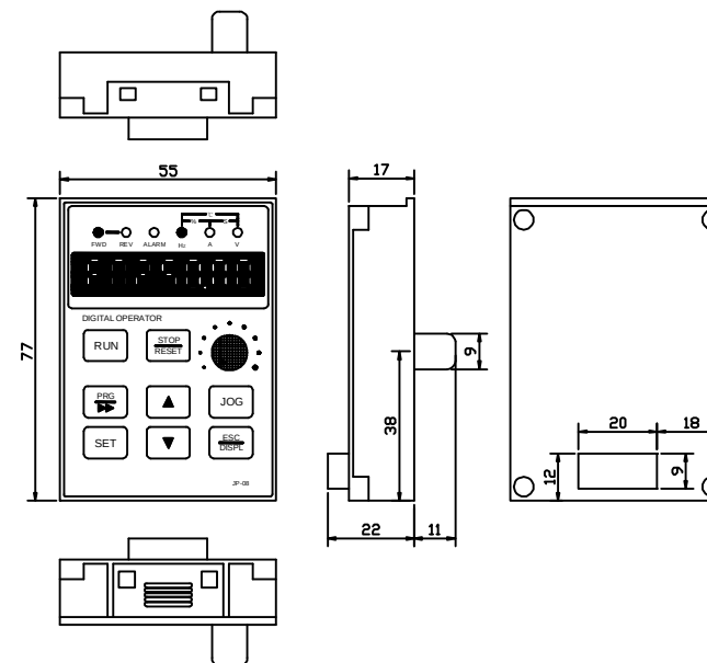
JP5E7000 尺寸图:
