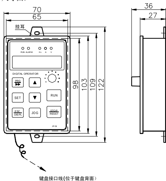
JP3E7000 尺寸图:
