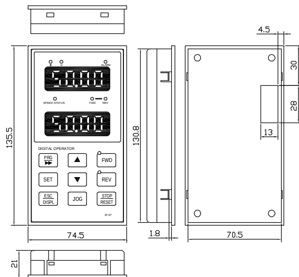
JP6E7000/ JP6C7000 尺寸图:
