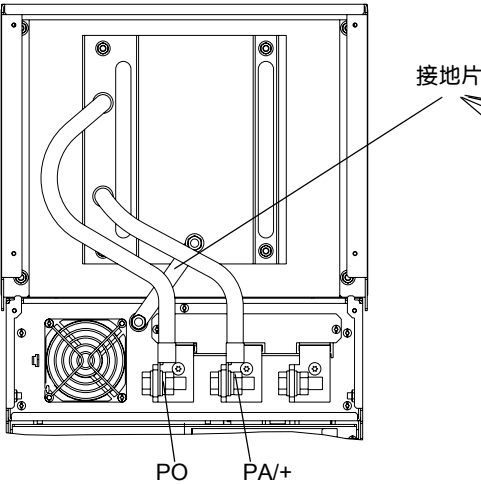
示例 2: ATV71H C16N4 ... C28N4
