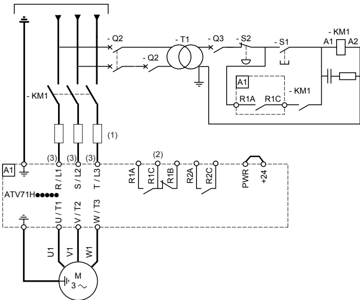
带有线路接触器的连接图
