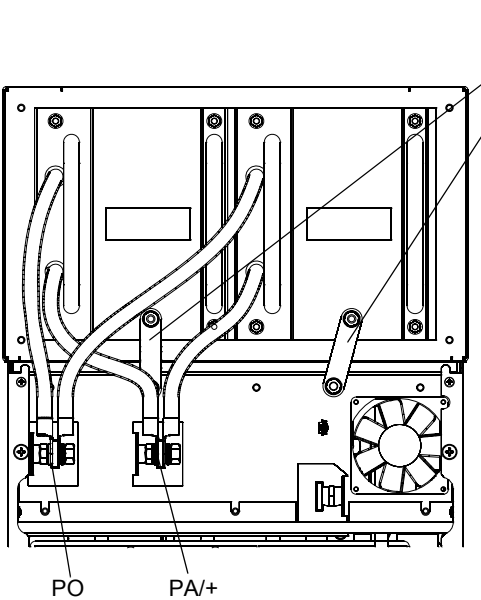
示例 2: ATV71H C16N4 ... C28N4
