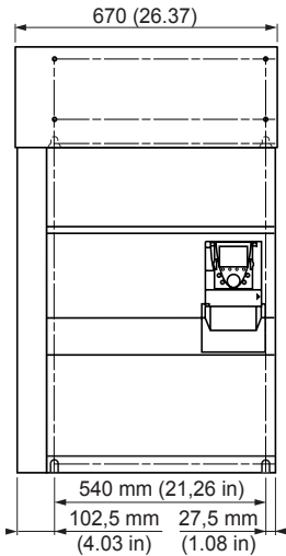
ATV71H C20Y 至 C31Y 带有制动单元
