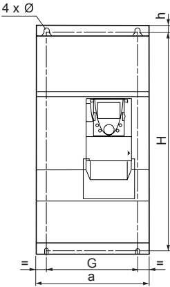
ATV71H D55M3XD, D75M3XD ATV71H D90N4D 至 C28N4D
