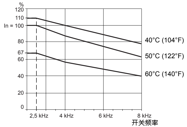
ATV71HD90N4
