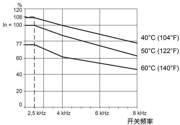
ATV71HC25N4
