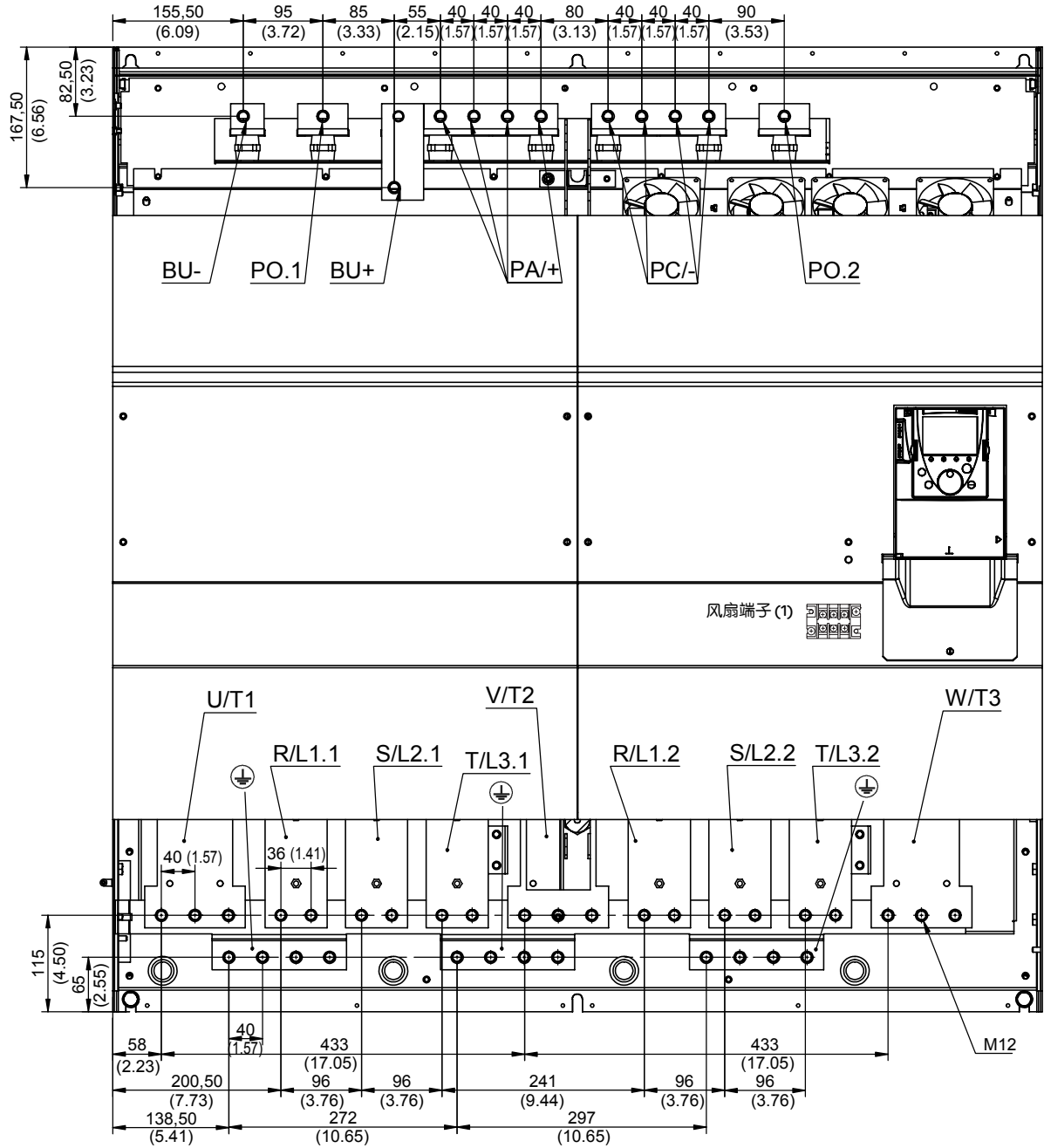
正视图
