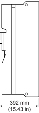
带 2 个可选卡 (1)
