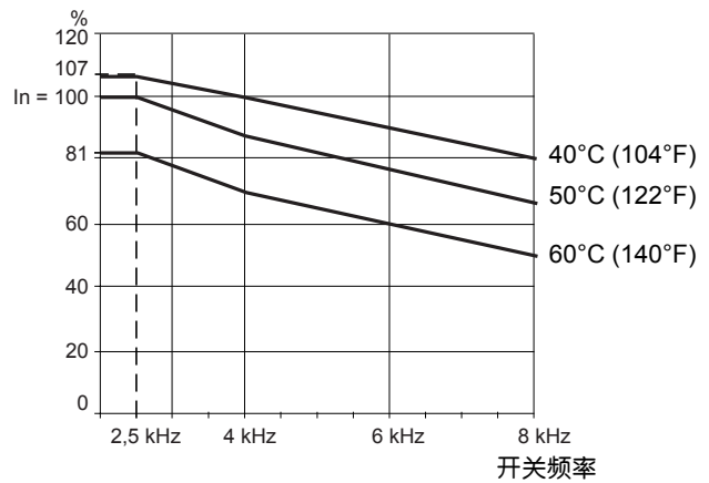
ATV71HC28N4
