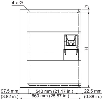
ATV71H C20N4D 至 C28N4D 带有制动单元 (VW3A7101)
