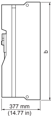
无可选卡或带 1 个可选卡 (1)
