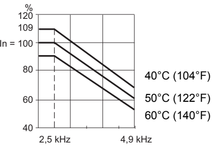
ATV71HC63Y
