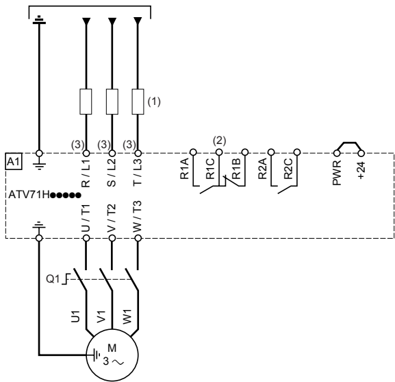
带有负荷开关的连接图
