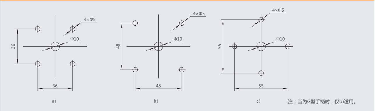
图3 NKZ1系列安装开孔尺寸
