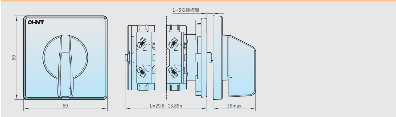
图1 NKZ1系列R型手柄产品外形尺寸
