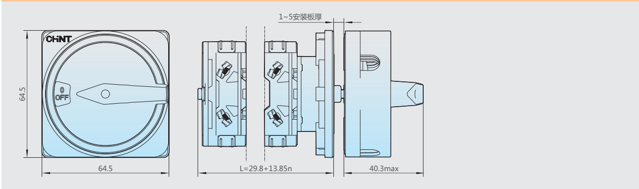
图2 NKZ1系列G型手柄产品外形尺寸
