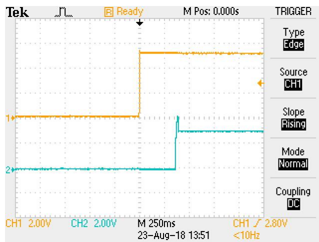
ESM7000 主板上电时 RESET_IN_OUTn 时序 (CH1: 5V 电源, CH2: RESET_IN_OUTn 信号)
