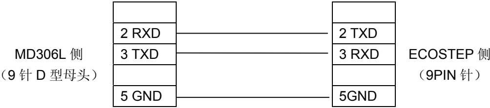
MD-ECOSTEP-CAB485 连线图
