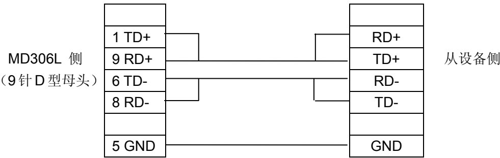
MD2-MODBUS-RS422 连线图
