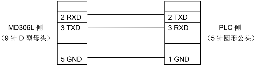
MD2-FP 电缆连线图
