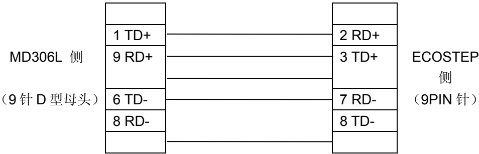
MD-ECOSTEP-CAB422 连线图
