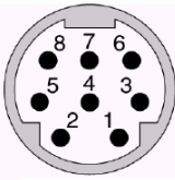
8 针圆形母座管脚图
