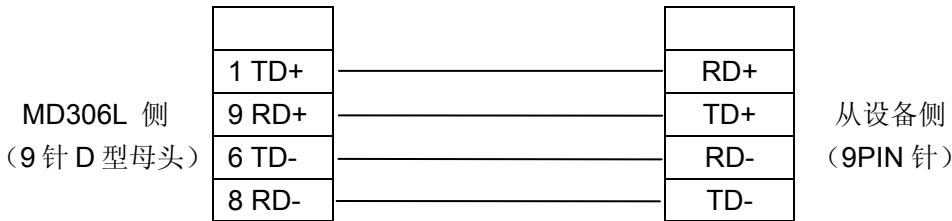
MD2-MODBUS-RS422 连线图
