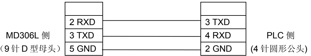
MD2-FACON FBS 系列电缆连线图
