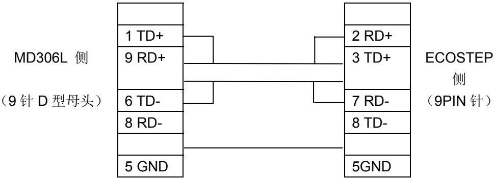
MD-ECOSTEP-CAB422 连线图
