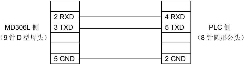
MD2-AB 电缆连线图
