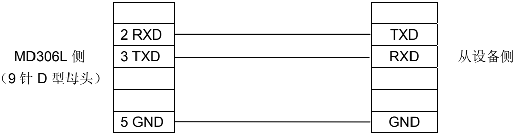
MD2-MODBUS-RS232 连线图
