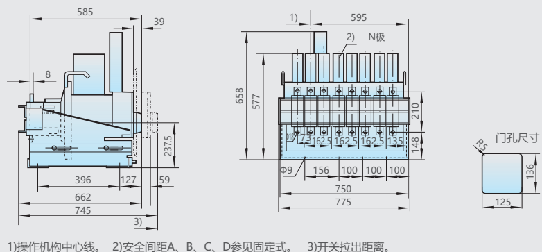
图16-7 DW17D-2900/4(In=2000A、2500A)四极抽屉式接线
