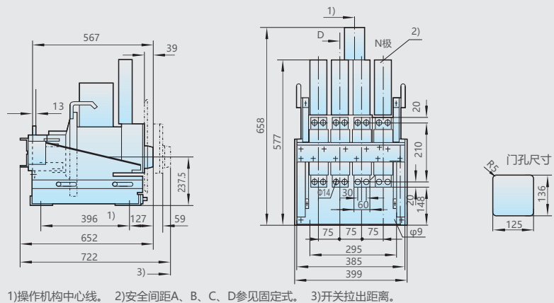
图16-7 DW17D-2900/4(In=2000A、2500A)四极抽屉式接线
