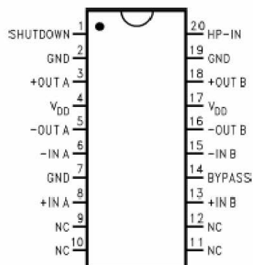
TSSOP20封装
