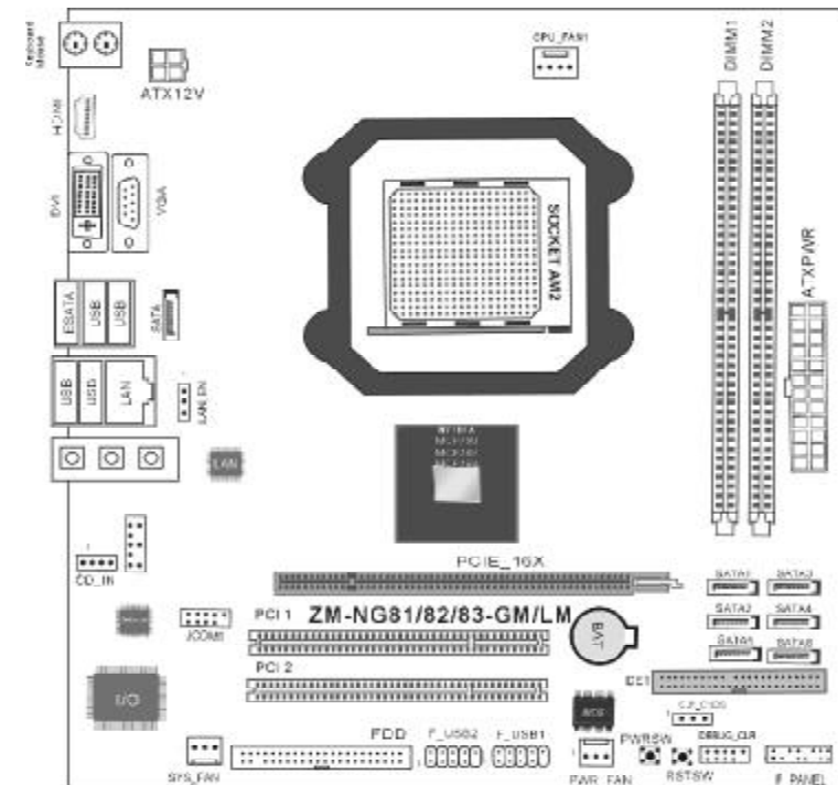
ZM-NG81/NG82/NG83-GM (LM) 主机板布局图
