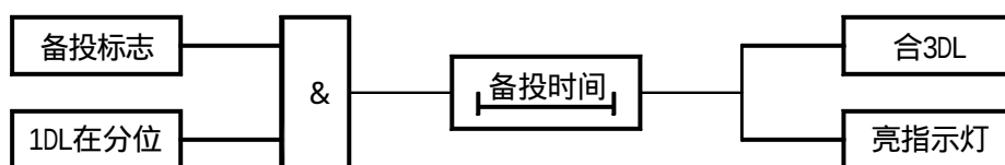
图 3.5 分段开关自投 1 的备投逻辑
