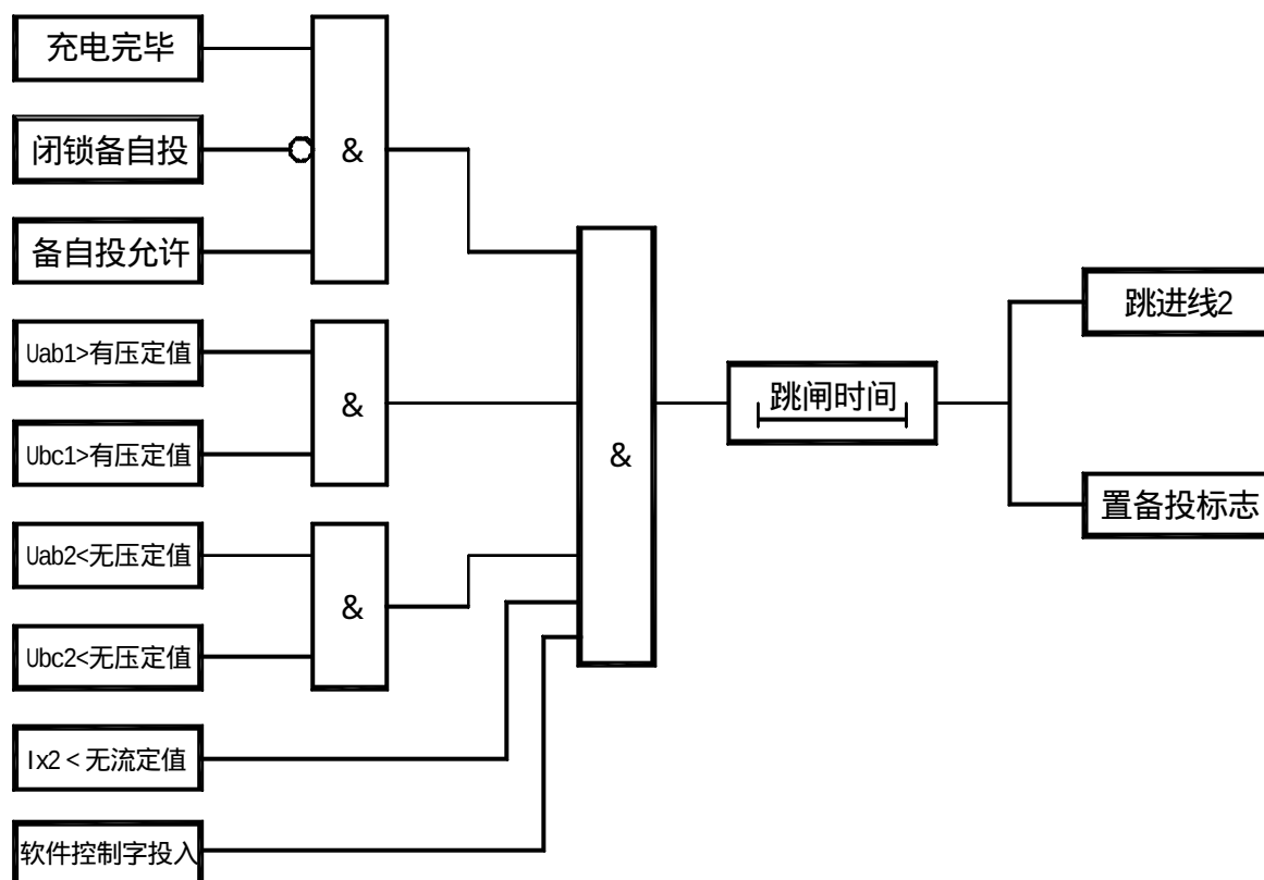
图 3.6 分段开关自投 2 的跳闸逻辑
