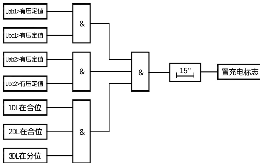
图 3.2 分段开关自投的充电逻辑
