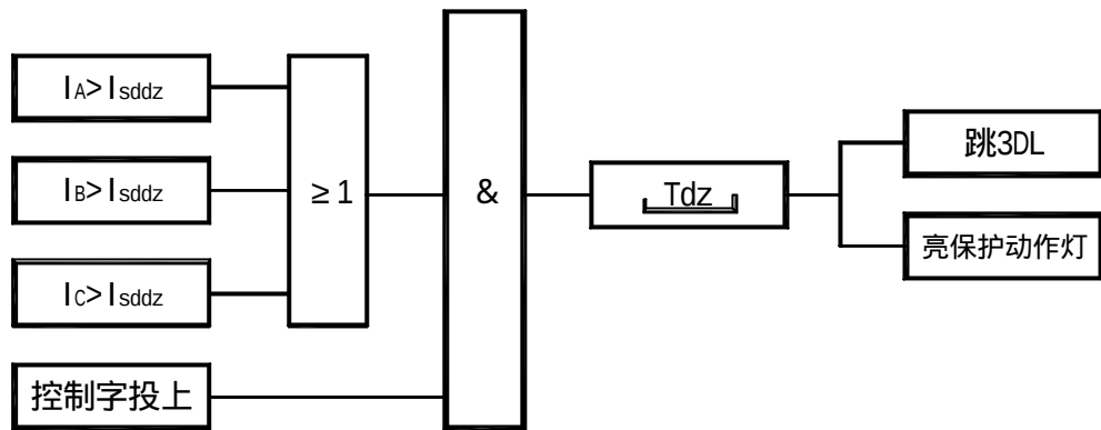
图 3.8 限时速断动作逻辑图
