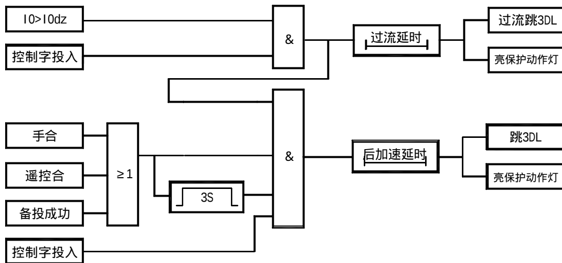
图 3.10 定时限零序过电流保护及后加速保护动作逻辑图
