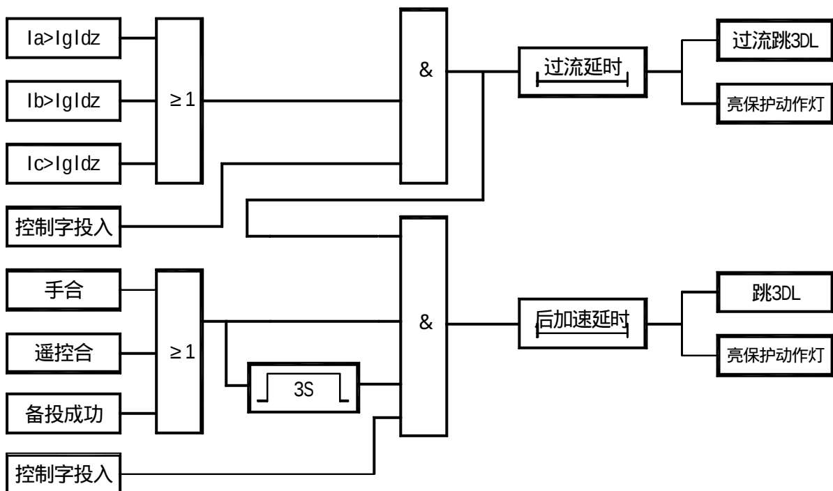
图 3.9 定时限过电流保护及后加速保护动作逻辑图
