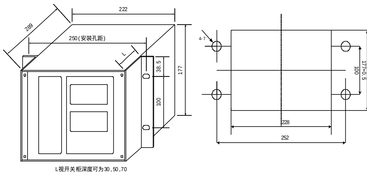
机箱外形尺寸及安装开孔尺寸（二）
