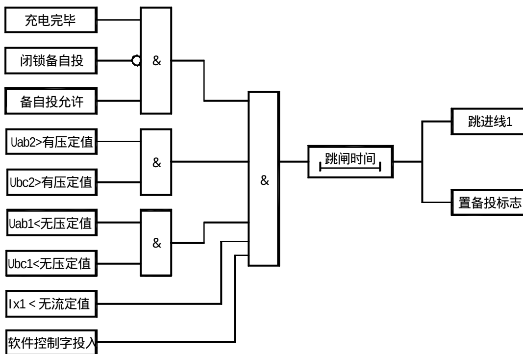
图 3.3 分段开关自投的慢速放电逻辑图
