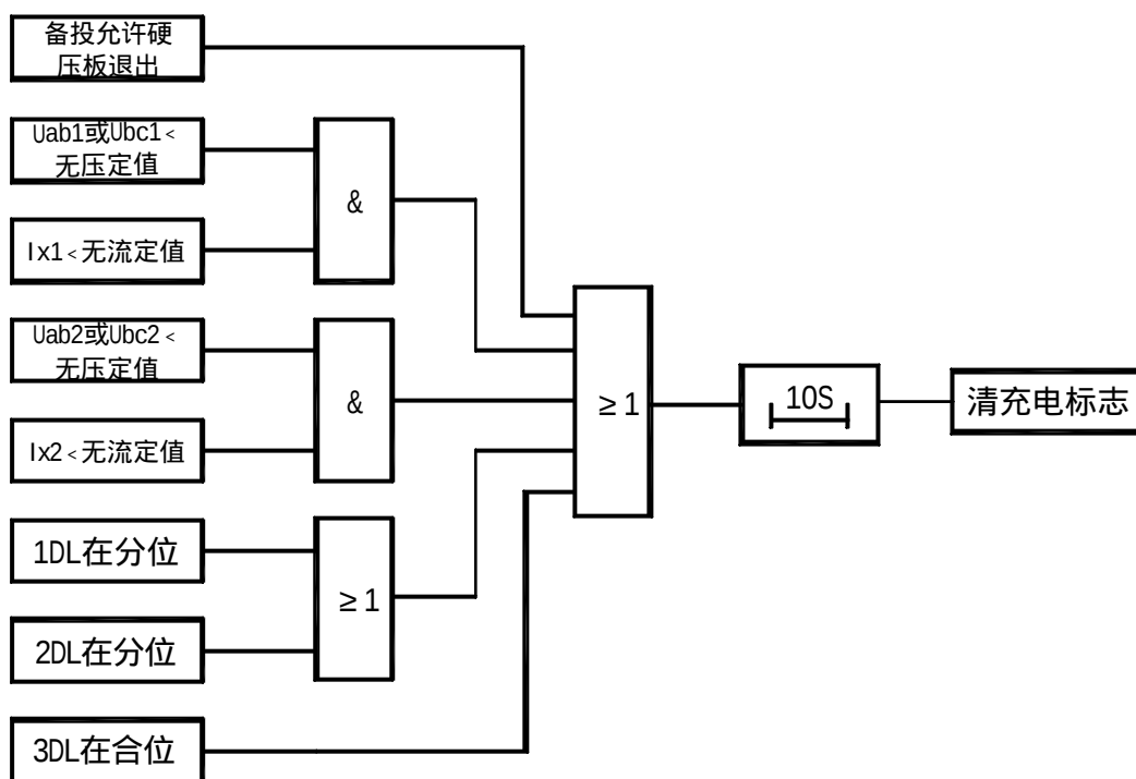
图 3.4 分段开关自投 1 的跳闸逻辑
