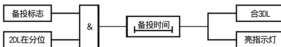
图 3.7 分段开关自投 2 的备投逻辑
