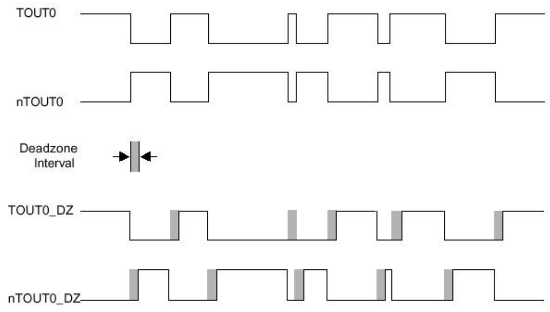
图 9 - 7 当死区使能时的输出波形图
