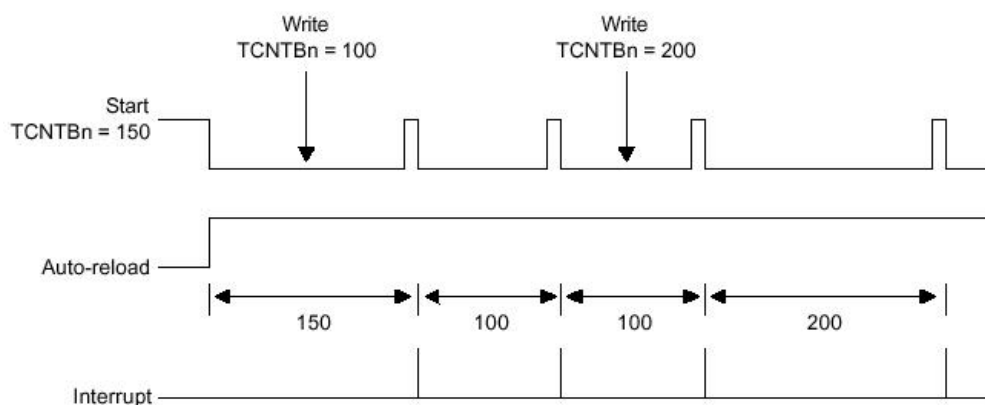
图 9-3 双缓冲器定时效果示例图
