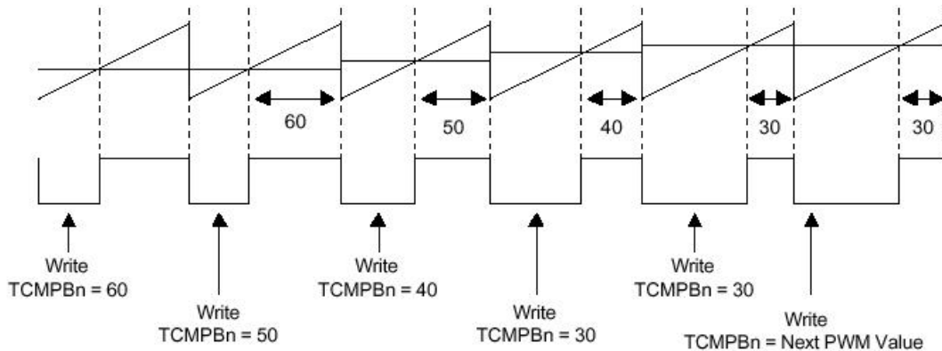
图 9—5 PWM 的实例图
