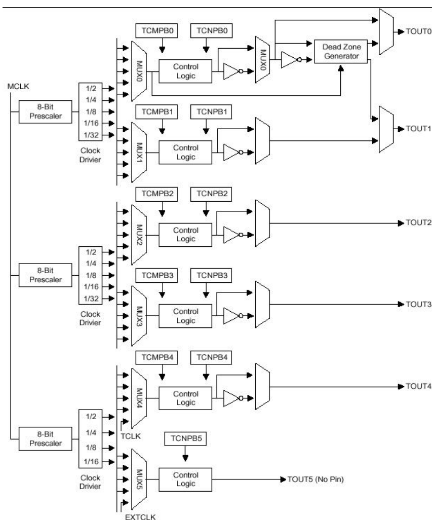
图 9-1 定时器内部结构图
