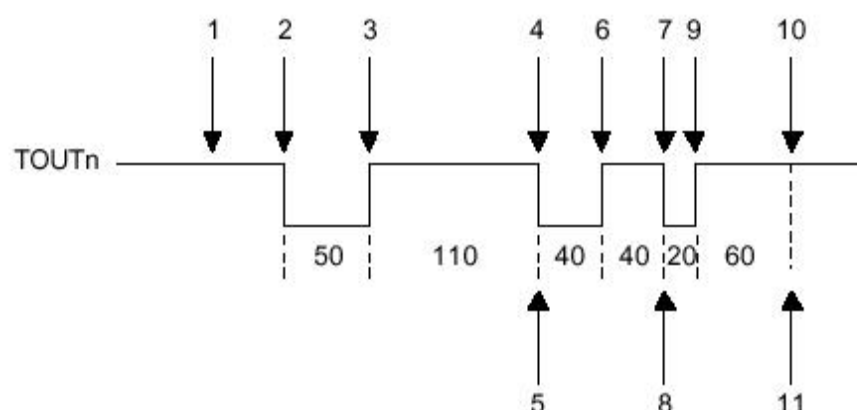
图 9-4 定时器操作的例子
