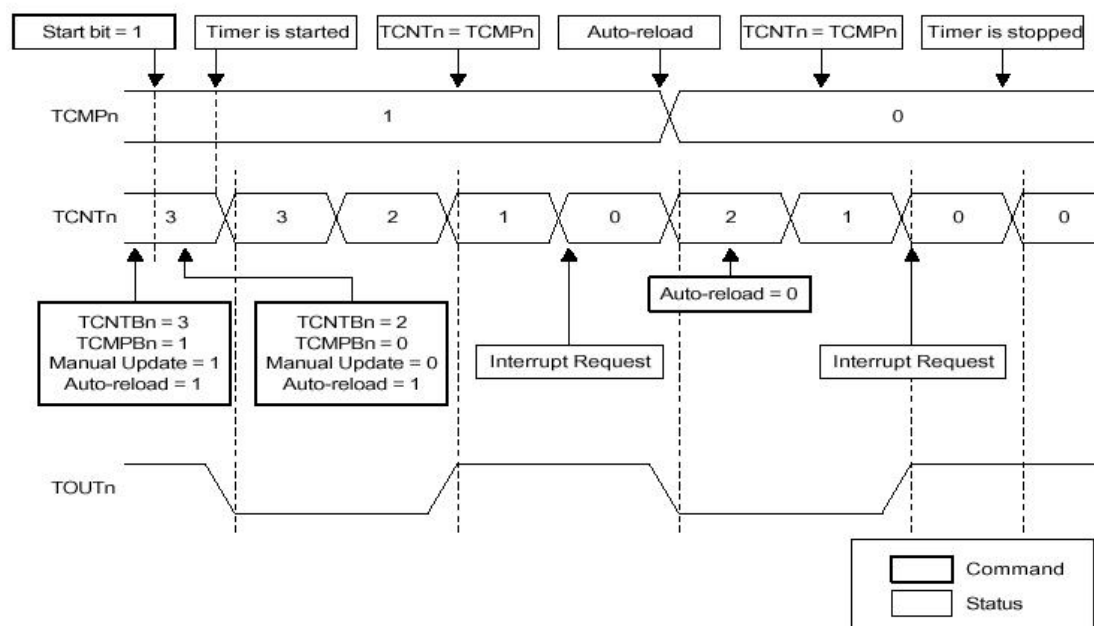
图 9-2 定时器操作
