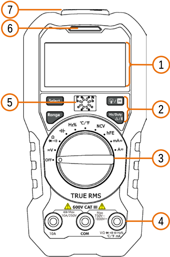
图 2-1 前面板概览（以 OW16B 为例）
