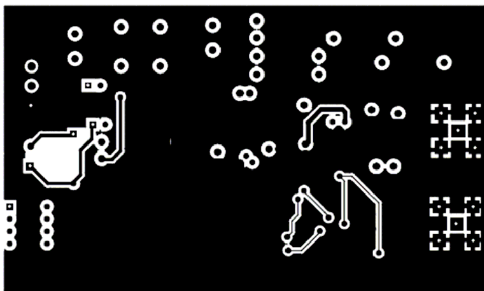
Bottom LAYER
