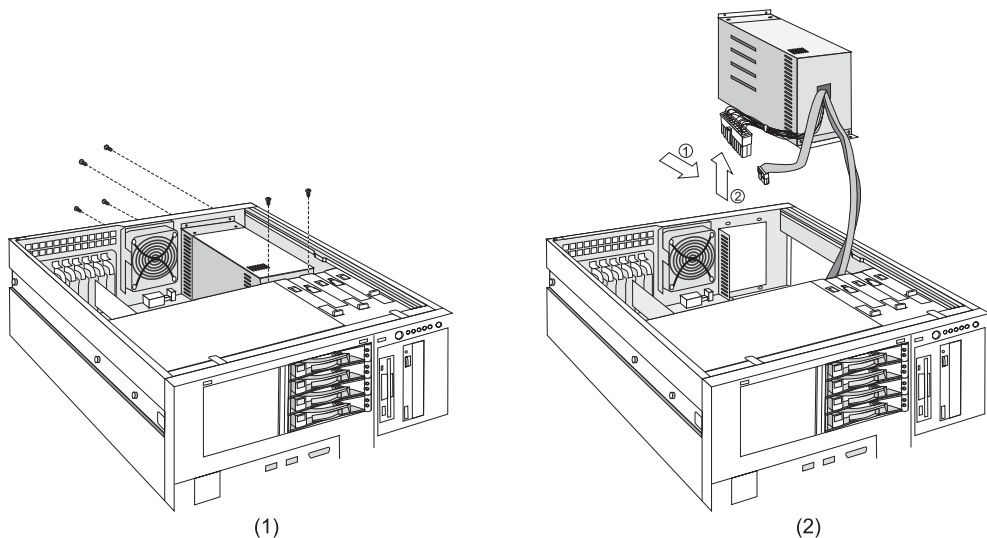
电源的拆装
