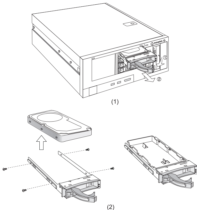
硬盘的拆装
