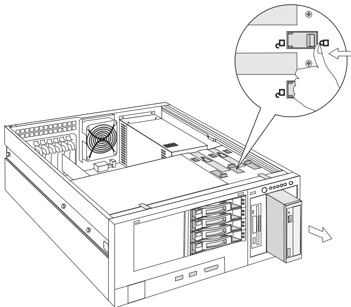
光驱的拆装
