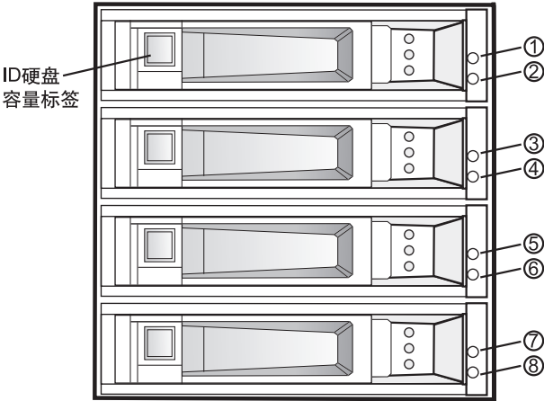
模组前面板示意图
