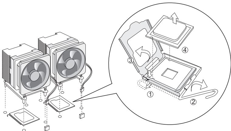
CPU 及散热器的拆装
