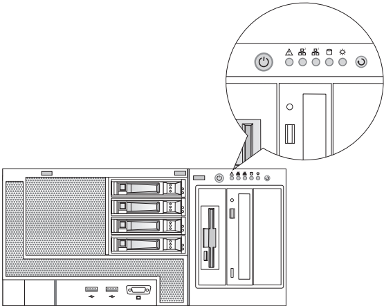
前面板示意图（RACK）
