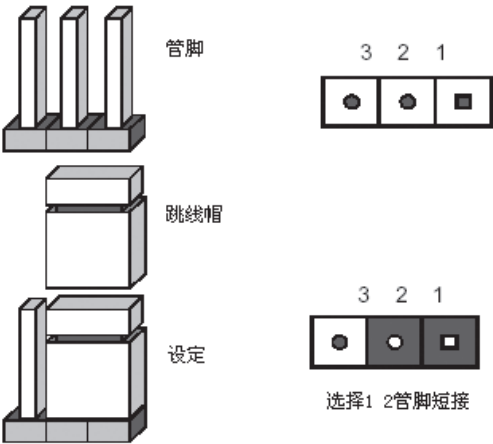
跳线设置示意图
