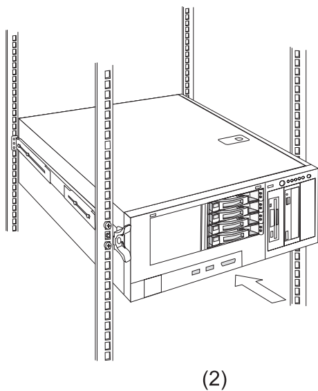
服务器上机架安装
