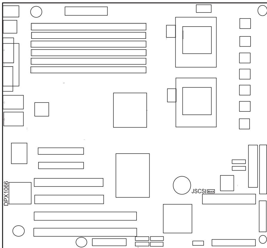
启用 / 禁用板载 SCSI 跳线位置示意图
