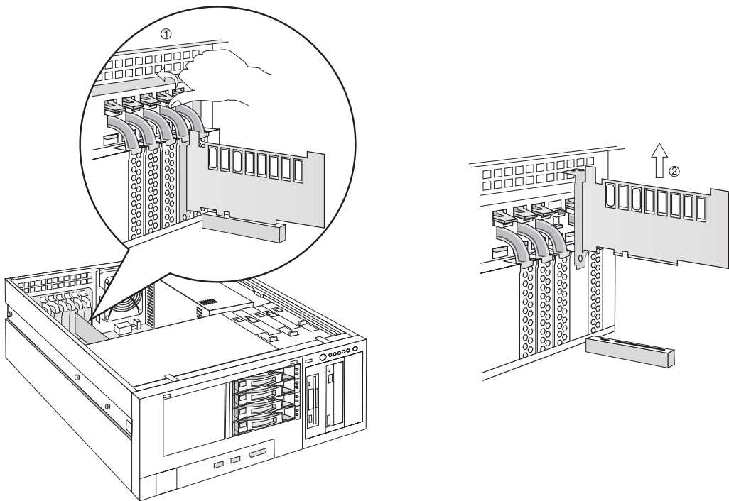
外插卡的拆装
