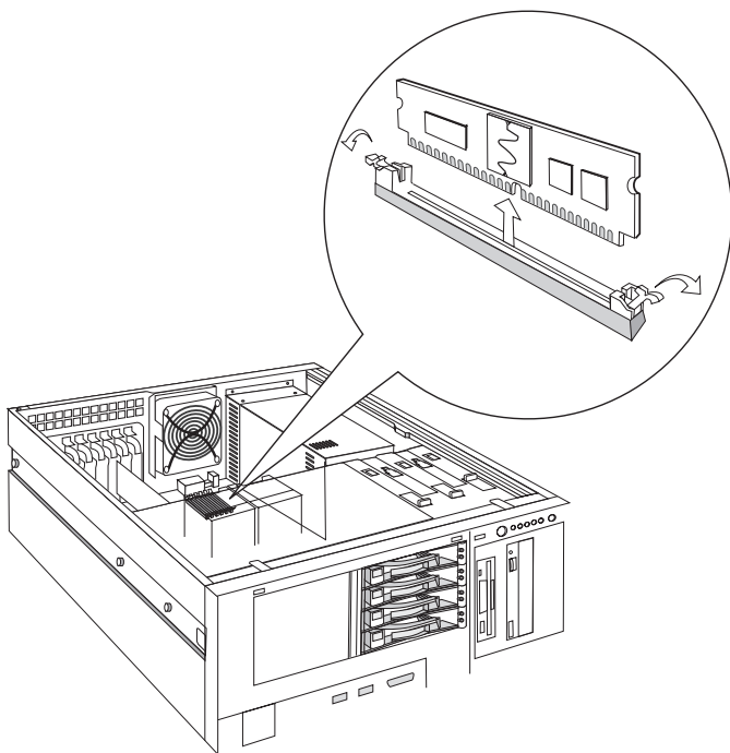
内存的拆装
