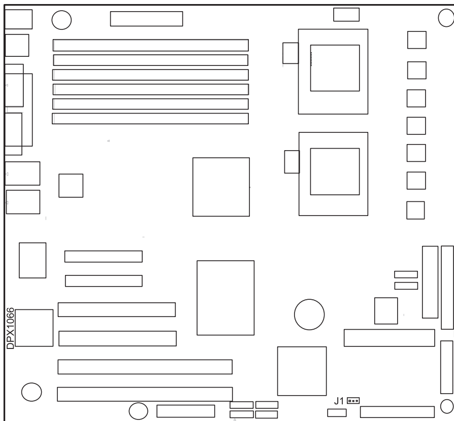
模组终结器设置跳线位置示意图
