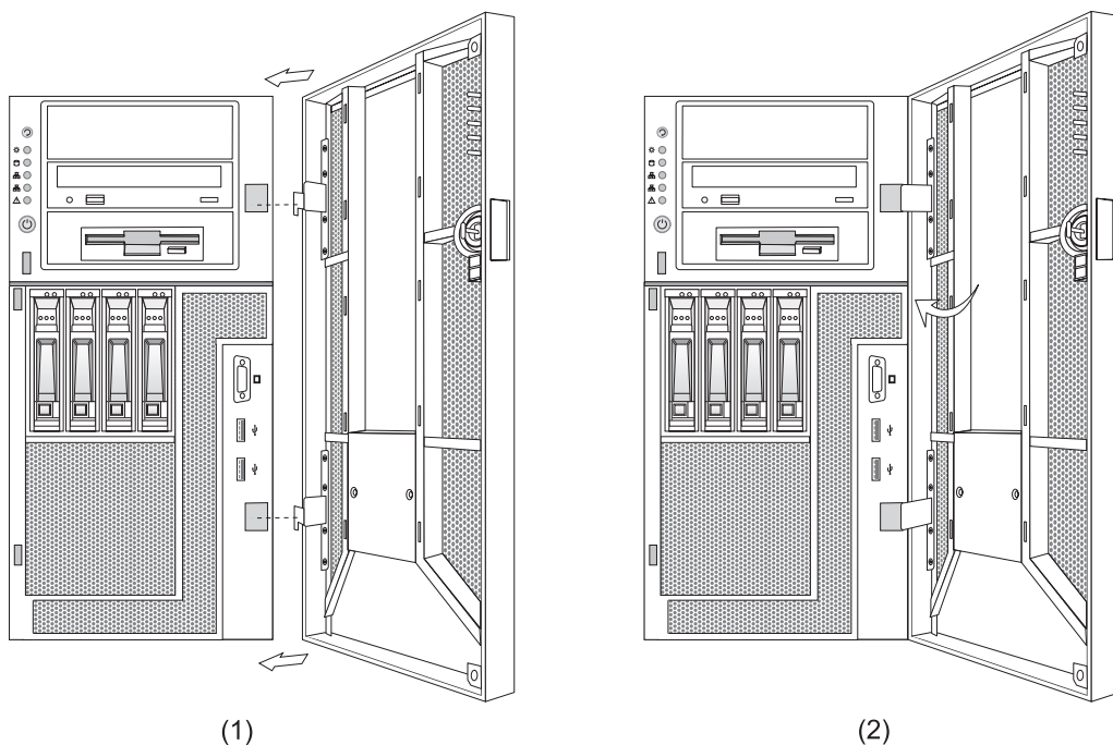
T350 G6B 机箱外面板的拆装
