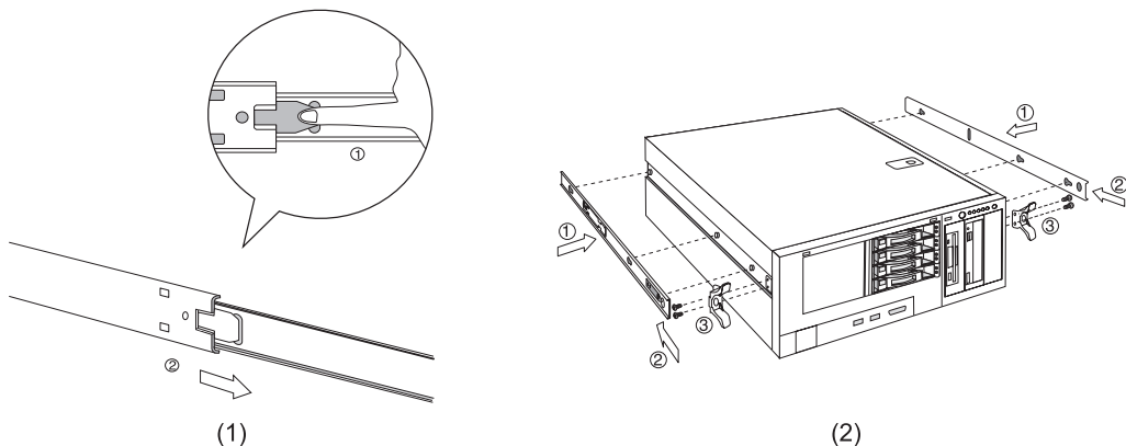
内导轨的拆装
