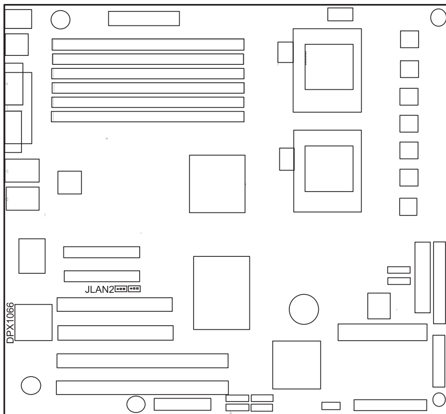
启用 / 禁用板载 LAN 跳线位置示意图
