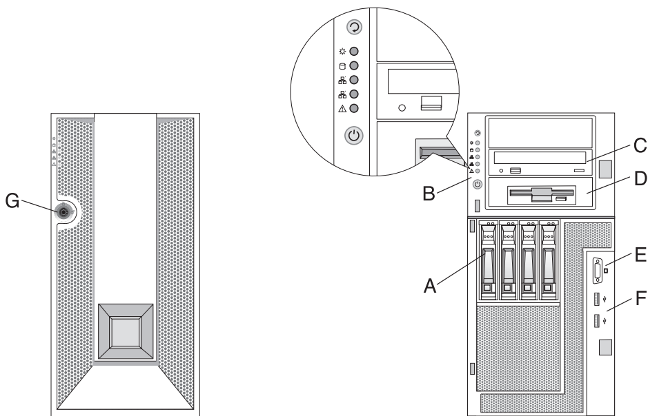
前面板示意图（塔式）
