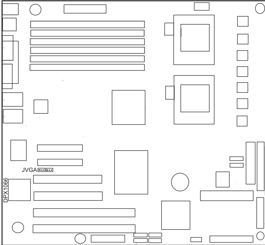
启用 / 禁用板载 VGA 跳线位置示意图
