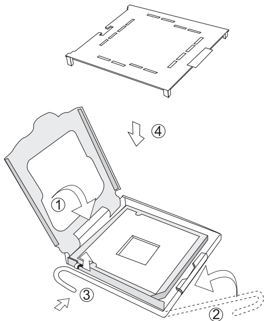
CPU 座保护盖安装
