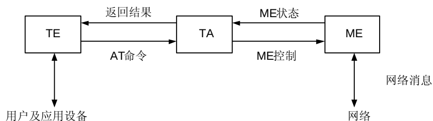
图1-1 系统结构图
