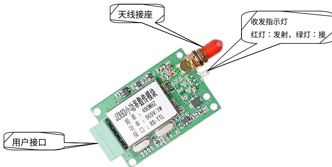
JZ893 接口示意图
