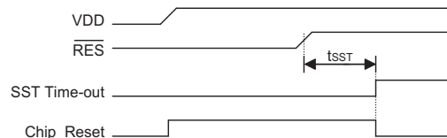
复位时序
