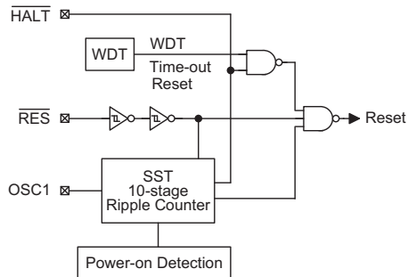
复位电路结构
