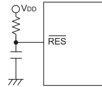
复位电路
