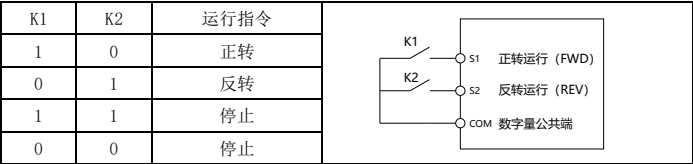
图 6-8 两线式模式 1
