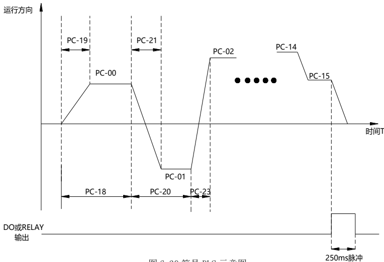
图 6-30 简易 PLC 示意图
