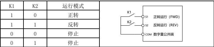
图 6-9 两线式模式 2
